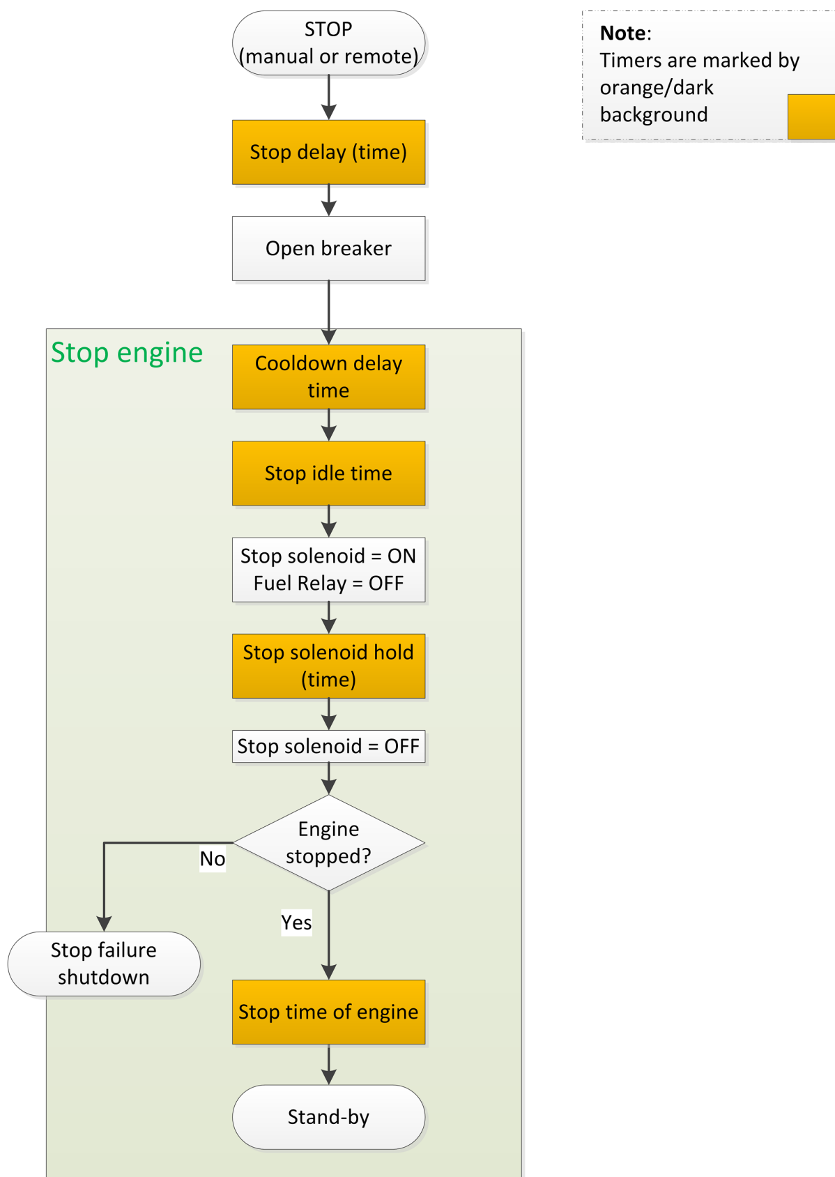
Fig. 4: Procedura arresto/stand-by del motore
