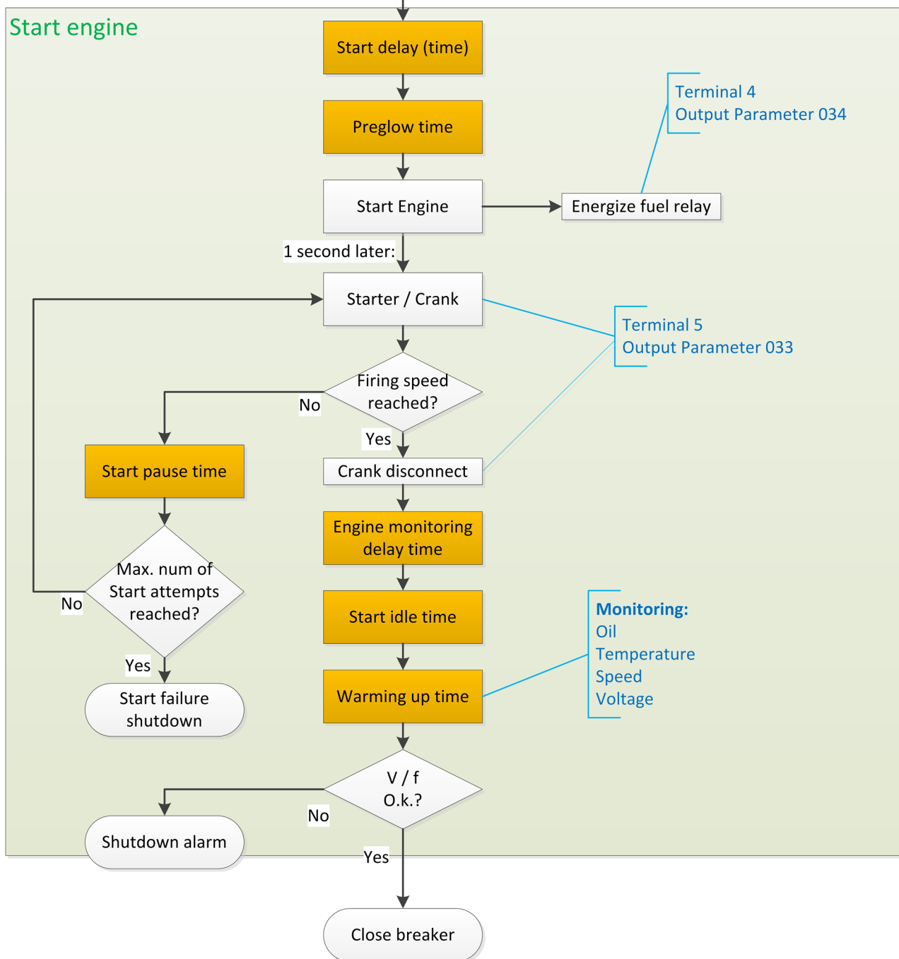
Fig. 3: Procedura di avvio del motore
