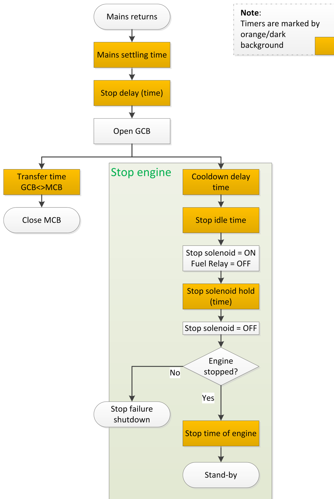
Rys. 4: Przekazywanie agregatu prądowórczego do sieci obejmujące procedurę zatrzymania silnika/przejęcia w stan gotowości
