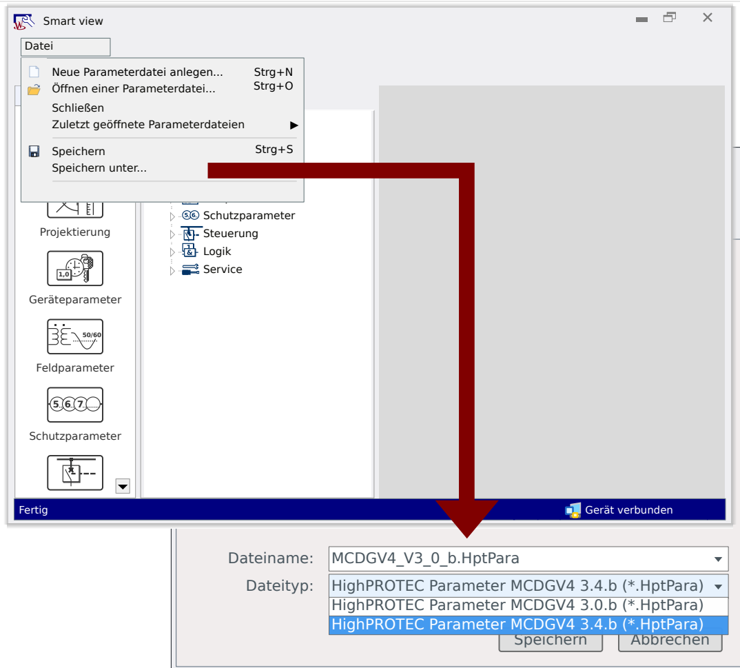
Abb. 6: Eine Konfigurationsdatei für ein MCDGV4 wird von Version „3.0.b“ nach „3.4.b“ konvertiert.
