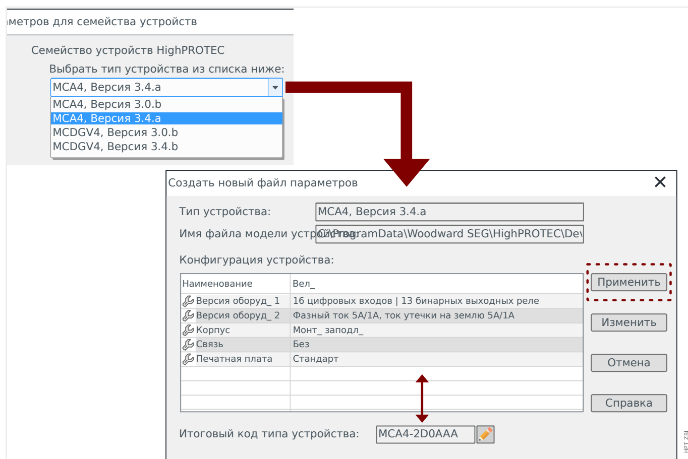
Рис. 4: Для автономного создания файла конфигурации сначала необходимо указать имя и версию устройства. Затем необходимо указать конкретный вариант устройства.
