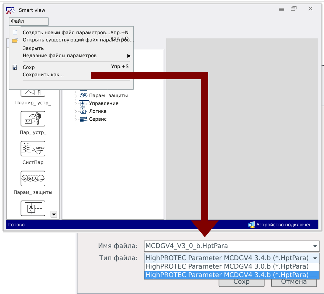
Рис. 6: Преобразование файла конфигурации для MCDGV4 с версии «3.0.b» на версию «3.4.b».
