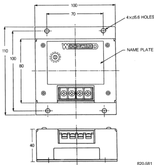
外形図 (工事に使用してはならない。)
