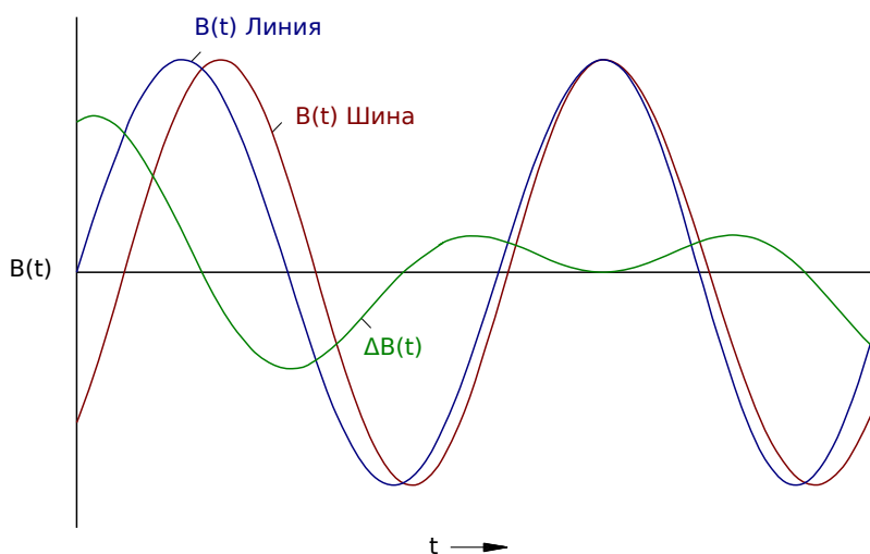
Рис. 110: Кривая напряжения с увеличенным разрешением.
