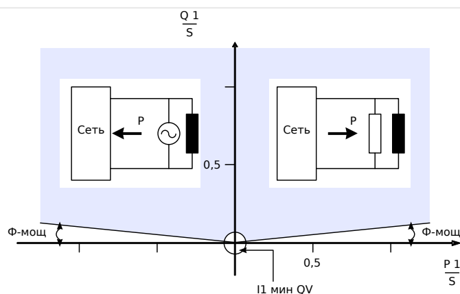
Рис. 91: Метод 1: контроль угла мощности.
