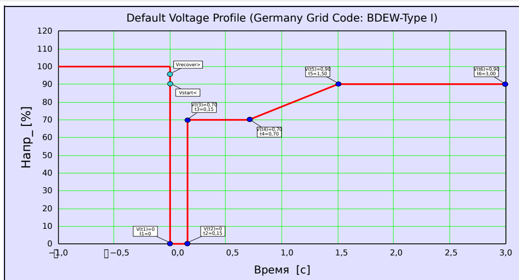
Рис. 80: Профиль LVRT по умолчанию (BDEW, тип I).
