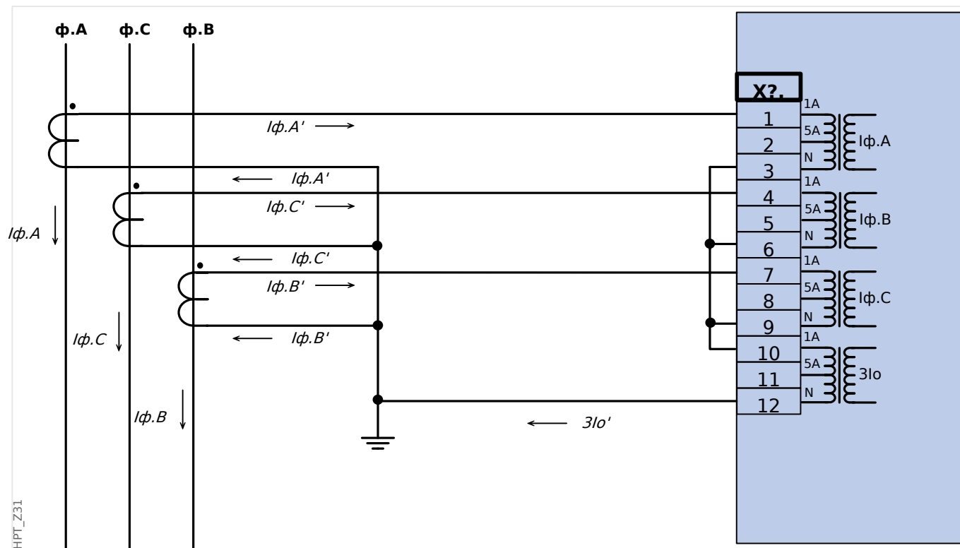
Рис. 24: Измерение фазных токов по схеме «полной» звезды; I_n вторичн. = 1 А. Ток на землю, измеряемый через соединение по схеме Холмгрена 3I_o .ном.втор. = 1 А.
