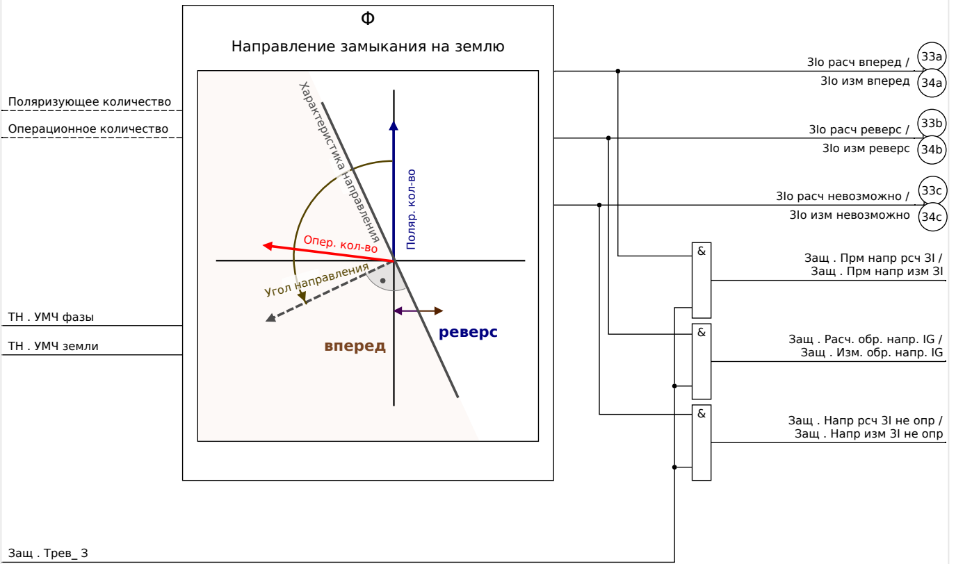
Рис. 65: Определение направления для всех методов, кроме « \cos(\phi) » и « \sin(\phi) ».
