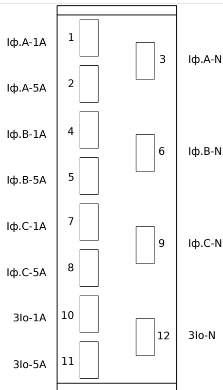
Рис. 18: TIs — электромеханическая адресация
