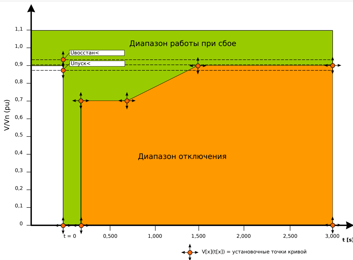
Рис. 79: Область продолжения работы и область отключения.
