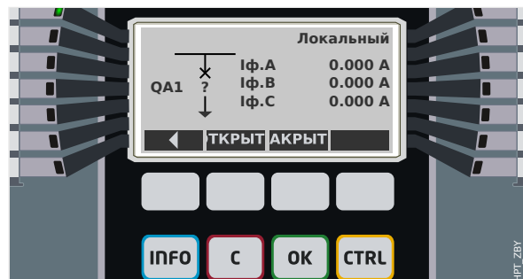
Рис. 120: Пример страницы управления, выключатель в аварийном (недопустимое состояние) положении.
