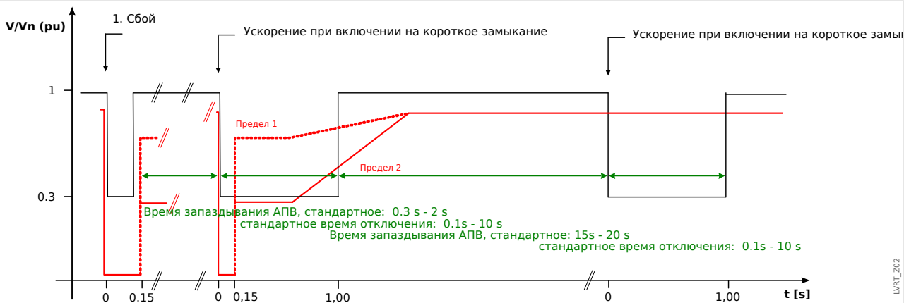
Рис. 78: Кривая напряжения во время двух неудачных попыток автоматического повторного включения; источник: Technische Richtlinie, Erzeugungsanlagen am Mittelspannungsnetz, Ausgabe Juni 2008, BDEW Bundesverband der Energie- und Wasserwirtschaft e.V. (стр. 89.).
