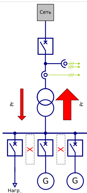
Рис. 98: Децентрализованное использование в сетях с преобладанием энергоснабжения.
