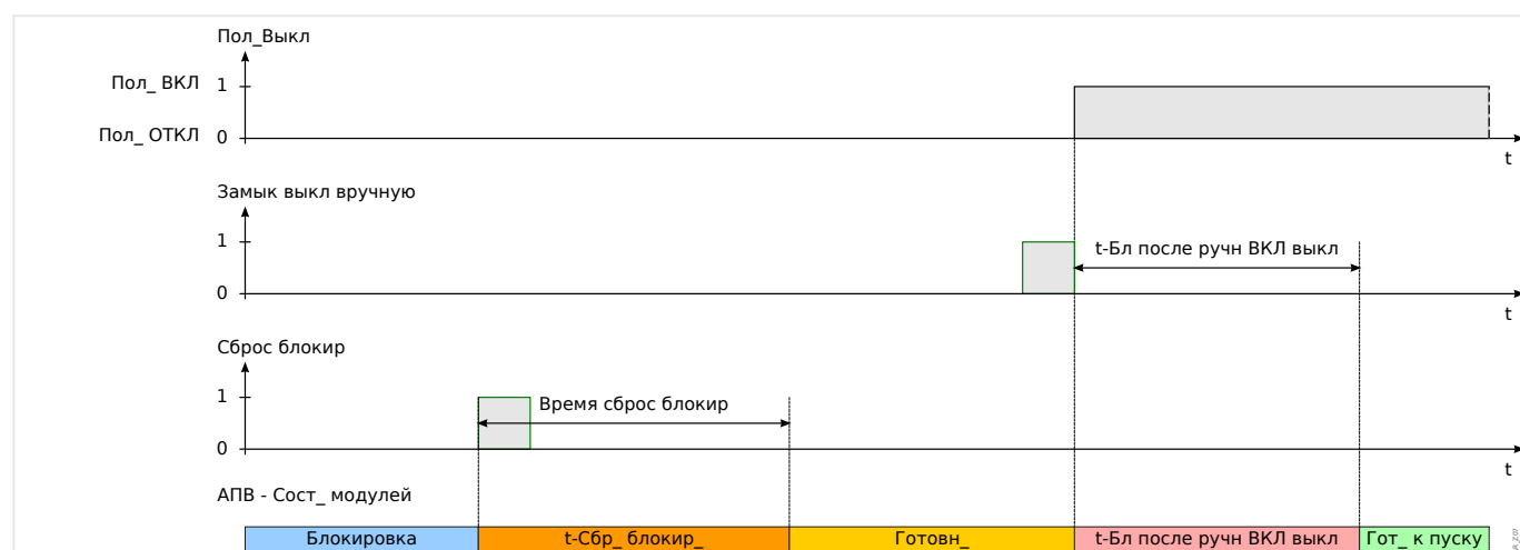
Рис. 107: Логика сброса блокировки АПВ при получении команды сброса блокировки перед замыканием выключателя вручную.
