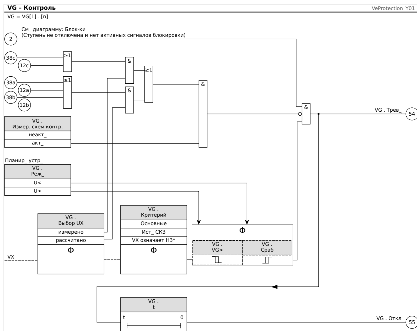
Рис. 81: Контроль напряжения VG, VX, часть 1 (функция контроля, отключение).
