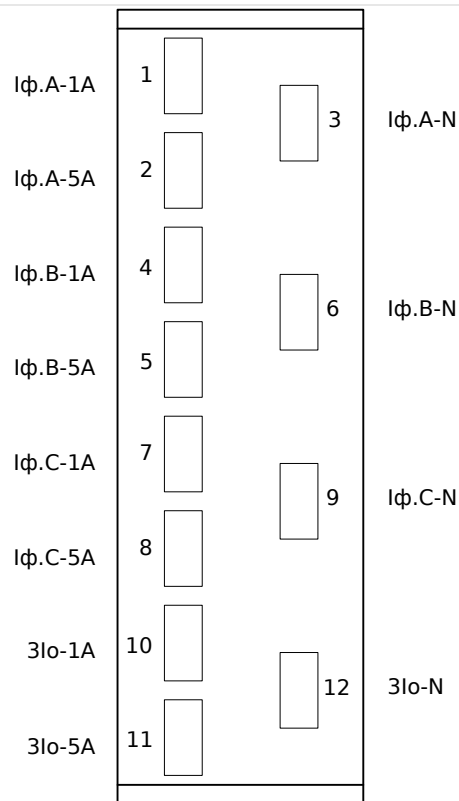
Рис. 16: TI — электромеханическая адресация
