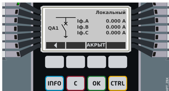
Рис. 121: Пример страницы управления, выключатель в разомкнутом положении.
