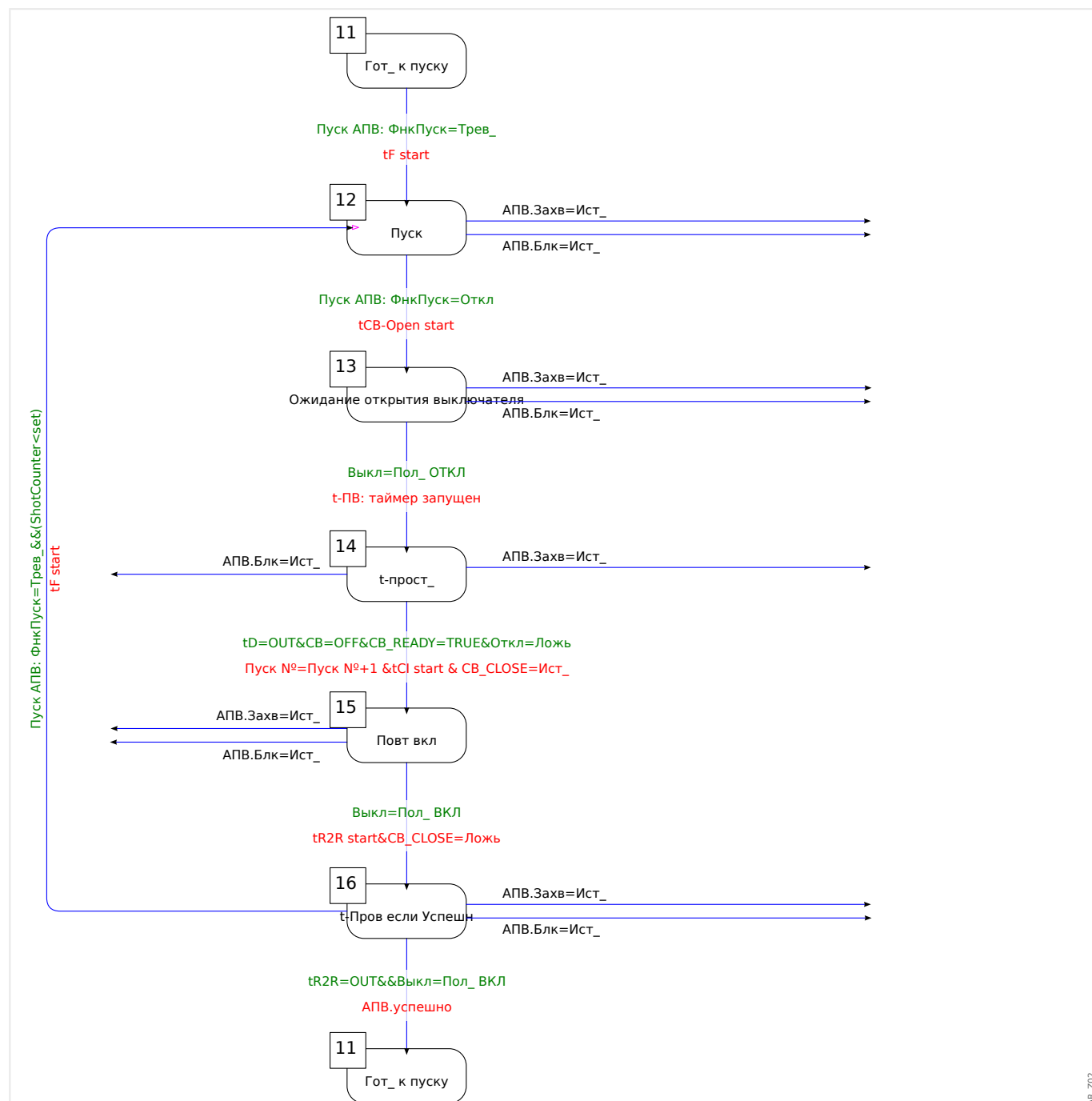
Рис. 102: Цикл выполнения АПВ (состояние 4).
