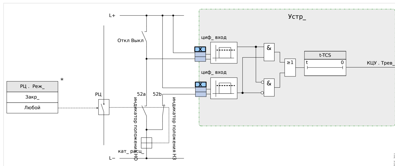
Рис. 115: Пример соединения: контроль цепи отключения с двумя вспомогательными контактами выключателя «Всп Вкл» (52a) и «Всп Выкл» (52b).
