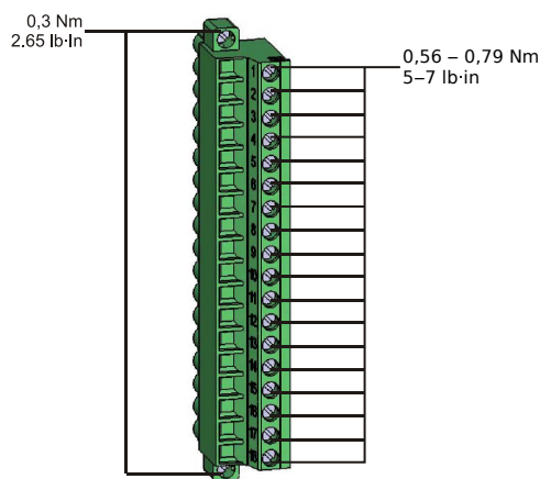
Рис. 139: Измерительные контакты плат измерения напряжения «TU-OR5» и «TU-DI8».
