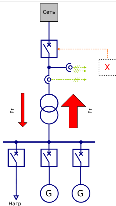
Рис. 97: Централизованное использование в сетях с преобладанием энергоснабжения.
