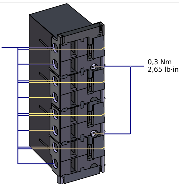
Рис. 137: Штепсельные соединения со встроенными закорачивающими перемычками (стандартные токовые входы)
