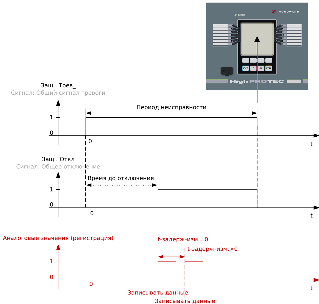
Рис. 129: Регистратор неисправностей: время и длительность.
