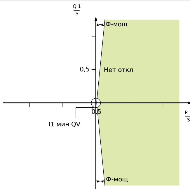
Рис. 99: Метод 1 (контроль угла мощности): «Метод UFLS» = «Контроль угла мощности».
