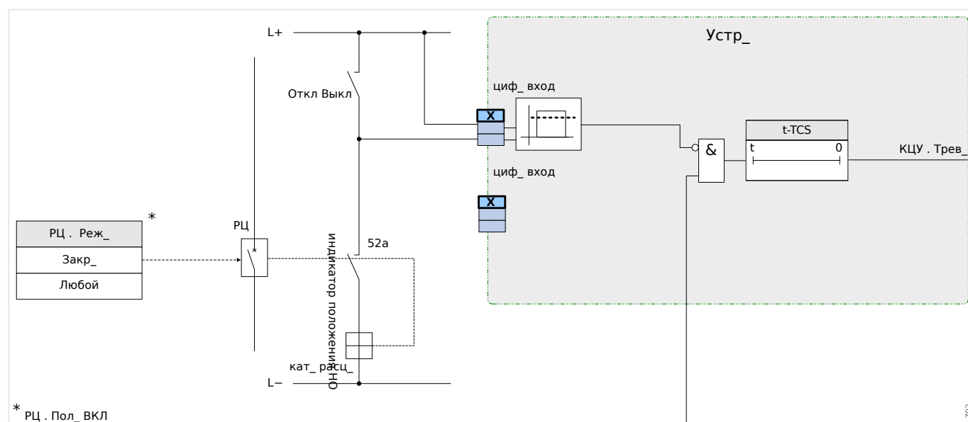
Рис. 116: Пример соединения: контроль цепи отключения только с одним вспомогательным контактом выключателя «Всп Вкл» (52a).
