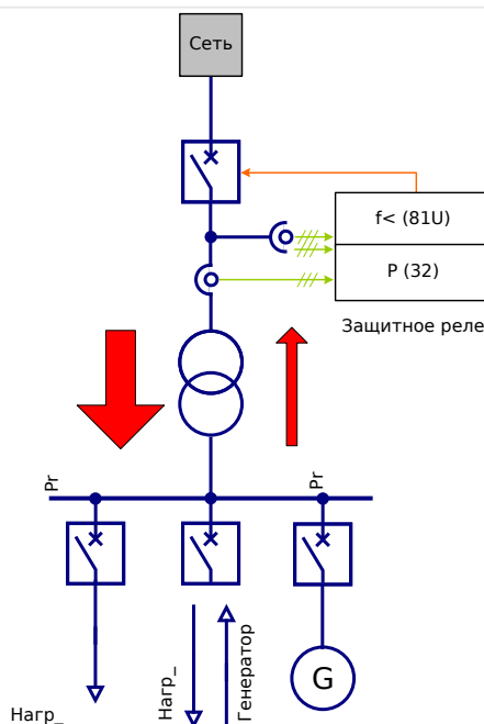
Рис. 95: Централизованная автоматическая частотная разгрузка в сетях с временным электроснабжением
