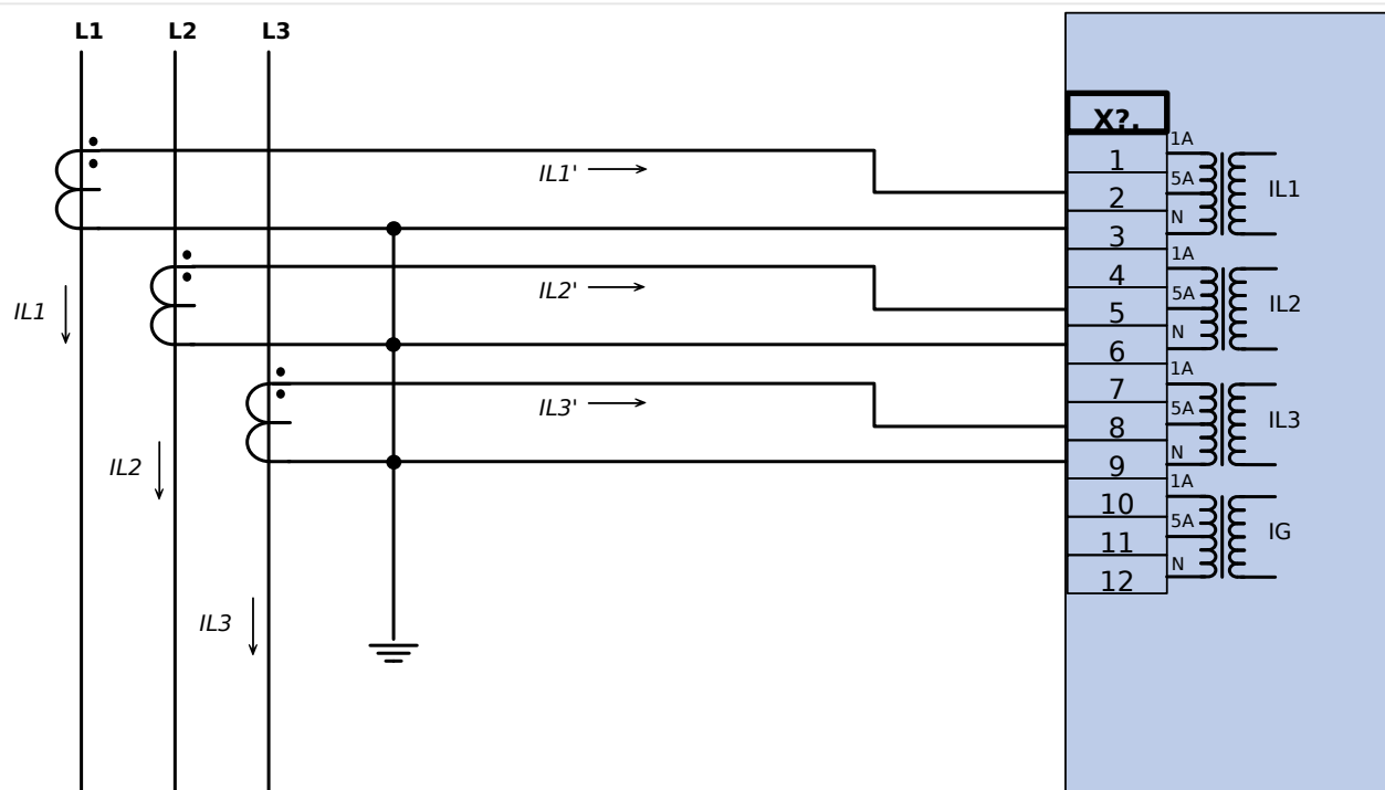
Fig. 19: Medição de corrente de trifásica; I_n secundário = 5 A
