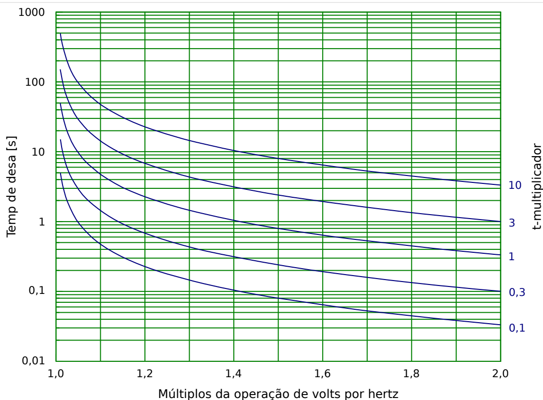
Fig. 88: Característica/formato da curva: INV A
