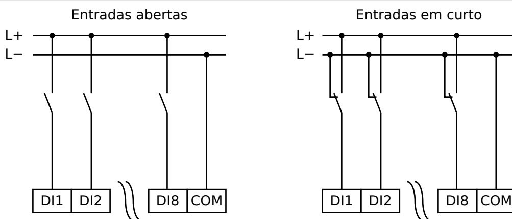
Fig. 156: Estado seguro das entradas digitais
