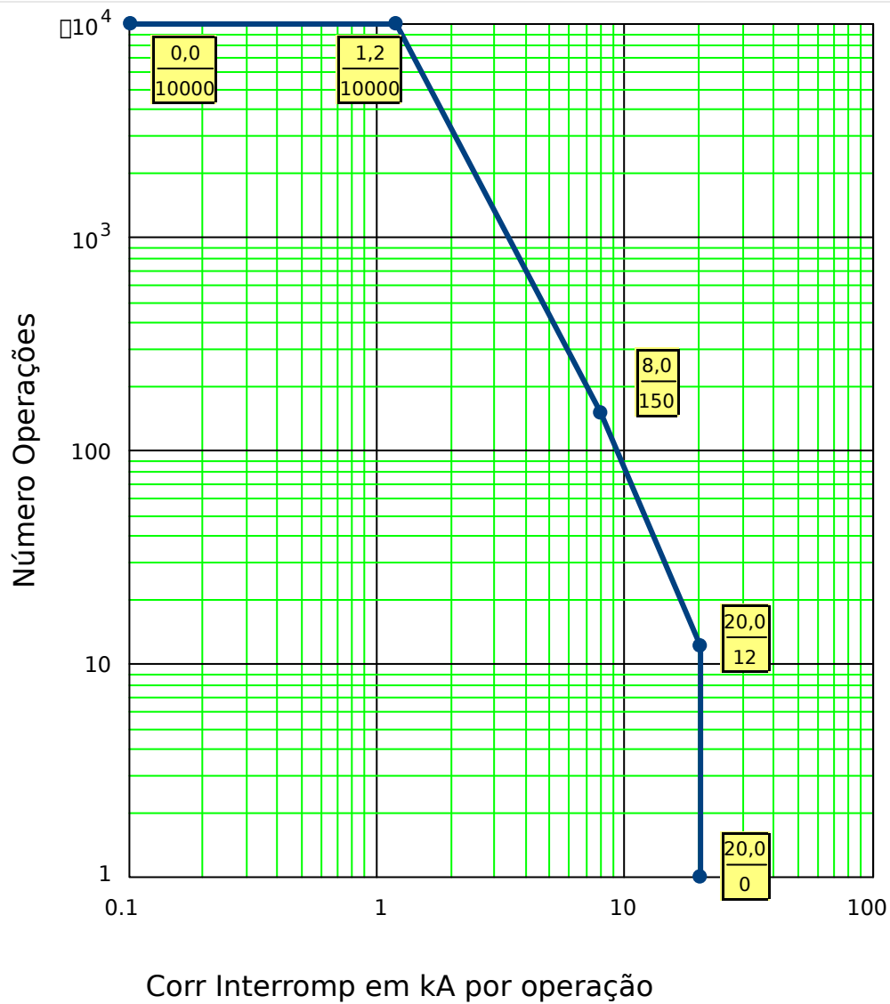
Fig. 140: Curva Manutenção de Disjuntor para Disjuntor normal 25kV
