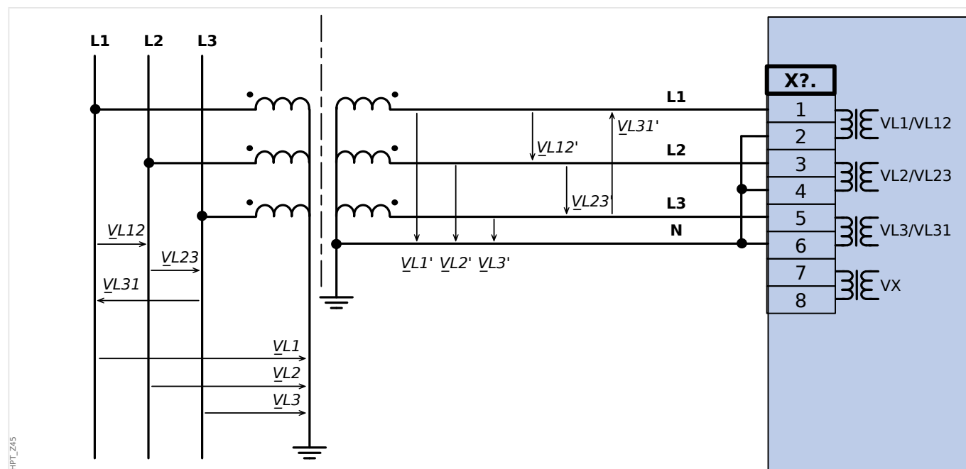
Fig. 30: VT Wye: Medição de voltagem trifásica - fiação das entradas de medição: "conexão estrela"
