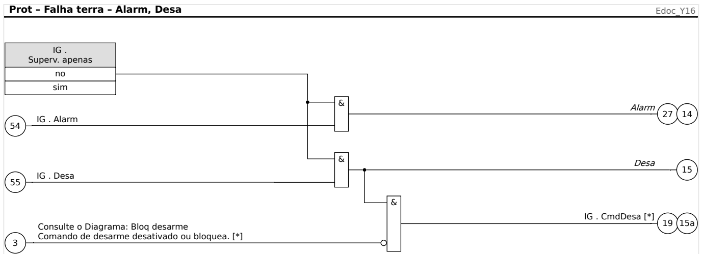
Fig. 86: Proteção de sobrecorrente de solo (aterramento), parte 2 (comando de disparo do alarme geral e disparo geral).
