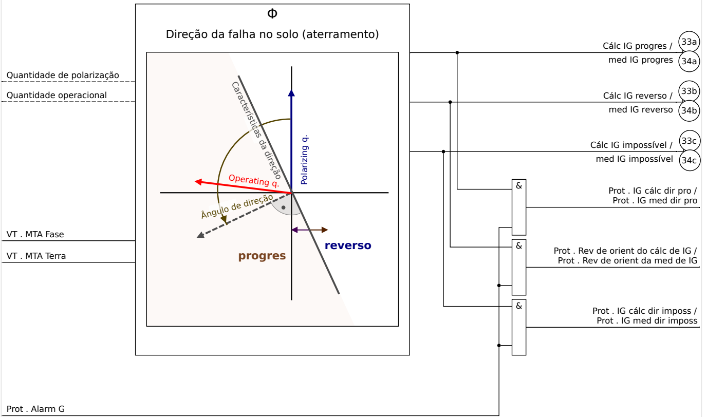
Fig. 67: Determinação da direção para todos os métodos, exceto " \cos(\phi) ", " \sin(\phi) ".
