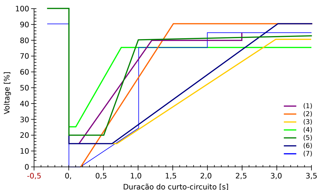
Fig. 125: Padrões LVRT; fonte: eBWK Bd. 60 (2008) Nr. 4. Autores: Dipl.-Ing. Thomas Smolka, Dr.-Ing. Karl-Heinz Weck, Zertifizierungstelle der FGH e.V., Mannheim, sowie Dipl.-Ing. (FH) Matthias Bartsch, Enercon GmbH, Aurich.
