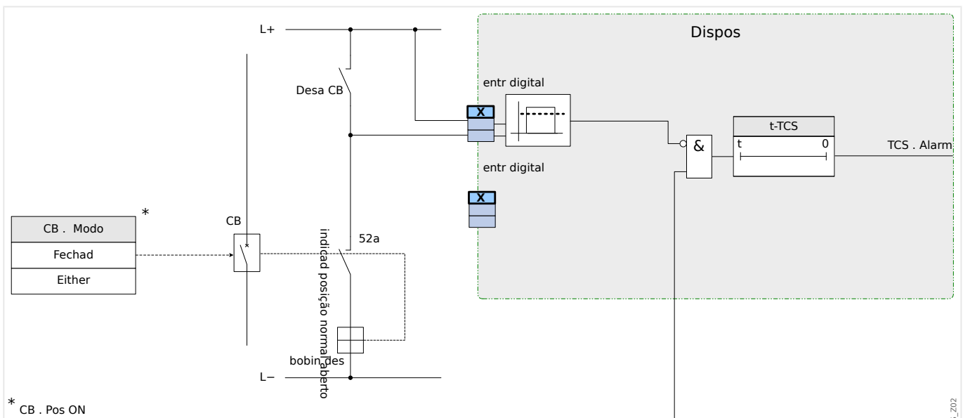
Fig. 132: Exemplo de conexão: Supervisão do circuito de disparo com apenas um contato CB auxiliar »Aux ON« (52a).
