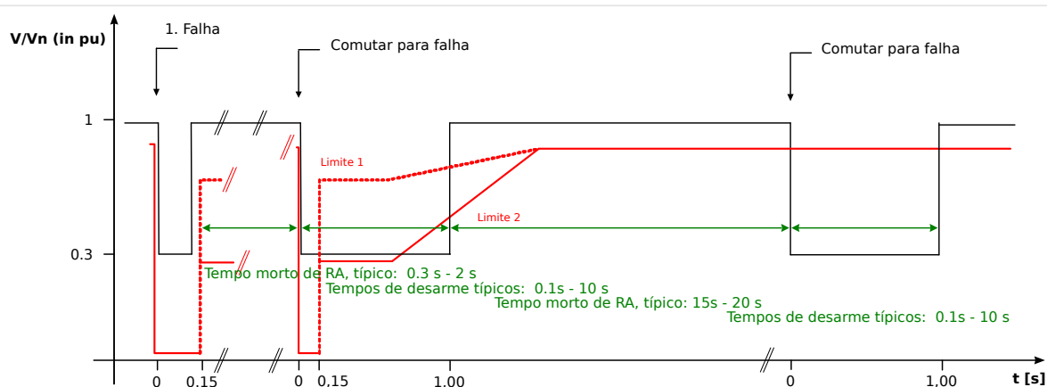
Fig. 126: Percurso de uma curva de tensão durante um autorreligamento malsucedido de dois disparos; fonte: Technische Richtlinie, Erzeugungsanlagen am Mittelspannungsnetz, Ausgabe Juni 2008, BDEW Bundesverband der Energie- und Wasserwirtschaft e.V. (página 89).
