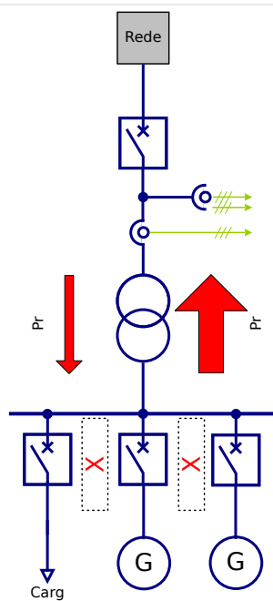
Fig. 122: Uso descentralizado em redes com fonte de alimentação predominante.
