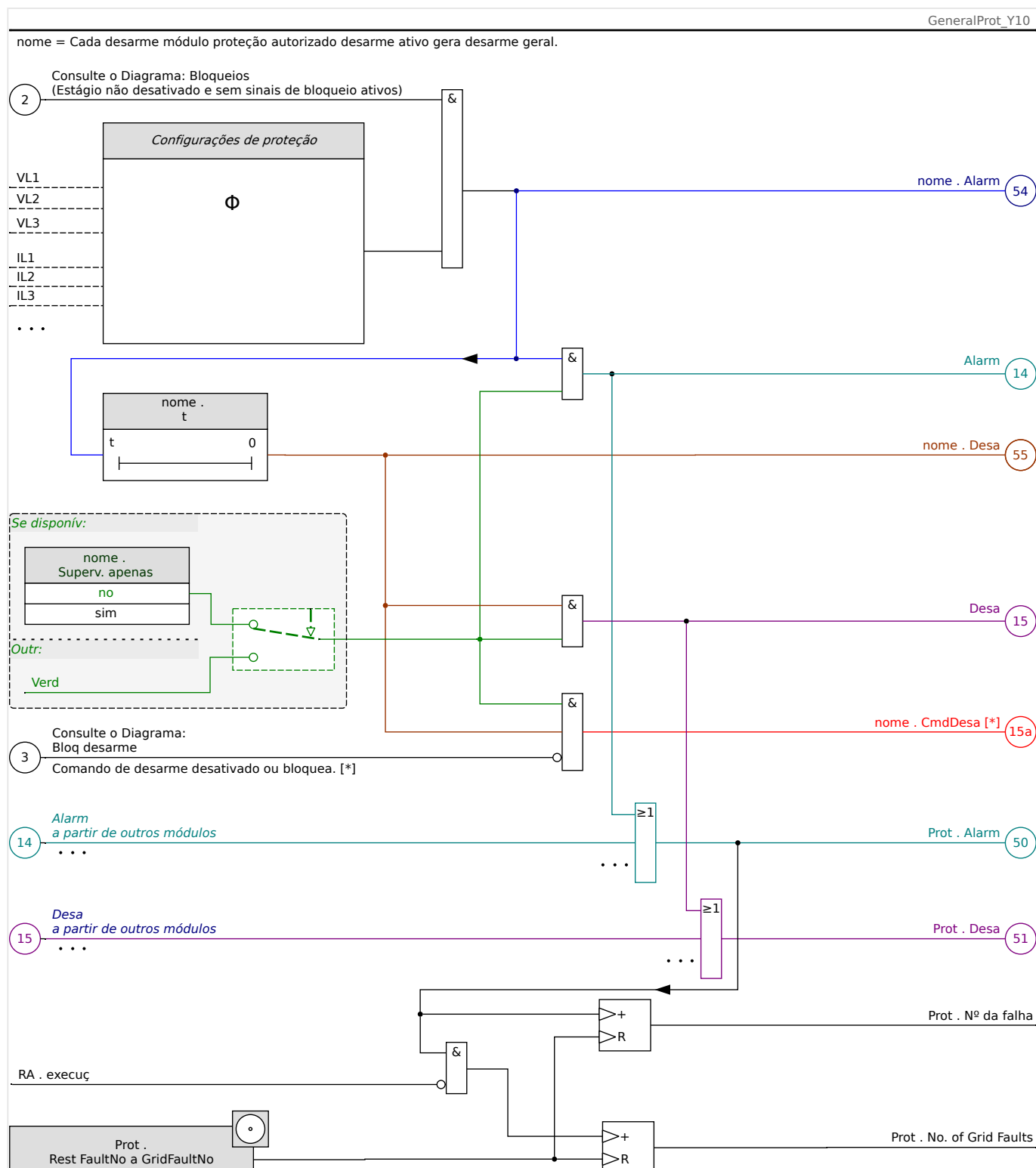
Fig. 63: Esboço rápido da funcionalidade de qualquer HighPROTEC elemento de proteção.
