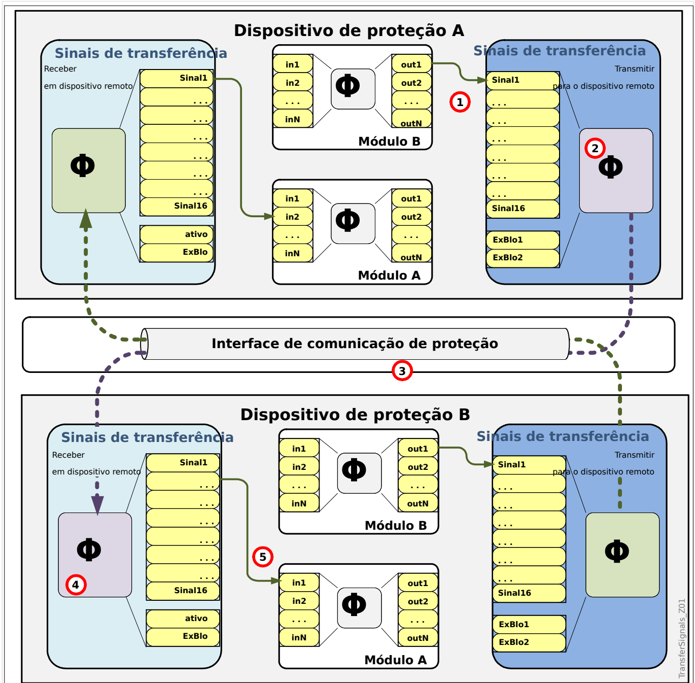
Fig. 84: Princípio da funcionalidade do »Trans-Sinal«.
