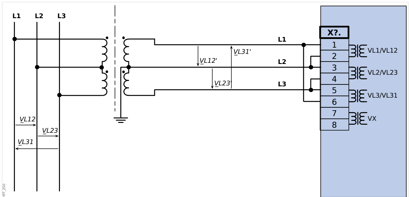
Fig. 34: Medição de tensão bifásica - fiação das entradas de medição: "Delta Aber"
