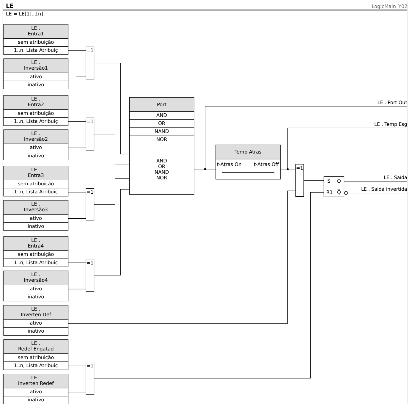
Fig. 147: Visão Geral Detalhada - Diagrama Lógico Geral.
