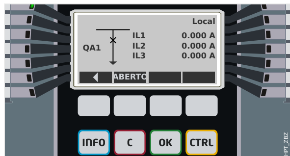
Fig. 135: Exemplo de página de controle, com o "Disjuntor" na posição fechada.
