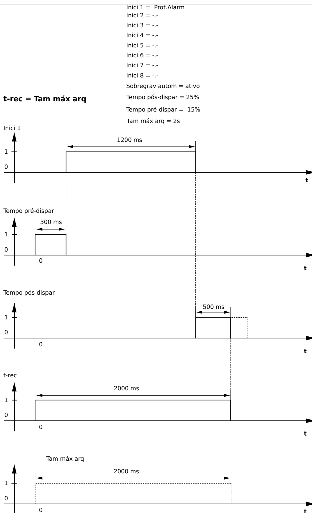
Fig. 143: Exemplo de Gráfico de Prazo do Gravador de Perturbação I
