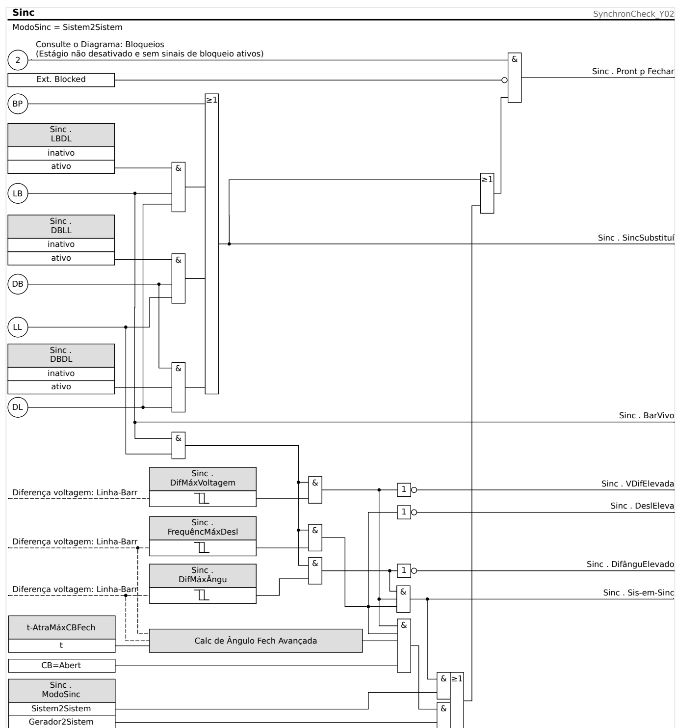
Fig. 113: Funcionalidade do módulo »Sinc«, "Sistem2Sistem".
