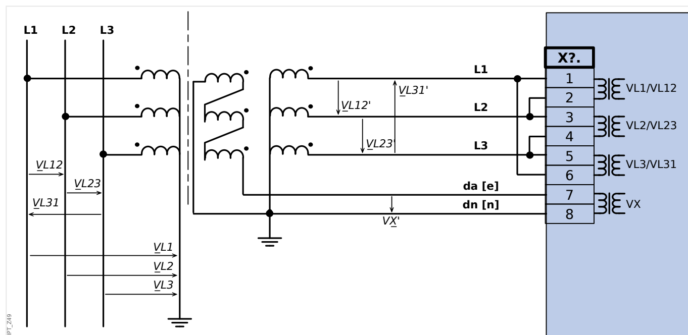
Fig. 33: Medição VG tensão residual por meio de "delta aberto" (e-n) de circuito auxiliar
