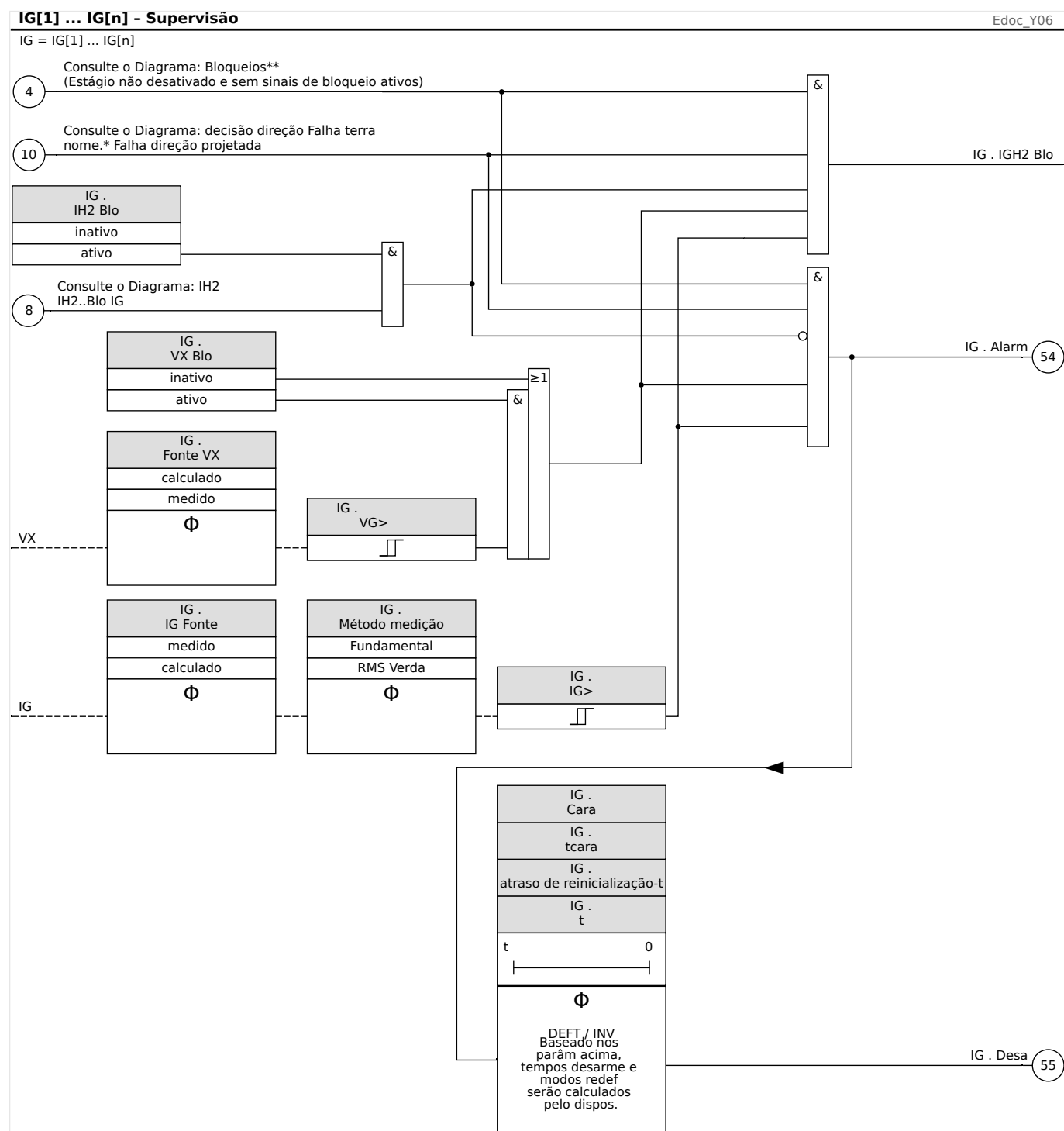
Fig. 85: Proteção de sobrecorrente de solo (aterramento), parte 1 (função de supervisão, decisão de disparo).
