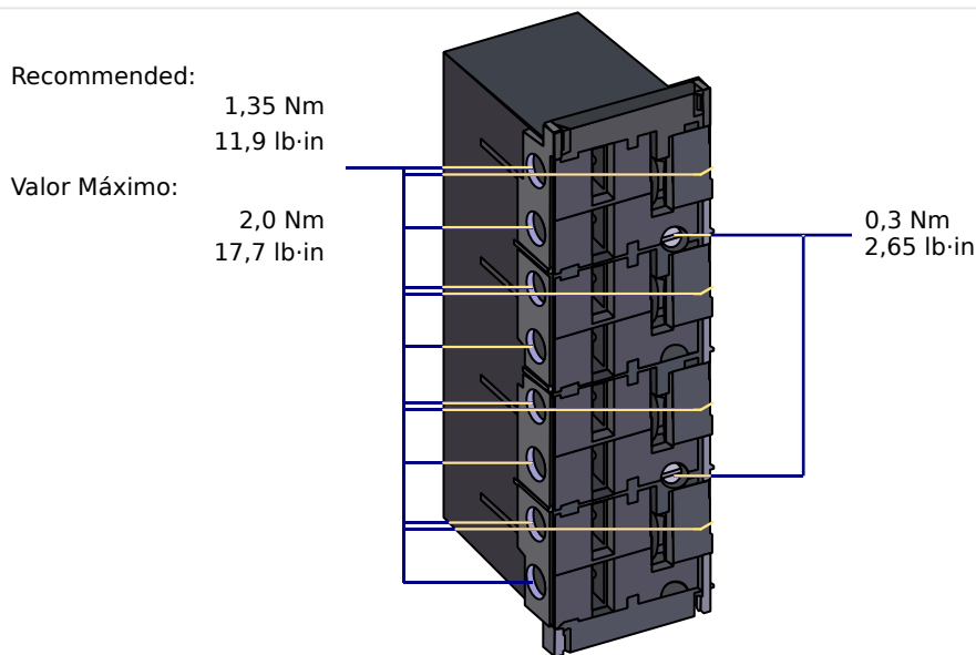
Fig. 153: Conector plug-in com acionador de curto-circuito integrado (entradas de corrente convencionais)
