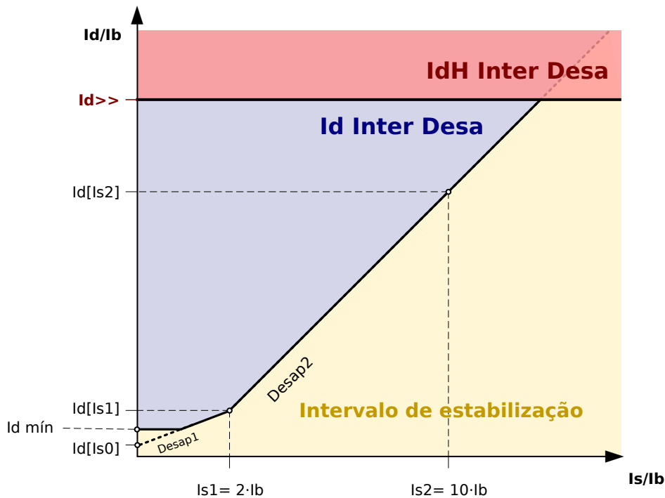
Fig. 76: As curvas de disparo das funções de proteção de "Id" (área azul) e de "IdH" (área vermelha).
