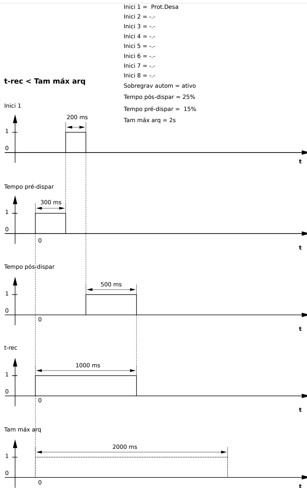
Fig. 144: Exemplo de Gráfico de Prazo do Gravador de Perturbação II
