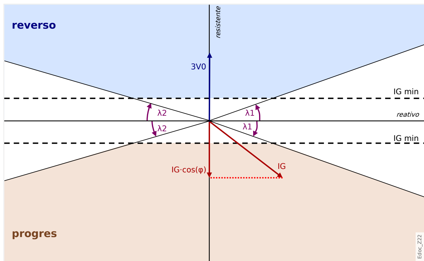
Fig. 68: Princípio de determinação da direção para o método " \cos(\phi) ".
