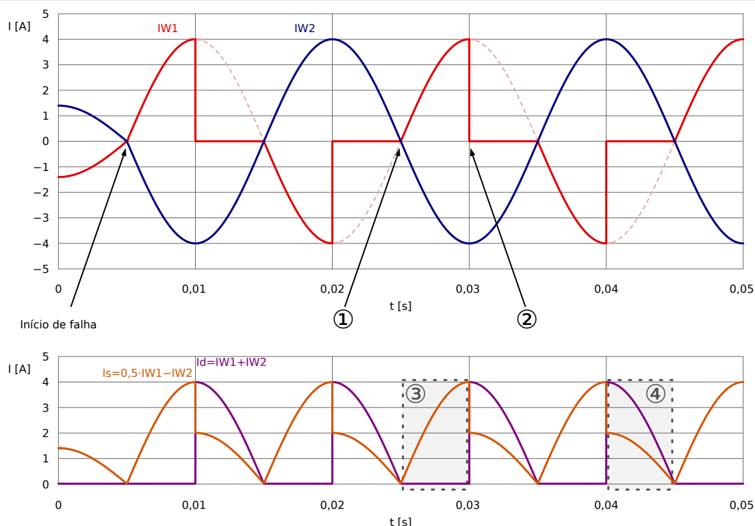
Fig. 78: Característica de I_d e I_s com a saturação no lado W1 para uma falha externa.
