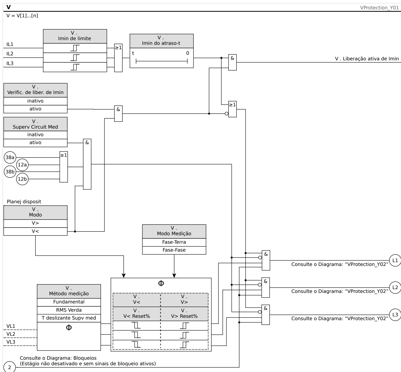
Fig. 100: Funcionalidade do módulo de proteção de tensão, parte 1.
