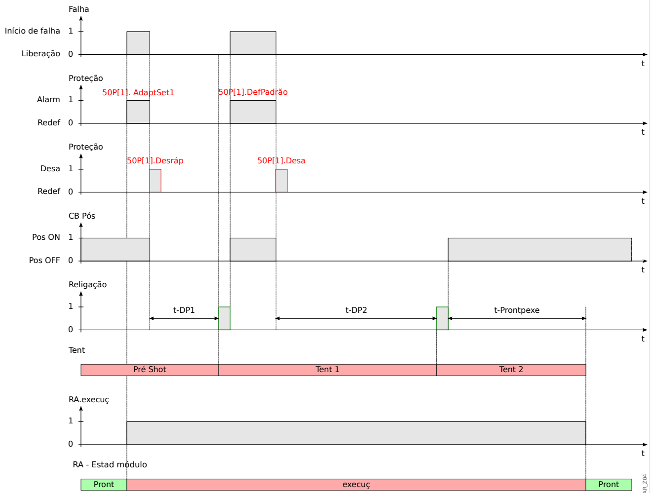
Fig. 95: Diagrama de temporização de religamento automático para esquema de religamento de 2 tentativas bem-sucedidas com aceleração na pré tentativa
