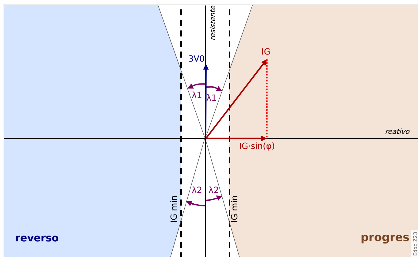
Fig. 69: Princípio de determinação da direção para o método " \sin(\phi) ".
