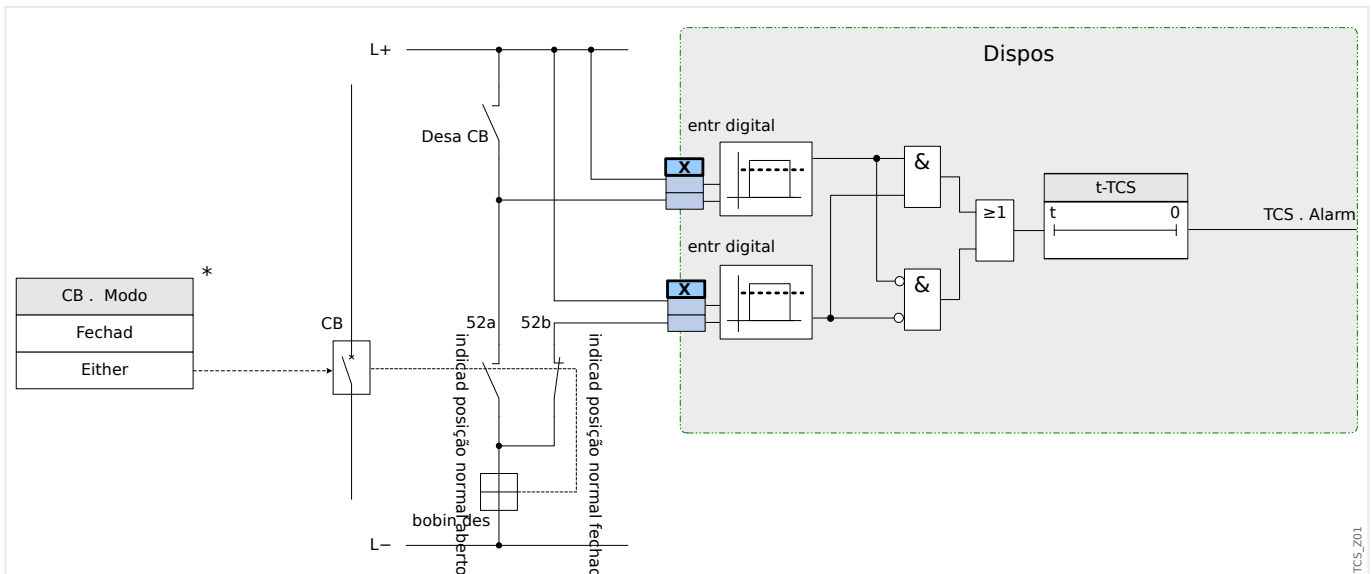
Fig. 131: Exemplo de conexão: Supervisão do circuito de disparo com dois contatos CB auxiliares »Aux ON« (52a) e »Aux OFF« (52b).
