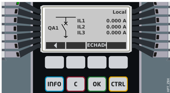
Fig. 137: Exemplo de página de controle, com o "Disjuntor" na posição aberta.
