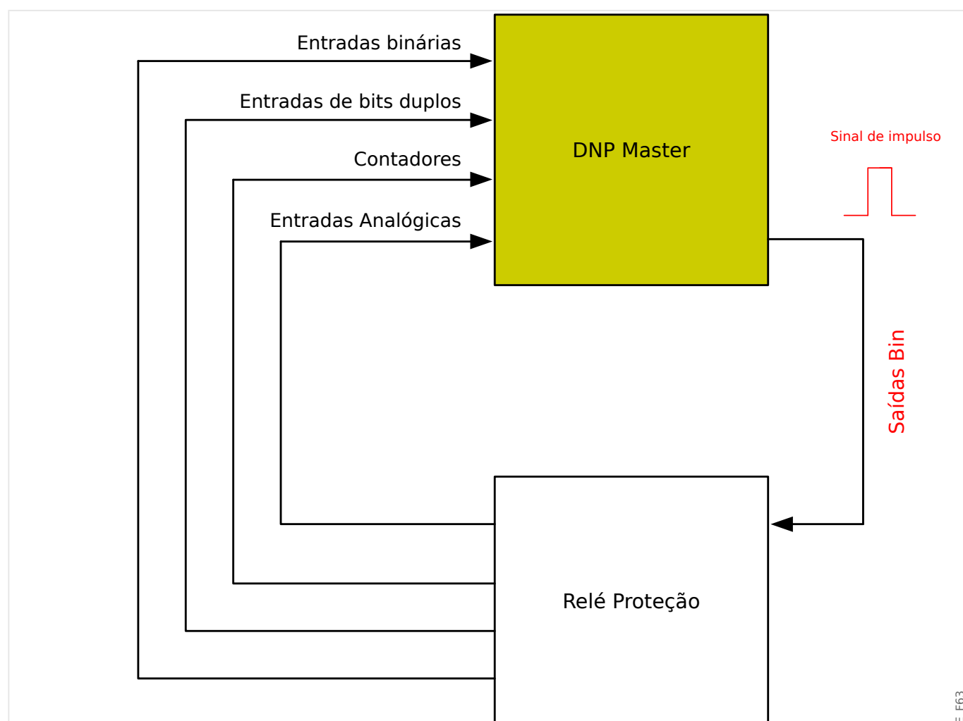
Fig. 58: Mapeamento de pontos
