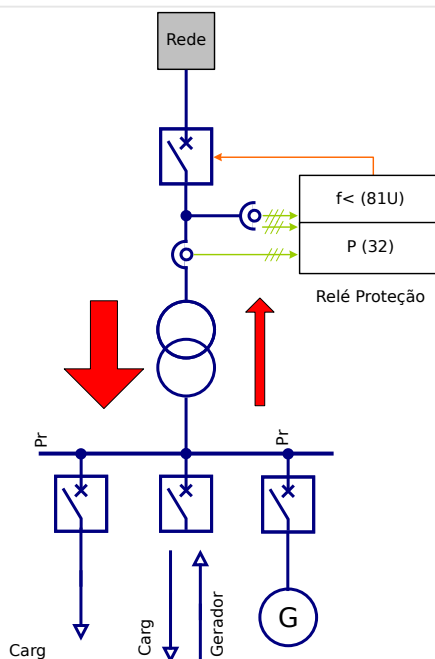
Fig. 119: Derramamento de carga de subfrequência centralizada em redes com fornecimento temporário de energia.
