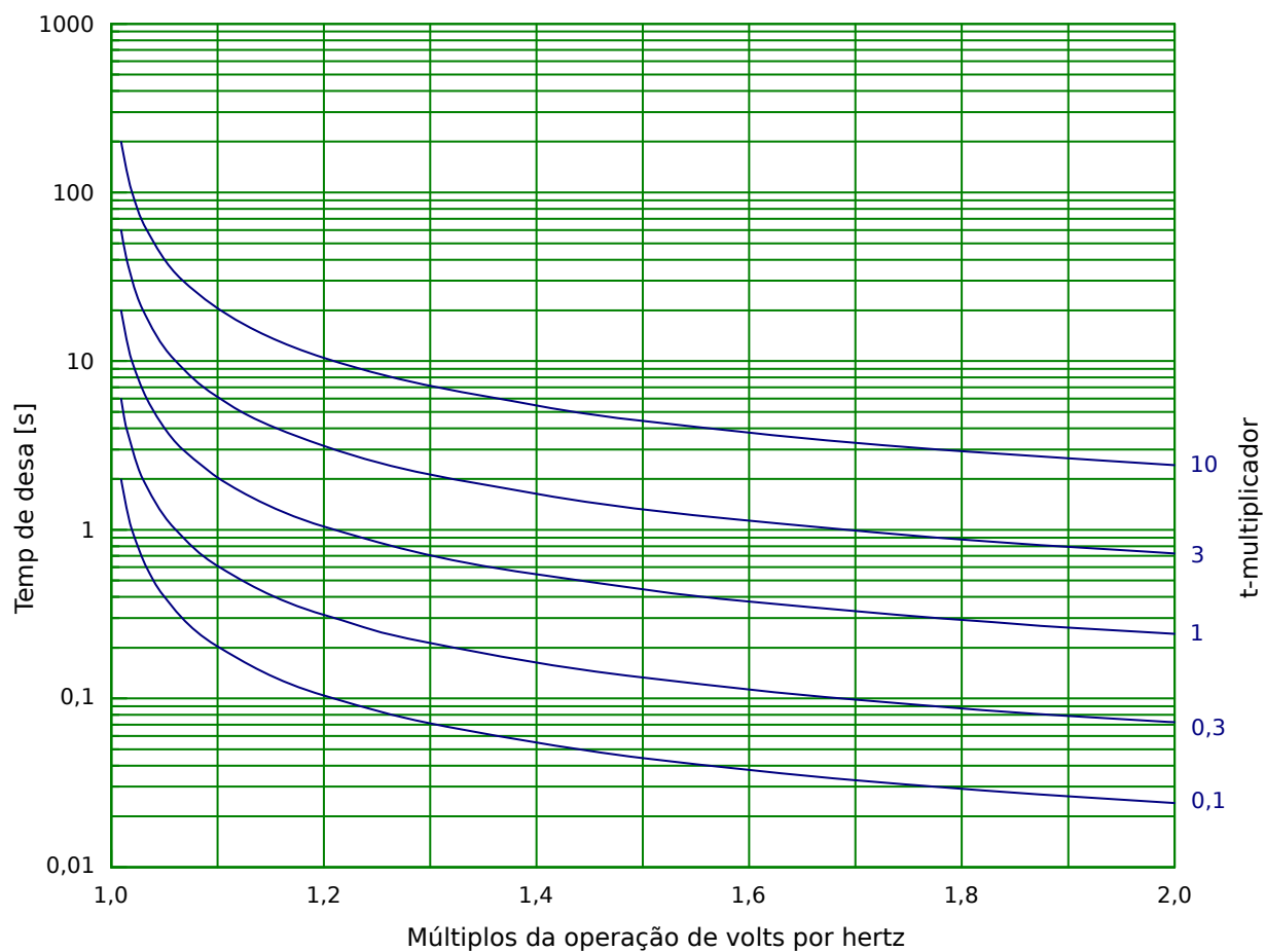
Fig. 90: Característica/formato da curva: INV C
