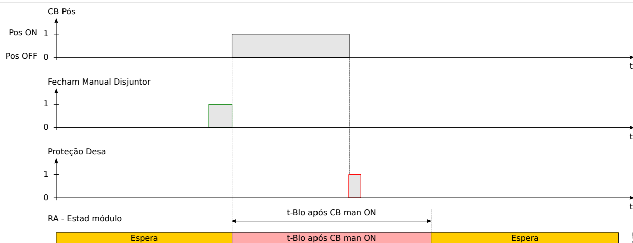
Fig. 97: Disparo de proteção enquanto o tempo de bloqueio de fechamento manual está cronometrando.
