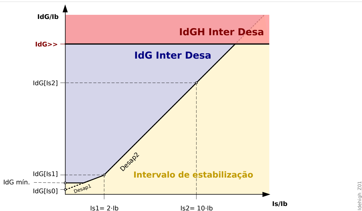
Fig. 81: Valor de arranque " I_dG>> " da corrente diferencial de aterramento com base na corrente nominal " I_b " do objeto de proteção relacionado.
