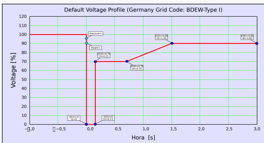
Fig. 128: Perfil padrão do LVRT (BDEW-Tipo I).
