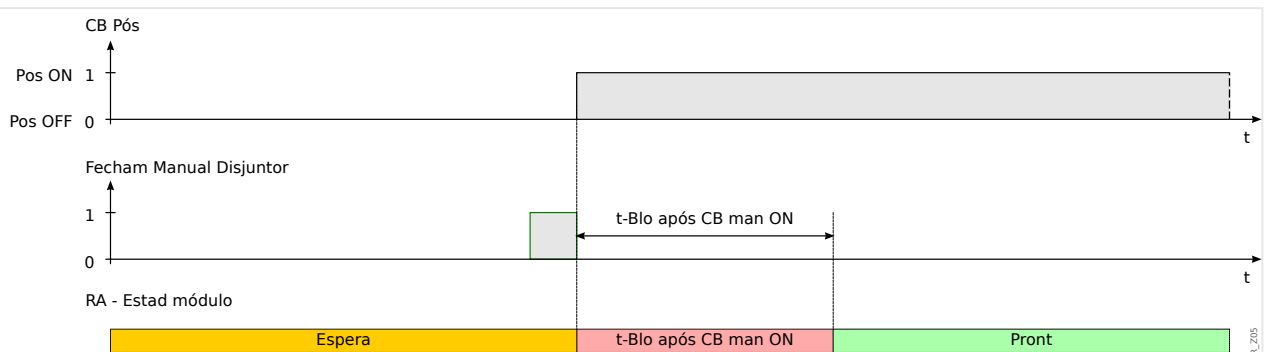
Fig. 96: Estados de religamento automático durante fechamento manual do disjuntor
