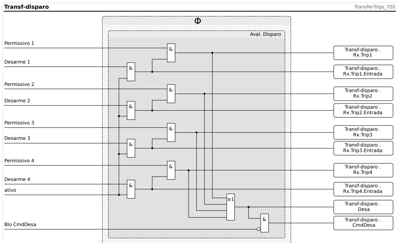
Fig. 83: Funcionalidade do módulo »Transf-disparo« (parte 3).
