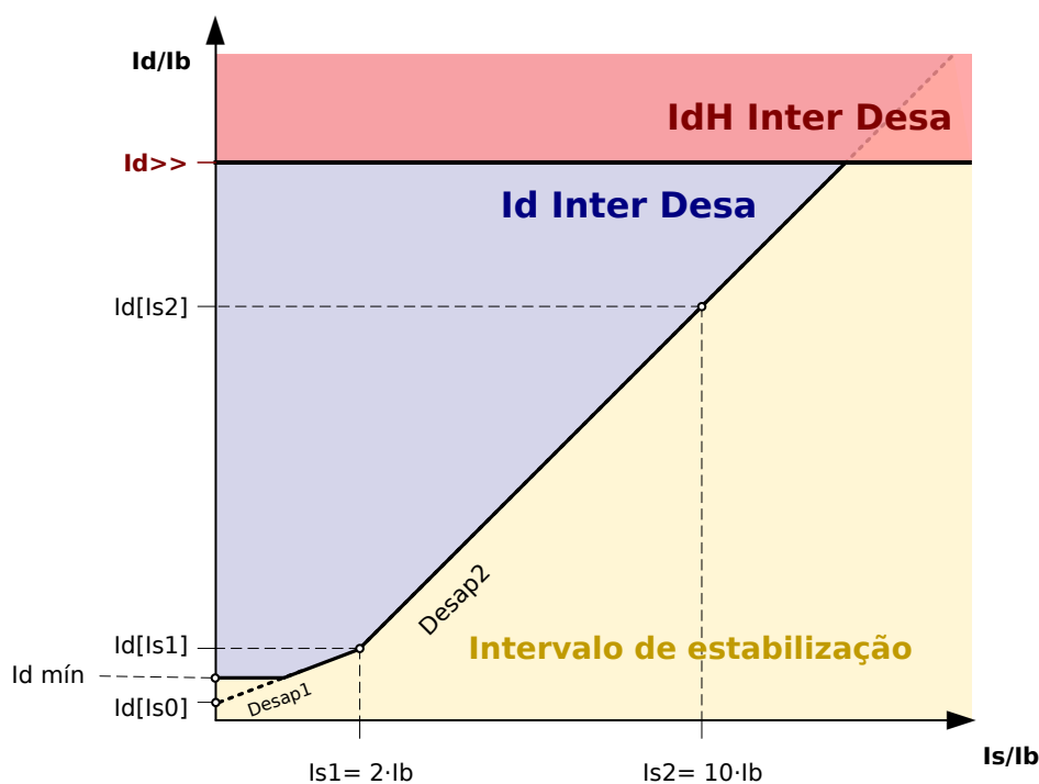
Fig. 79: Etapa da Proteção Diferencial Irrestrita de Alta Definição IdH.
