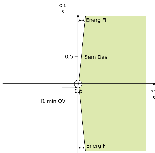
Fig. 123: Método 1 (Supervisão de Ângulo de Energia): “Método UFLS” = “Supervisão Âng Energ”.
