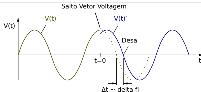
Fig. 108: Aumento de vetor de tensão.
