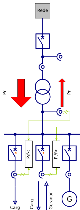
Fig. 120: Eliminação de carga de subfrequência descentralizada em redes com fornecimento temporário de energia.
