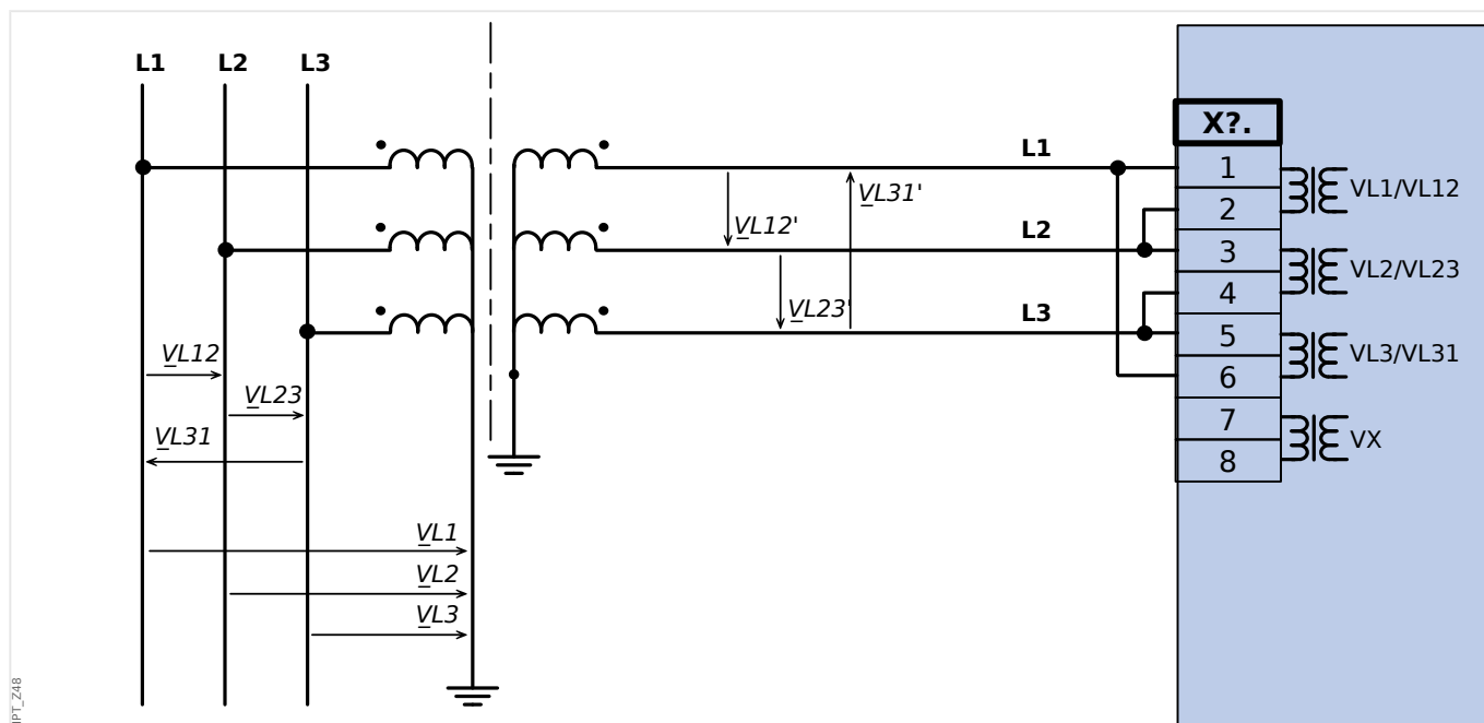
Fig. 32: Medição de tensão trifásica - fiação das entradas de medição: "conexão-delta"
