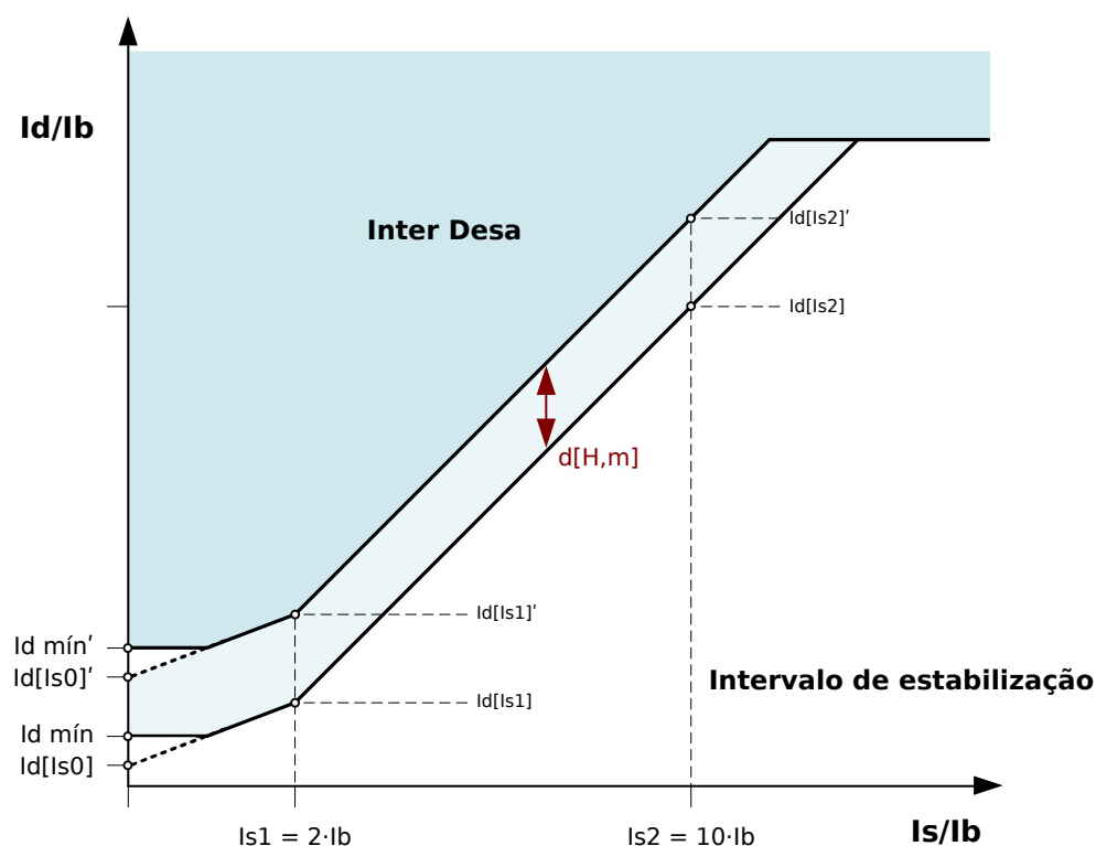
Fig. 77: Aumento Dinâmico Temporário da Característica de Disparo Estático
