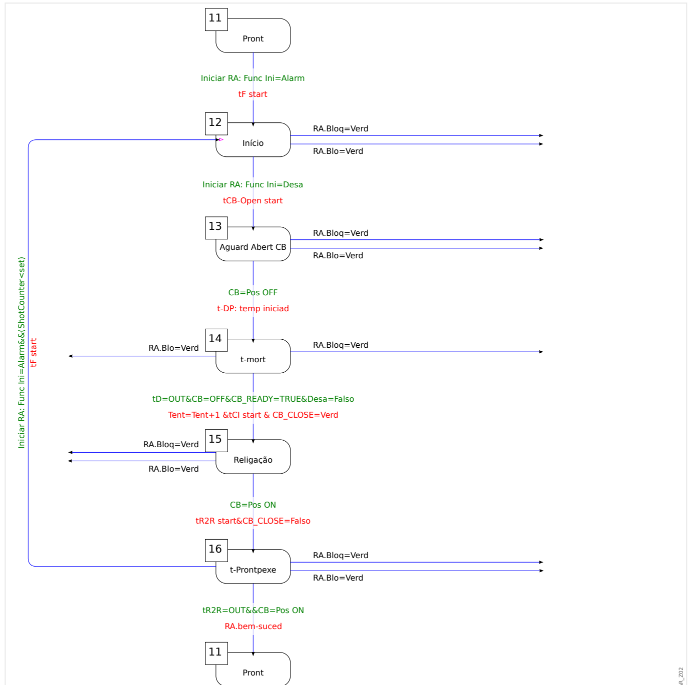
Fig. 93: Ciclo de execução de RA (estado 4).
