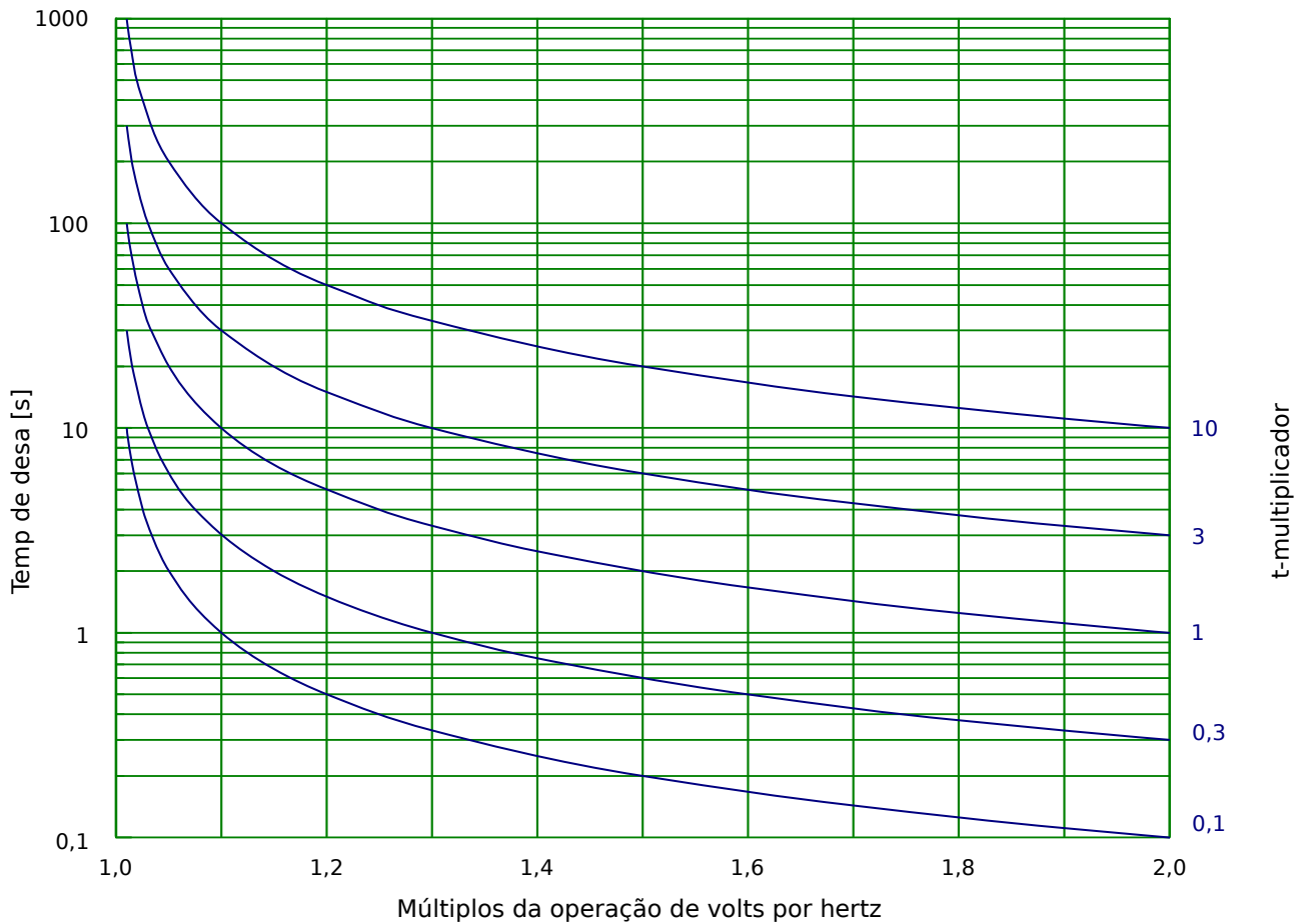
Fig. 89: Característica/formato da curva: INV B
