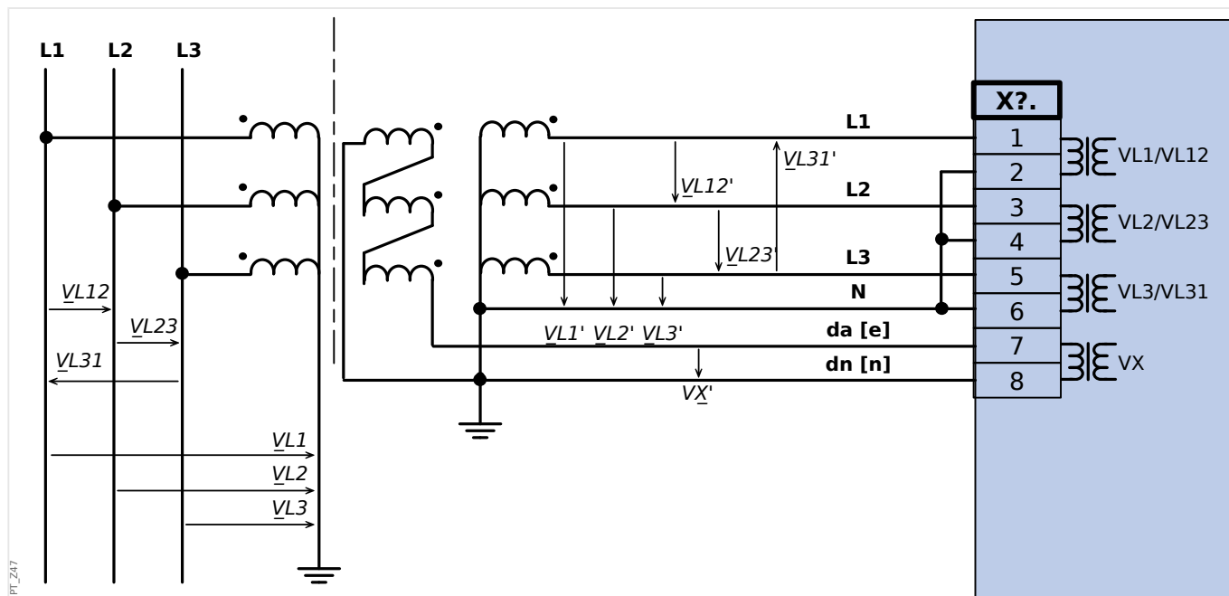
Fig. 31: VT Wye com conexão Broken Delt.
