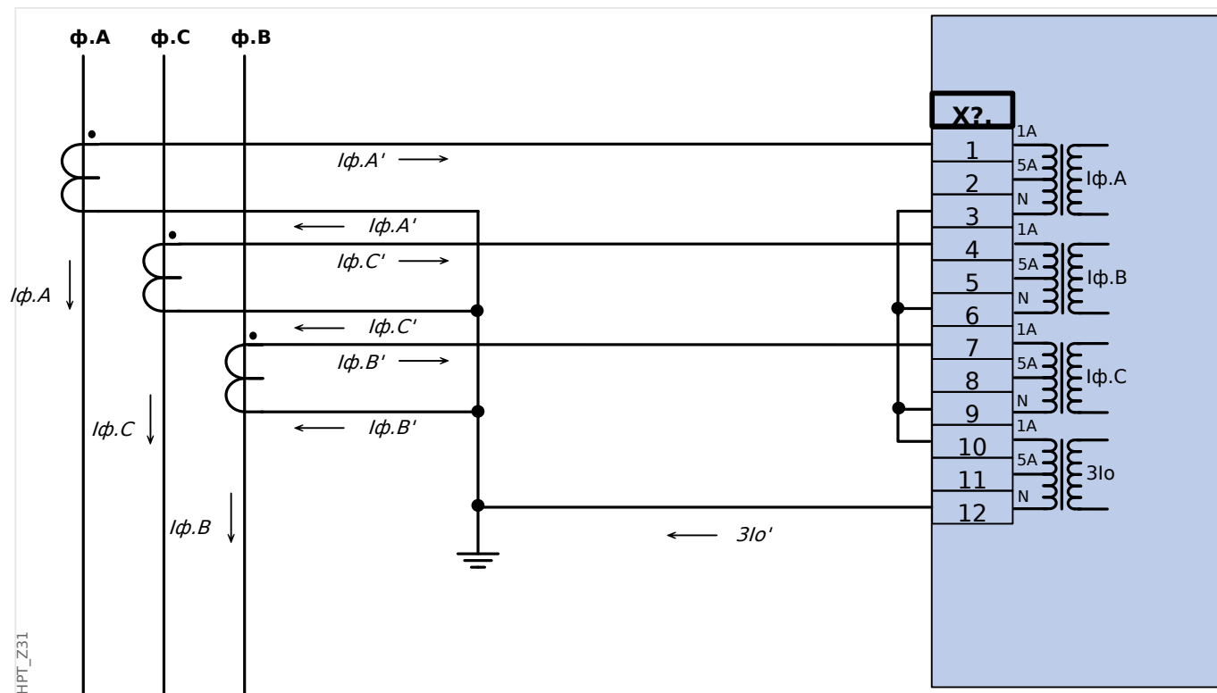
Рис. 24: Измерение фазных токов по схеме «полной» звезды; I_n вторичн. = 1 А. Ток на землю, измеряемый через соединение по схеме Холмгрена 3I_{0\text{ном.втор.}} = 1 А.
