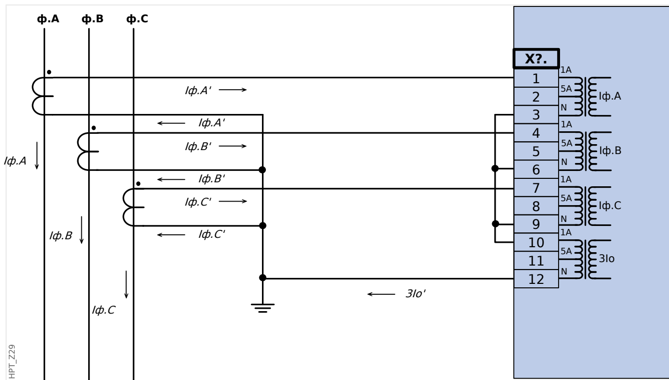
Рис. 22: Измерение фазных токов по схеме «полной» звезды; I_n вторичн. = 1 А. Ток на землю, измеряемый через соединение по схеме Холмгрена 3I_o .ном.втор. = 1 А.
