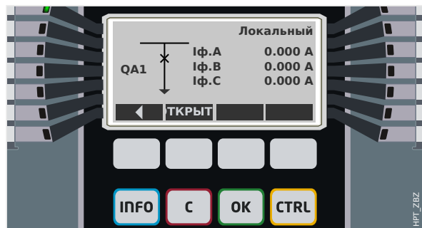
Рис. 135: Пример страницы управления, выключатель в замкнутом положении.
