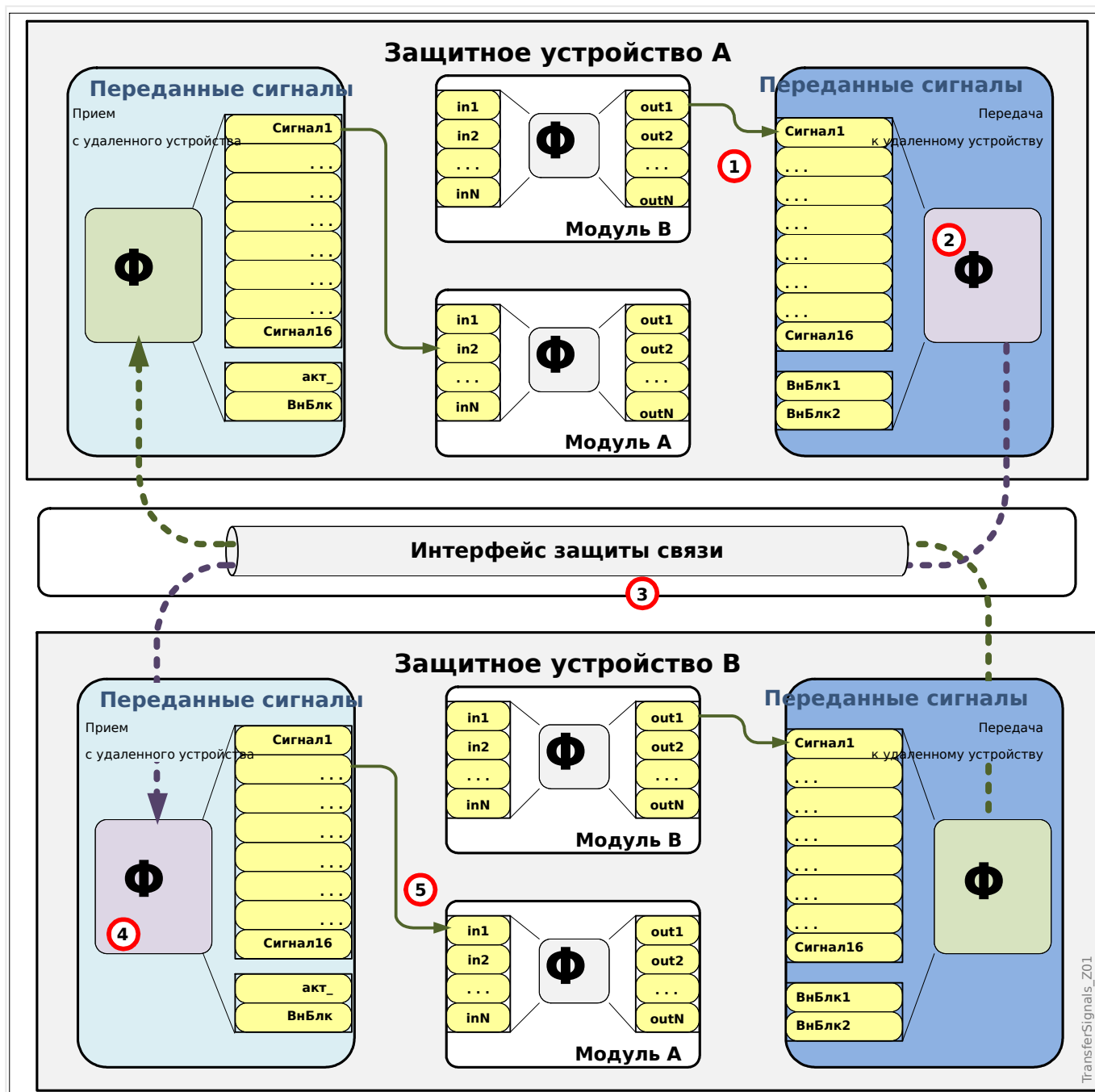
Рис. 84: Принцип работы «Передача сигнала».
