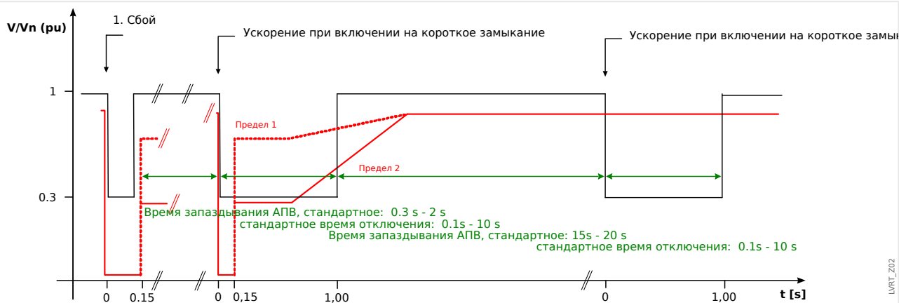
Рис. 126: Кривая напряжения во время двух неудачных попыток автоматического повторного включения; источник: Technische Richtlinie, Erzeugungsanlagen am Mittelspannungsnetz, Ausgabe Juni 2008, BDEW Bundesverband der Energie- und Wasserwirtschaft e.V. (стр. 89.).
