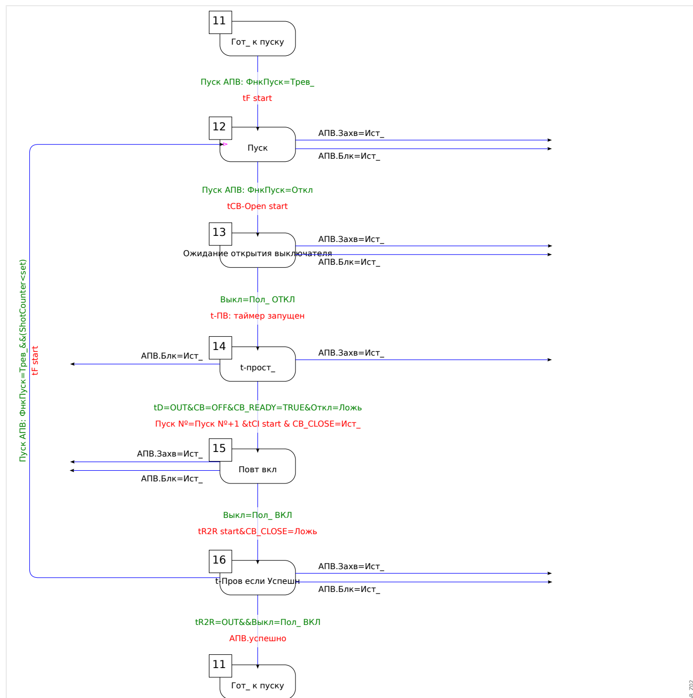
Рис. 93: Цикл выполнения АПВ (состояние 4).
