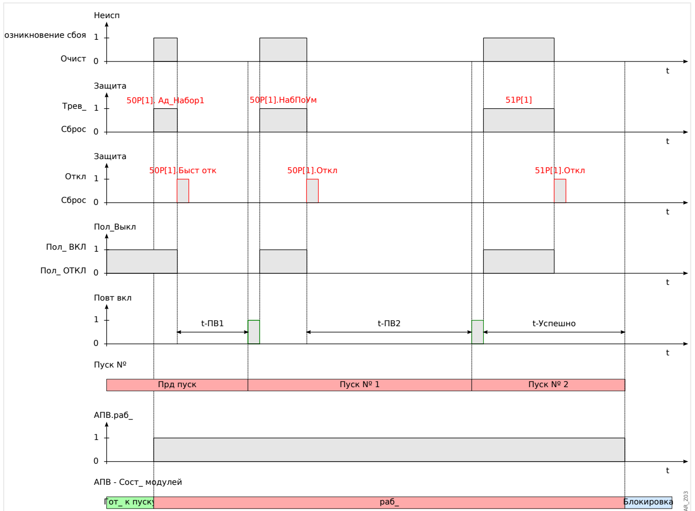
Рис. 94: Диаграмма синхронизации автоматического повторного включения для схемы с 2 неудачными попытками автоматического повторного включения и ускорением перед импульсом.
