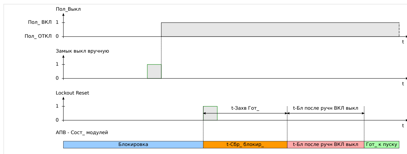
Рис. 99: Логика сброса блокировки АПВ при получении команды сброса блокировки после замыкания выключателя вручную.
