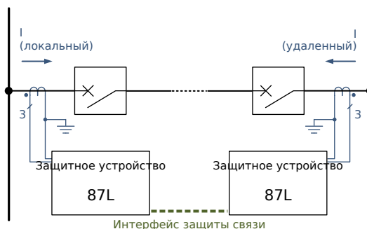
Рис. 74: ANSI 87L — дифференциальная защита линии.
