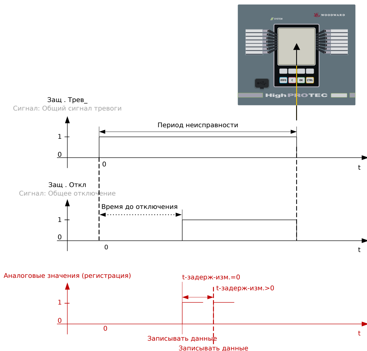
Рис. 145: Регистратор неисправностей: время и длительность.
