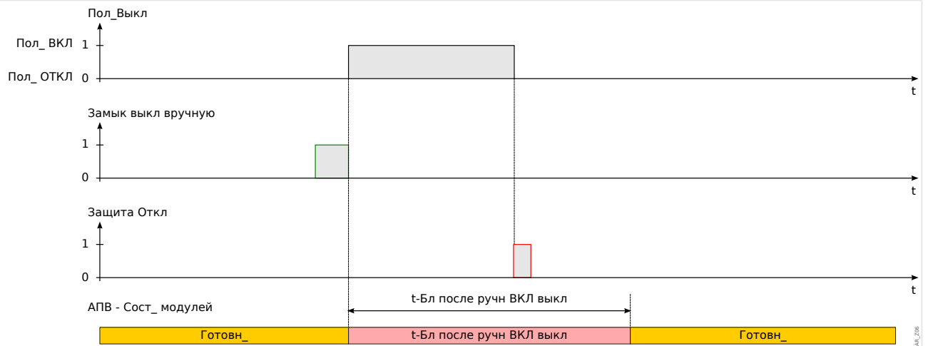
Рис. 97: Отключение защиты во время работы таймера блокировки замыкания вручную.
