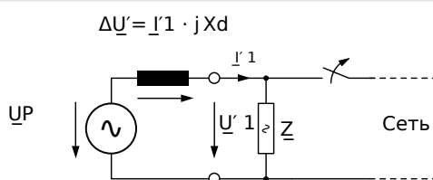
Рис. 106: Эквивалентная цепь при сбое электросети.
