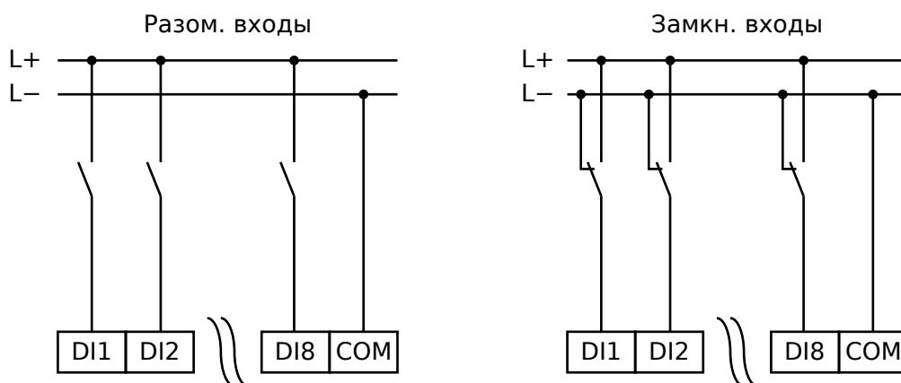
Рис. 156: Безопасное состояние цифровых входов
