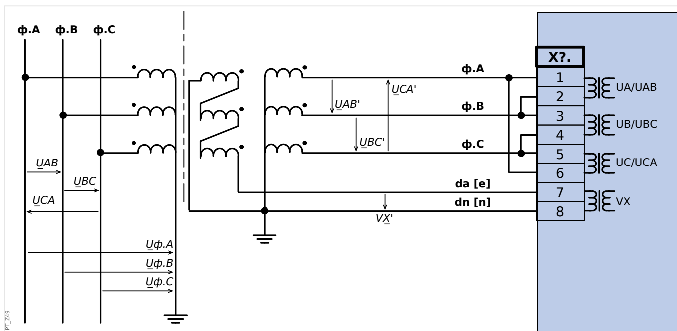
Рис. 33: Измерение трехфазного напряжения - схема измерительных входов: "соединение треугольником" Измерение напряжения нулевой последовательности V_G через вспомогательные обмотки (e-n) («открытый треугольник»)
