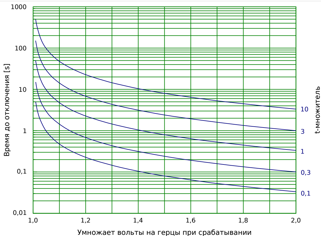
Рис. 88: Характеристика/форма кривой: INV A
