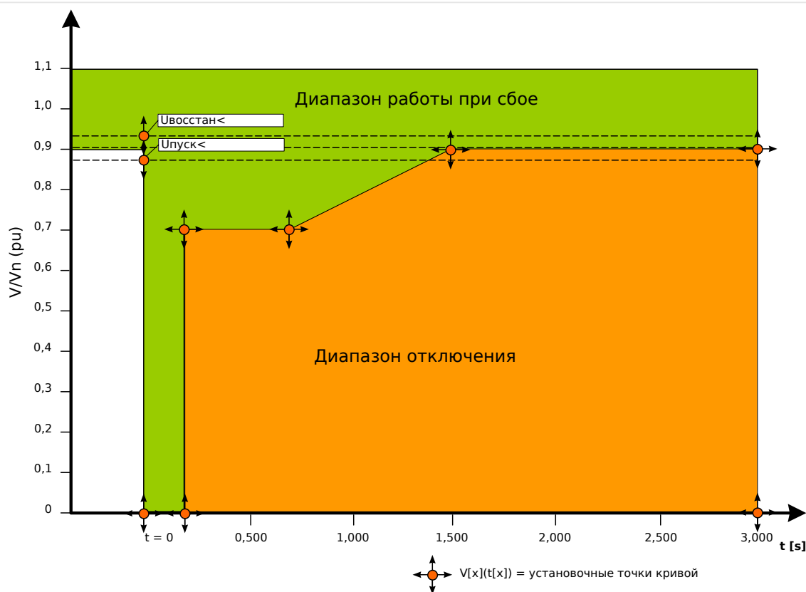
Рис. 127: Область продолжения работы и область отключения.
