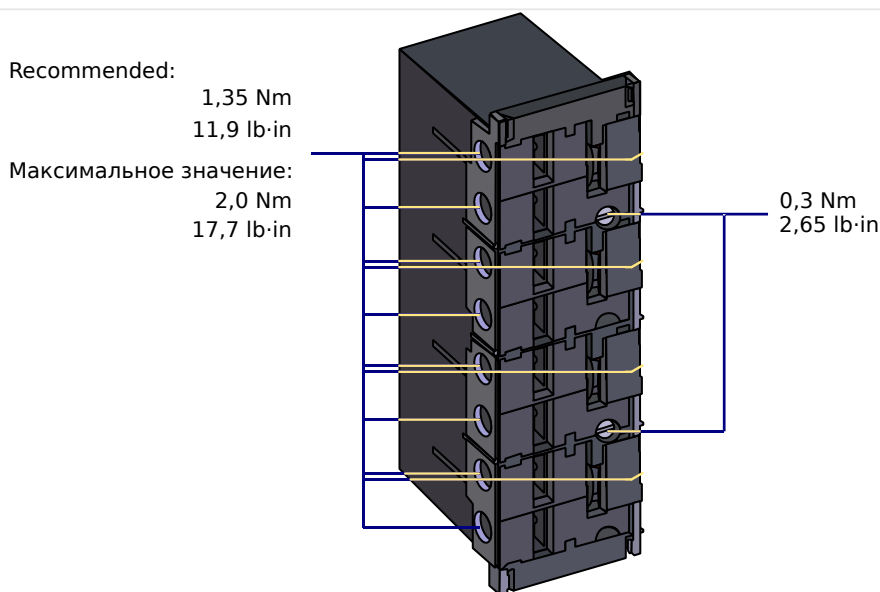
Рис. 153: Штепсельные соединения со встроенными закорачивающими перемычками (стандартные токовые входы)
