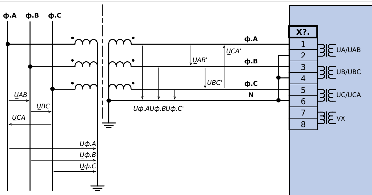
Рис. 30: VT Ууе: Измерение трехфазного напряжения по схеме «звезда»
