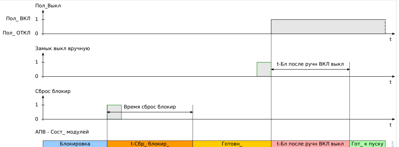
Рис. 98: Логика сброса блокировки АПВ при получении команды сброса блокировки перед замыканием выключателя вручную.
