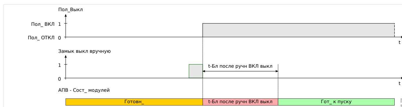
Рис. 96: Состояния автоматического повторного включения во время замыкания выключателя вручную.
