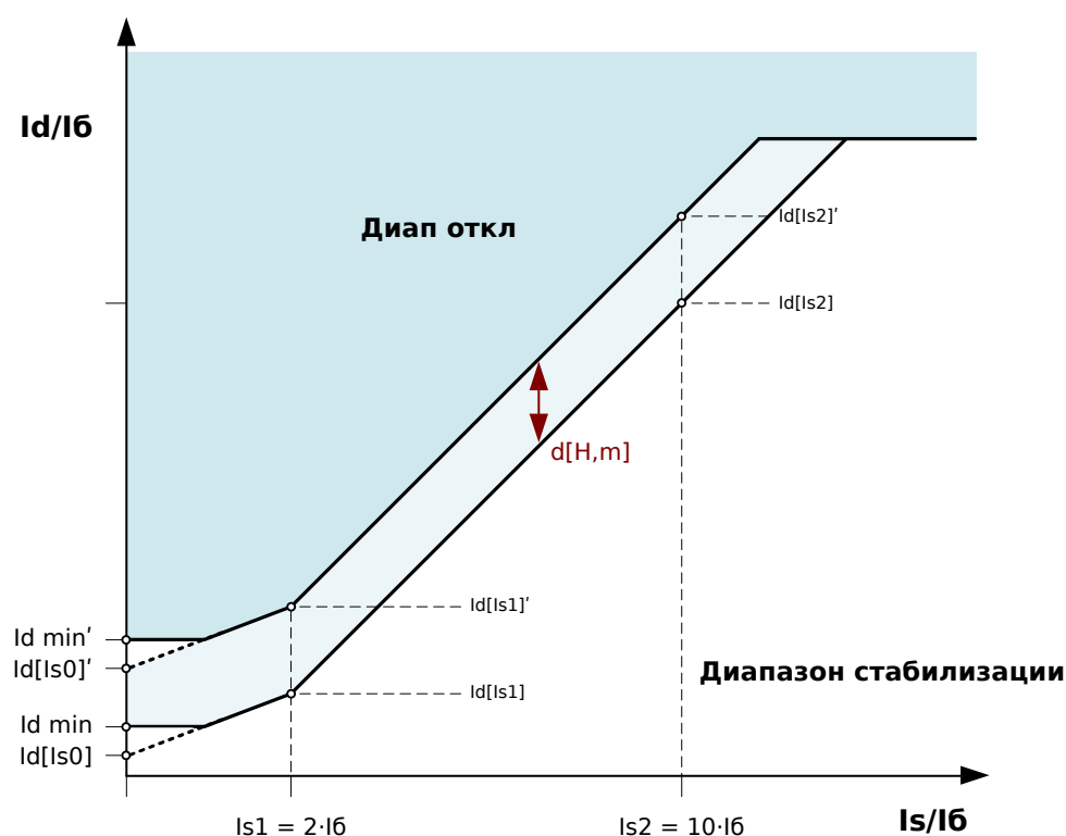
Рис. 77: Временное динамическое повышение статических характеристик отключения.
