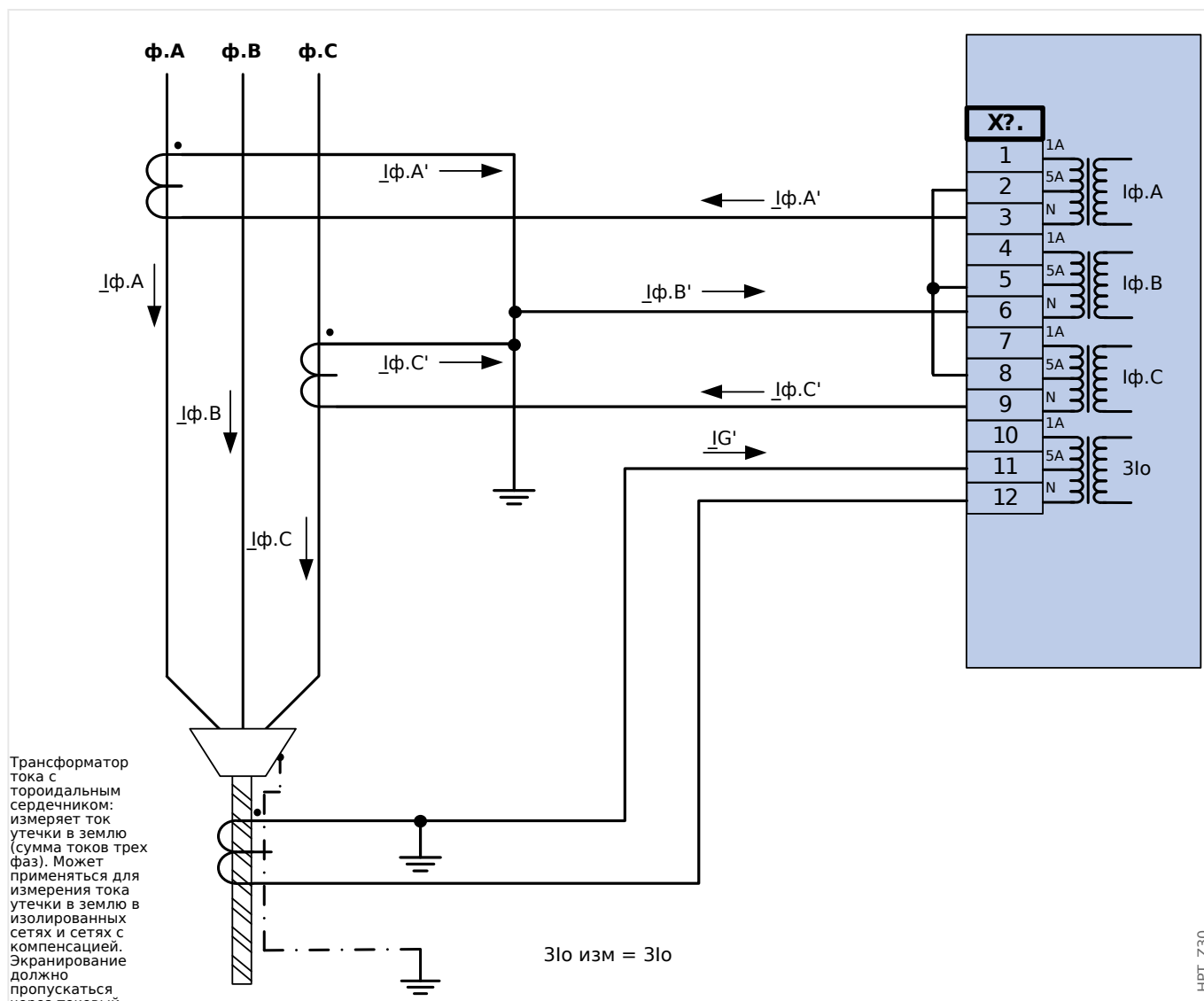
Рис. 23: Измерение двухфазного тока («соединение открытым треугольником»); I_n вторичн. = 5 A. Ток на землю, измеряемый через трансформатора тока нулевой последовательности 3I_{0.ном.втор.} = 5 A.
