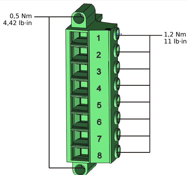
Рис. 154: Измерительные контакты платы измерения напряжения «TU» (→ «2.6.1 TU — измерительные входы напряжения»).
