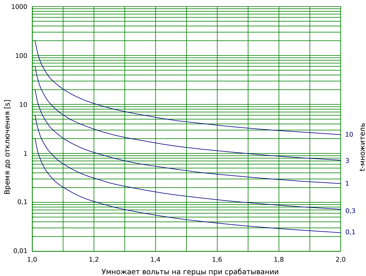
Рис. 90: Характеристика/форма кривой: INV C
