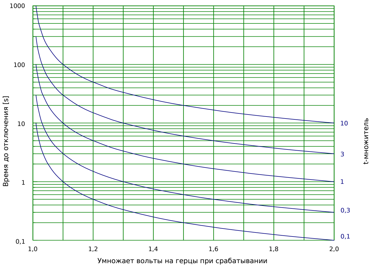
Рис. 89: Характеристика/форма кривой: INV B
