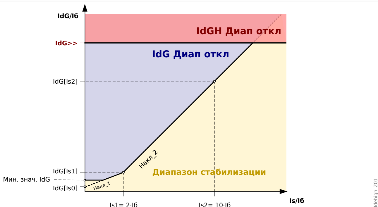
Рис. 81: Значение срабатывания « I_{dG}>> » по дифференциальному току утечки на землю, основанное на номинальной величине тока « I_6 » соответствующего объекта защиты.
