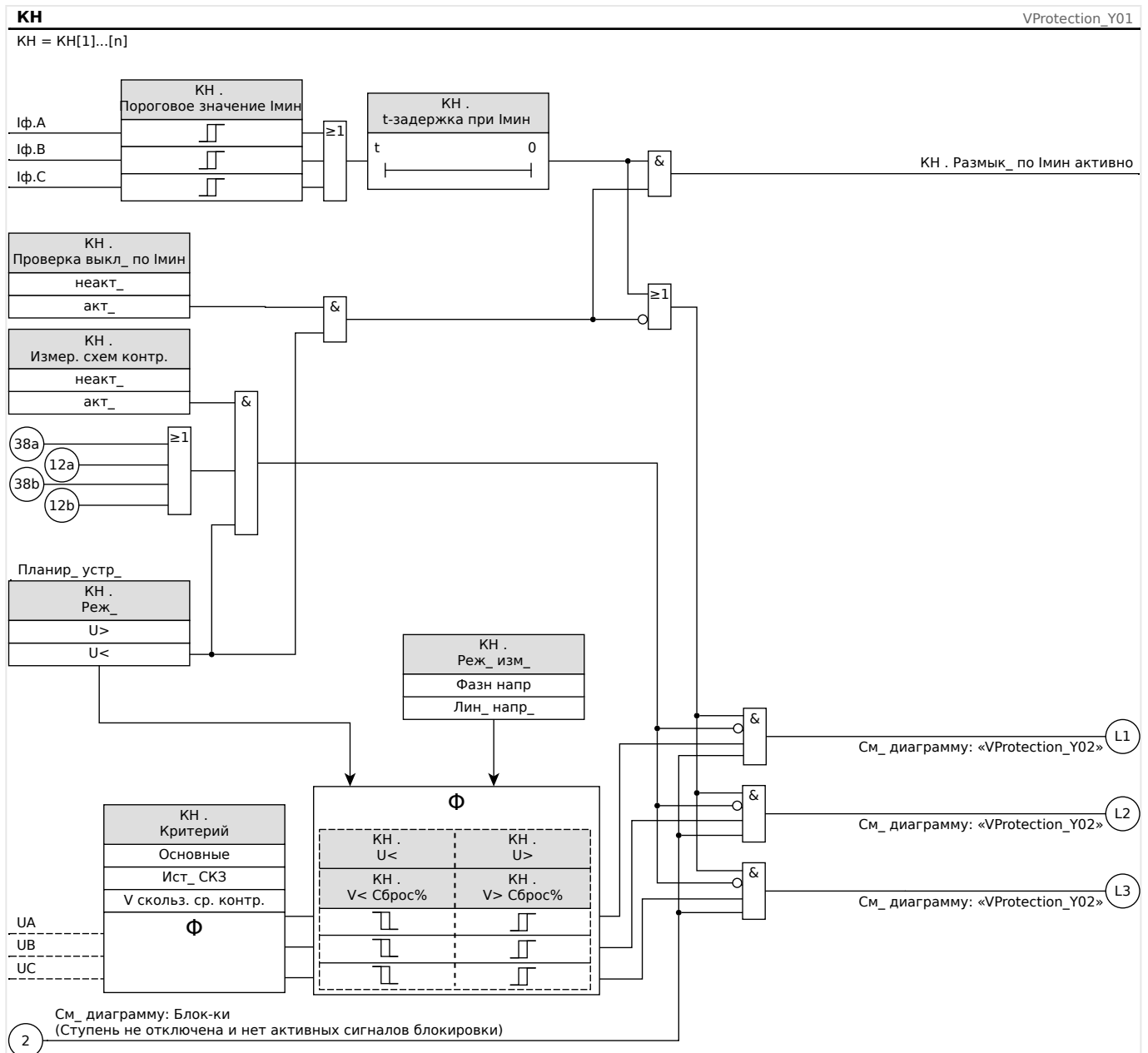
Рис. 100: Функциональные возможности модуля защиты по напряжению, часть 1.
