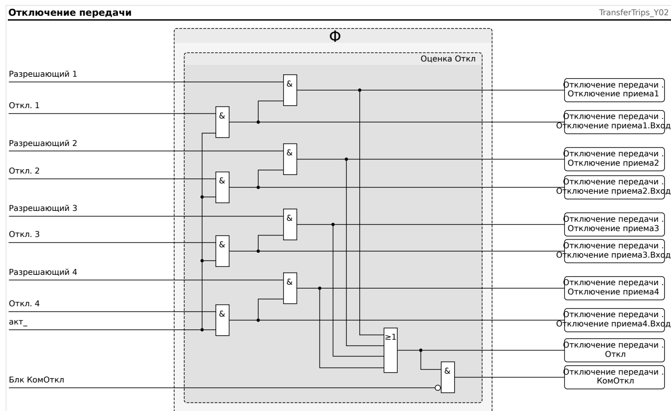
Рис. 83: Функциональные возможности модуля «Отключение передачи» (часть 2).
