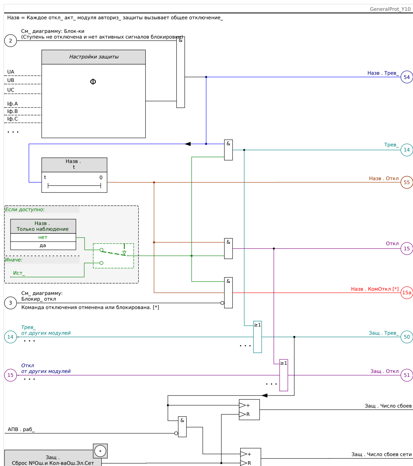
Рис. 63: Примерная схема функций любого элемента защиты HighPROTEC.
