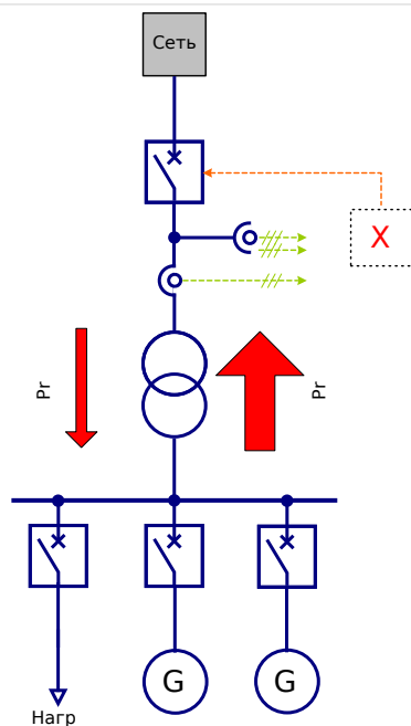
Рис. 121: Централизованное использование в сетях с преобладанием энергоснабжения.
