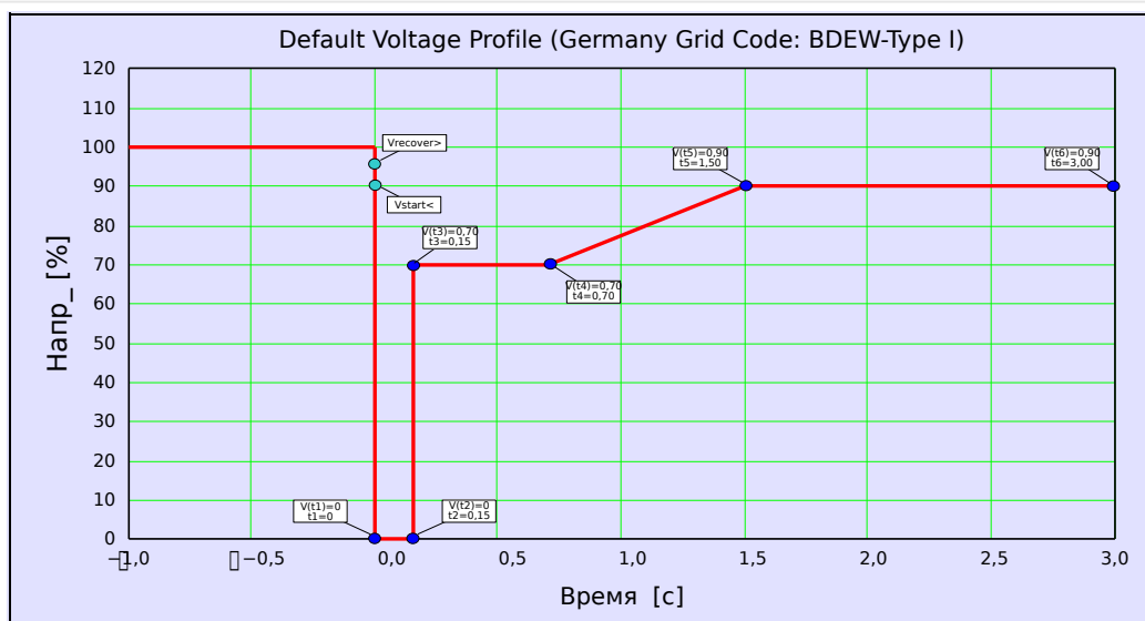
Рис. 128: Профиль LVRT по умолчанию (BDEW, тип I).
