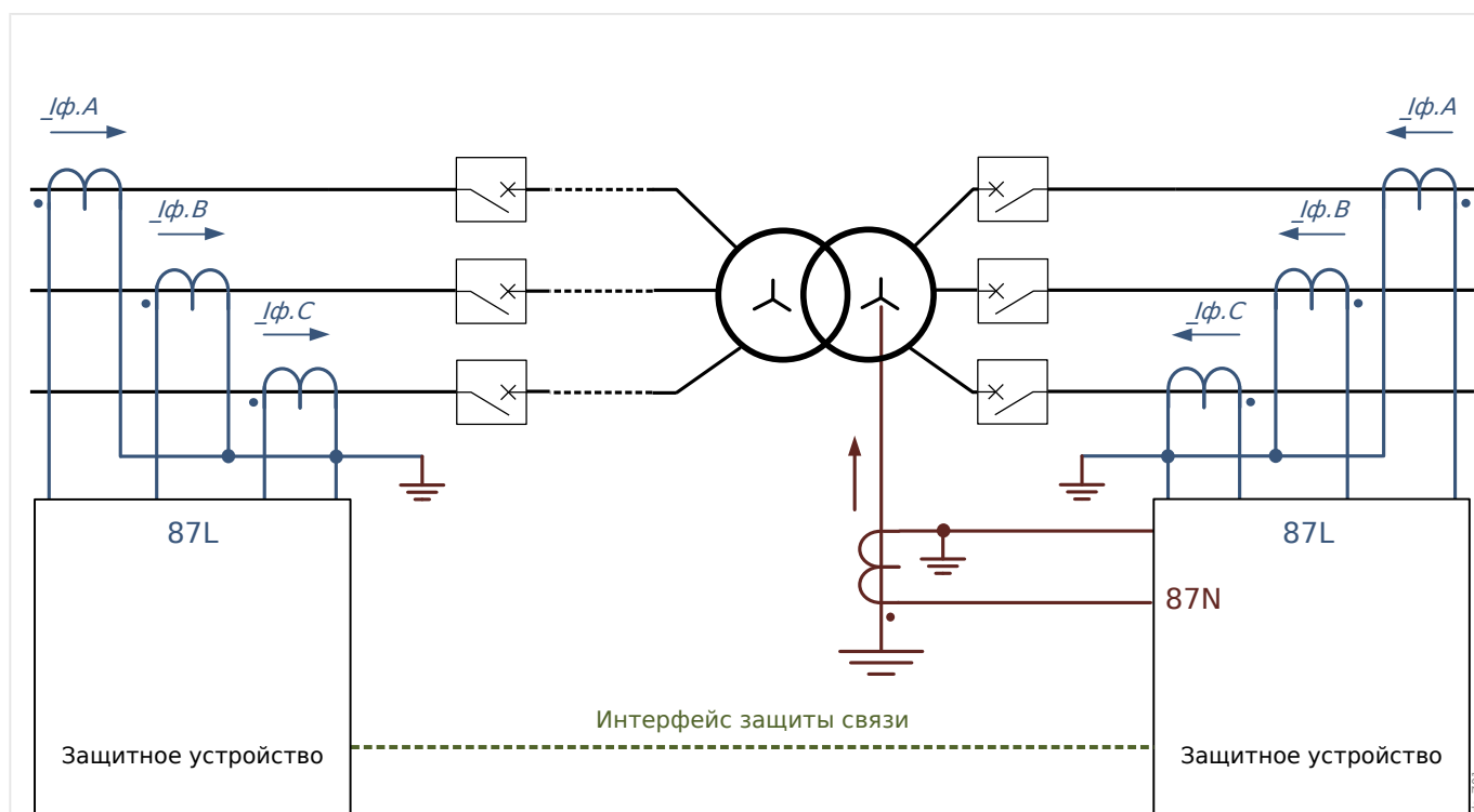
Рис. 80: Принцип работы дифференциальной защиты от тока замыкания на землю.
