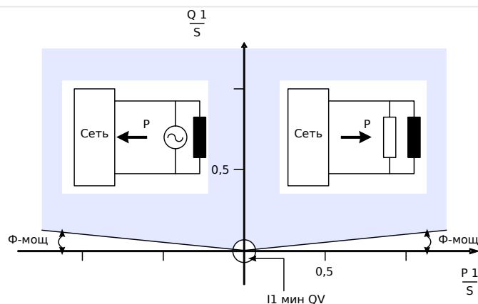
Рис. 115: Метод 1: контроль угла мощности.
