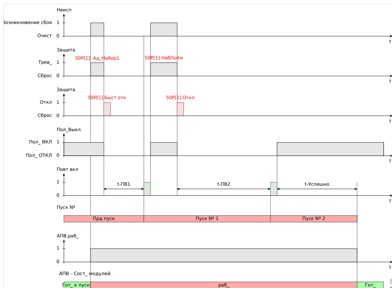
Рис. 95: Диаграмма синхронизации автоматического повторного включения для схемы с 2 удачными попытками автоматического повторного включения и ускорением перед импульсом.
