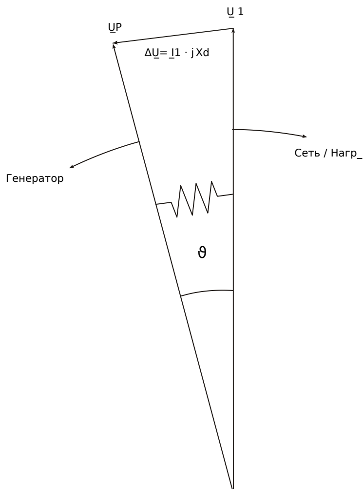
Рис. 105: Векторы напряжения в параллельной работе с электросетью.
