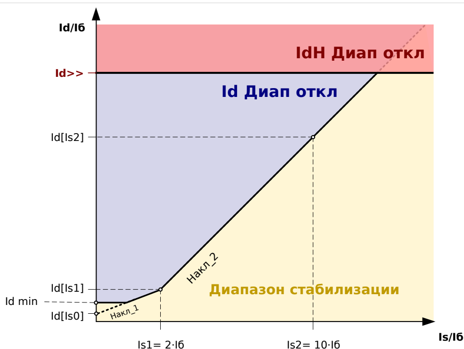
Рис. 76: Кривые отключения защитных функций «Id» (область синего цвета) и «IdH» (область красного цвета).
