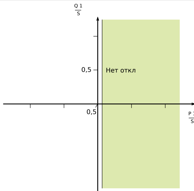
Рис. 124: Метод 2 (контроль чистой реактивной мощности): «Метод UFLS» = «Контр. чистой активной мощности».
