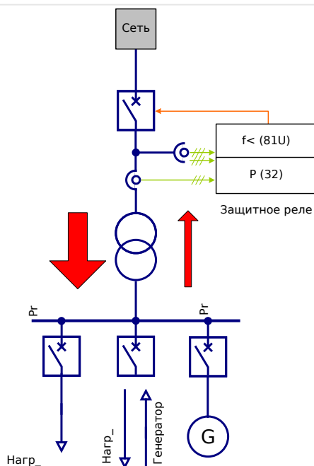
Рис. 119: Централизованная автоматическая частотная разгрузка в сетях с временным электроснабжением
