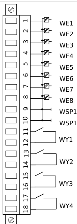
Rys. 37: Przypisanie elektromechaniczne
