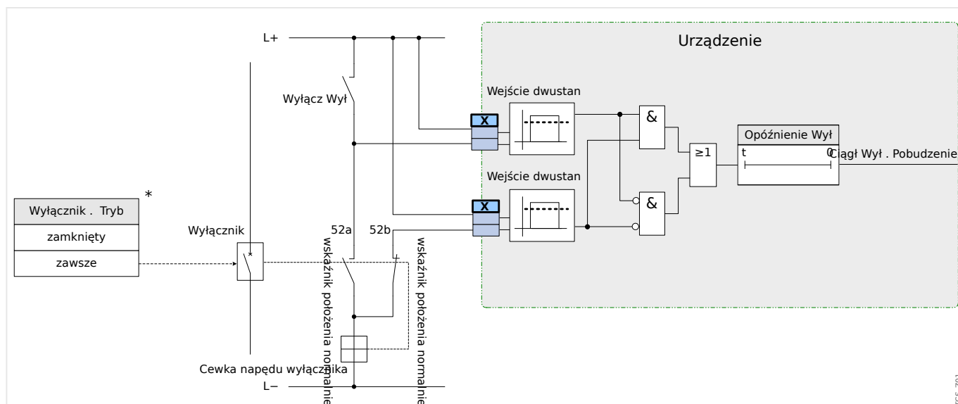
Rys. 115: Przykład okablowania: Układ kontroli ciągłości obwodów wyłącznika z dwoma stykami pomocniczymi wyłącznika „Położ ZAŁ” (52a) i „Położ WYŁ” (52b).
