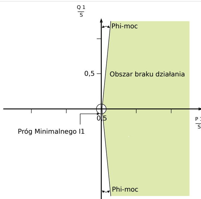
Rys. 99: Metoda 1 (kontrola kąta obciążenia): „Metoda UFLS” = „Nadzór kąta obciążenia”.
