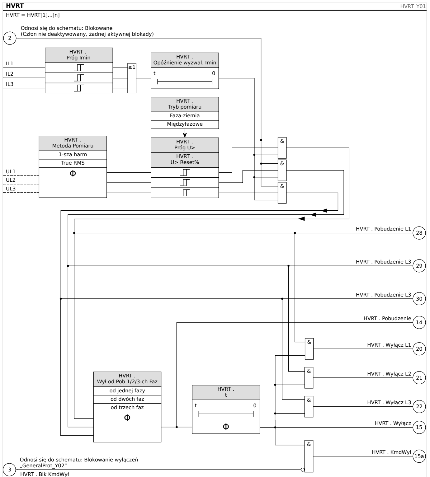
Rys. 76: Działanie zabezpieczenia HVRT.
