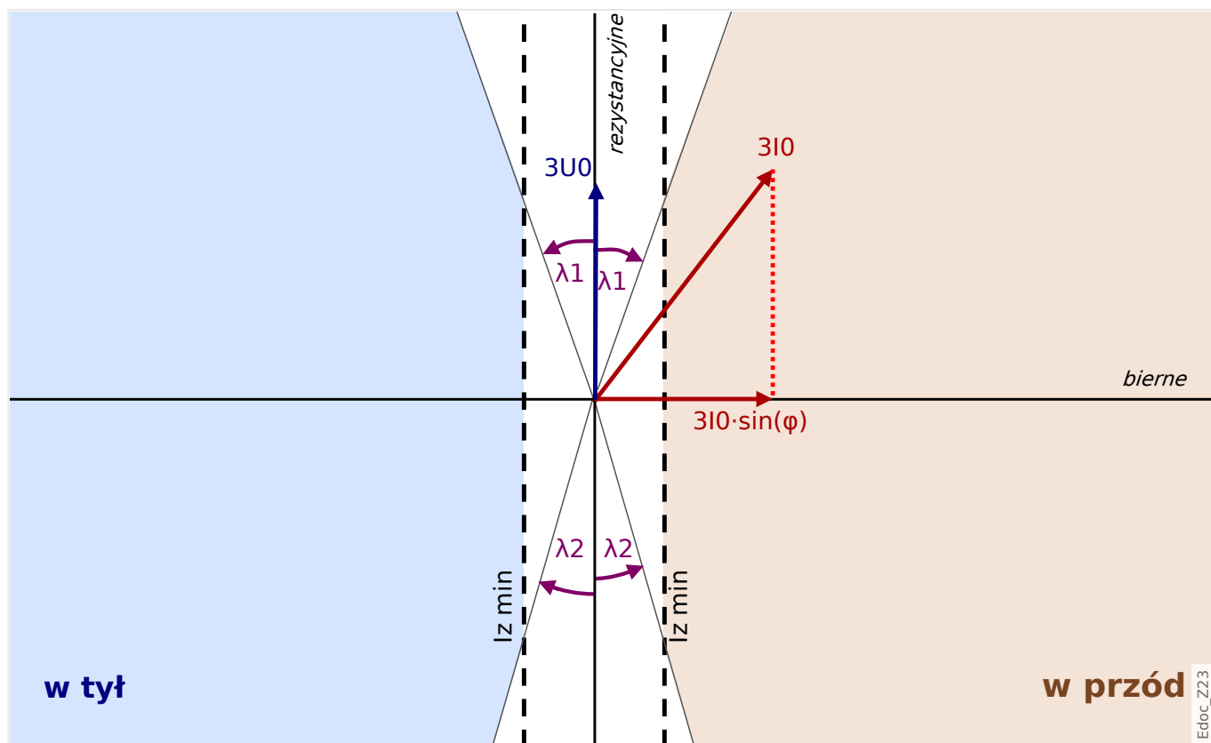
Rys. 67: Zasada określania kierunku metodą „sin(φ)”.
