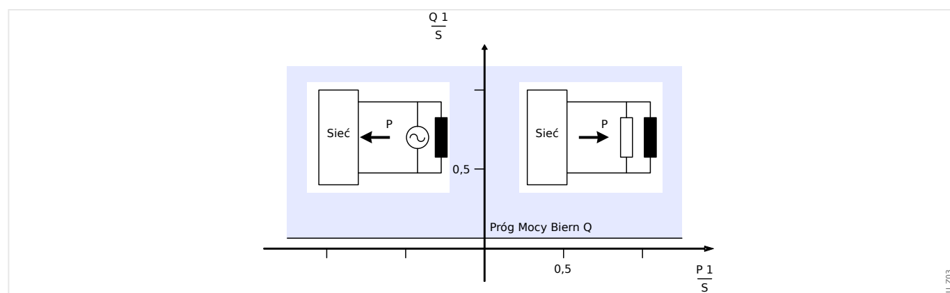
Rys. 92: Metoda 2: kontrola czystej mocy biernej.
