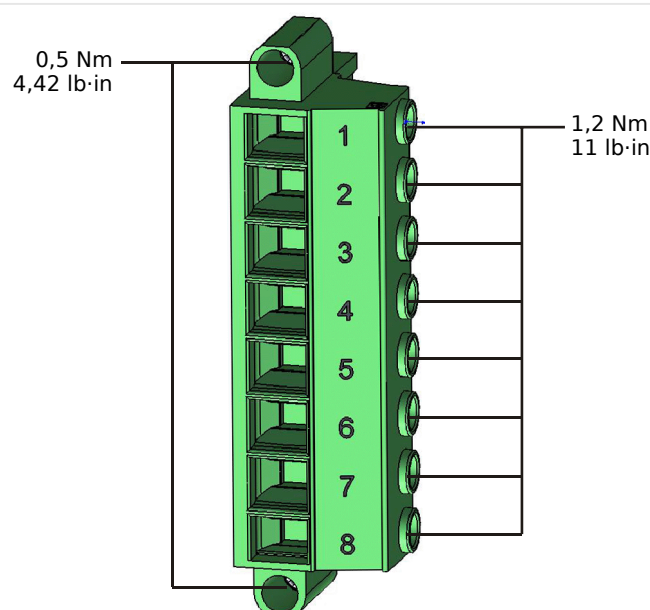
Rys. 138: Zaciski pomiaru napięcia karty pomiarowej „TU” (➡ „2.6.1 TU — wejścia do pomiaru napięcia”).
