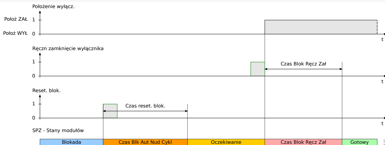
Rys. 107: Logika resetowania blokady automatyki SPZ w przypadku odebrania sygnału resetowania blokady przed ręcznym zamknięciem wyłącznika.
