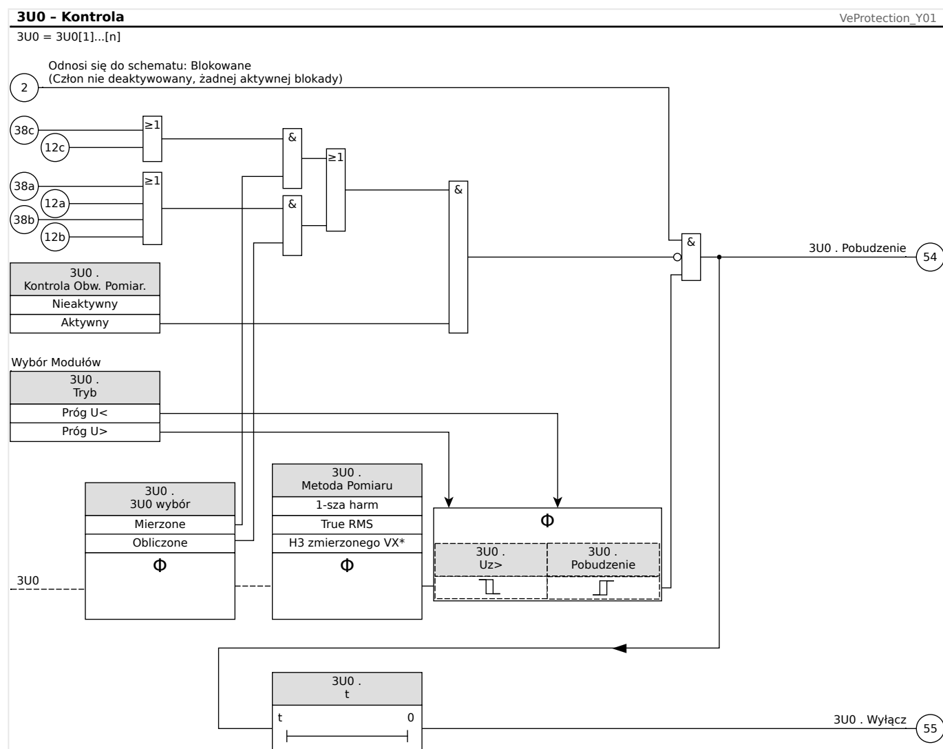
Rys. 81: Kontrola napięcia U0, UX, część 1 (funkcja kontroli, decyzja o wyzwoleniu).
