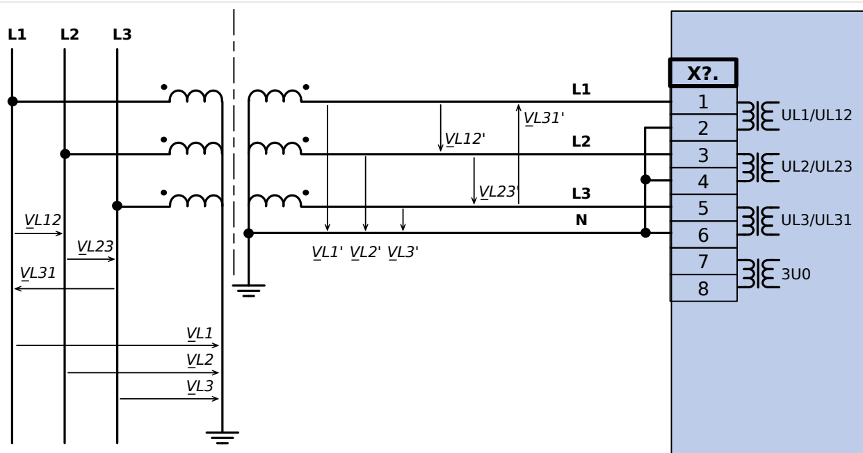
Rys. 30: Przekładnik napięciowy połączony w gwiazdę: Trójfazowy pomiar napięcia w układzie gwiazdy
