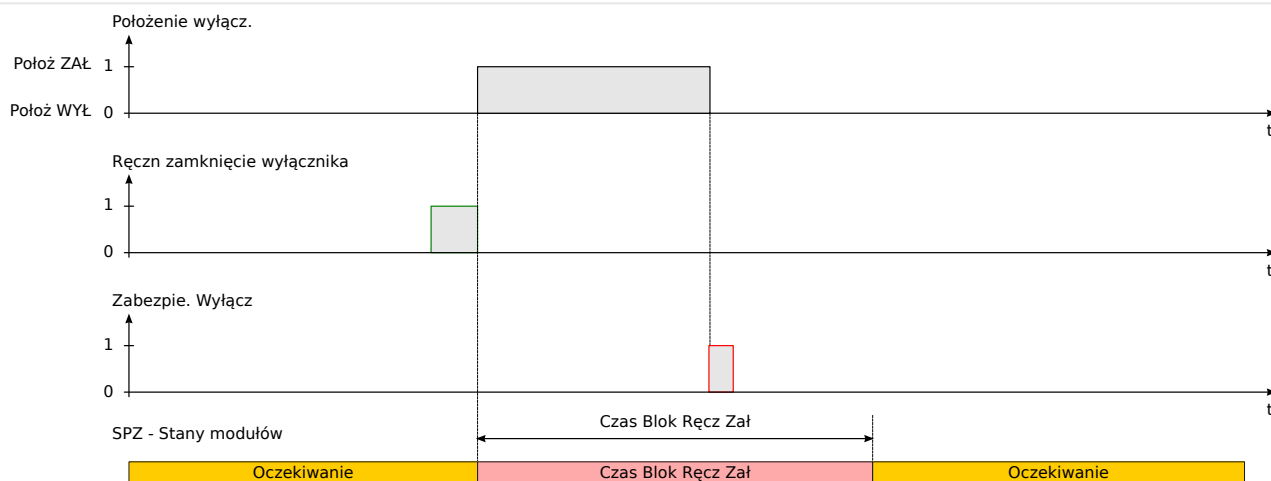
Rys. 106: Wyzwolenie zabezpieczenia podczas odliczania czasu blokady zamknięcia ręcznego.
