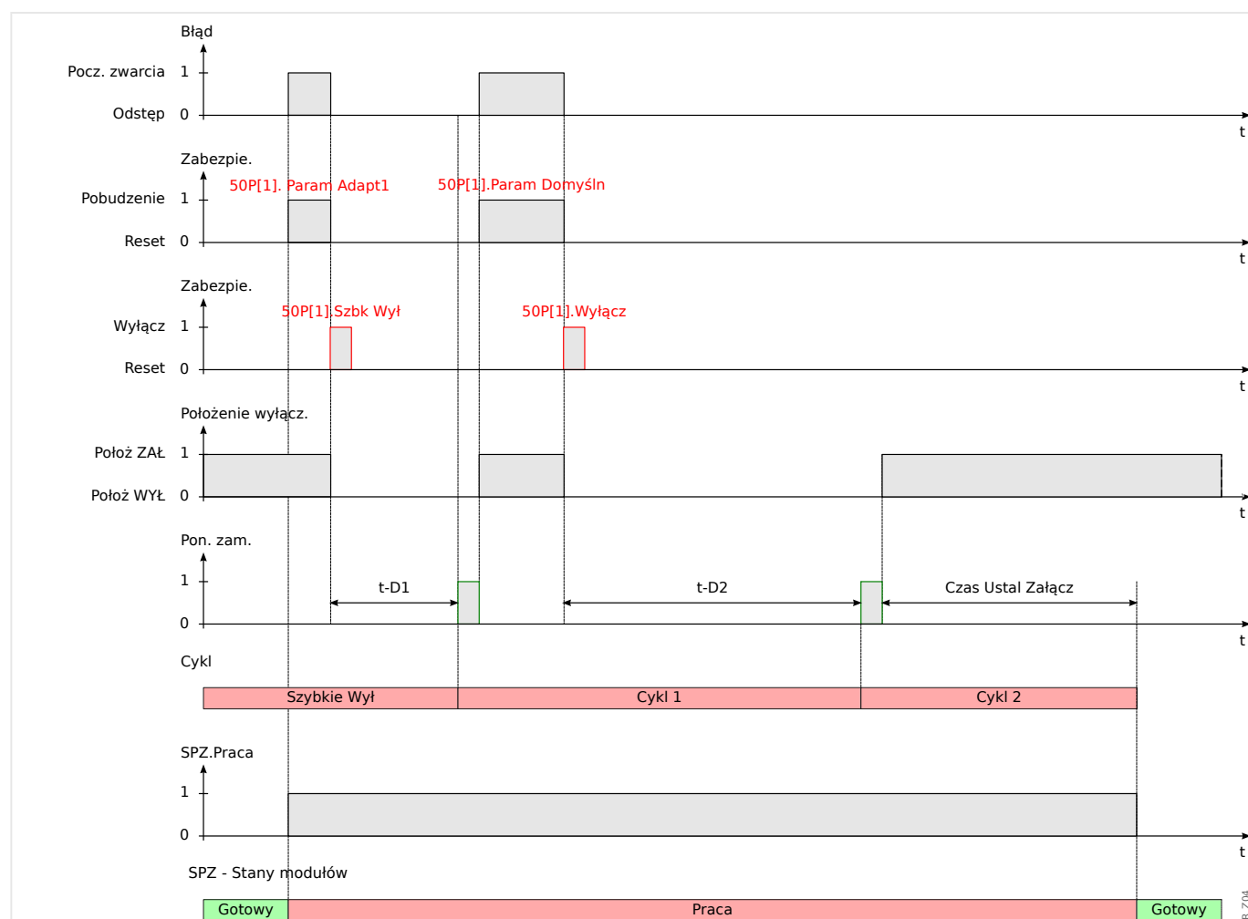
Rys. 104: Schemat czasów SPZ w przypadku udanego planu SPZ z 2 próbami i przyspieszeniem przy próbie wstępnej
