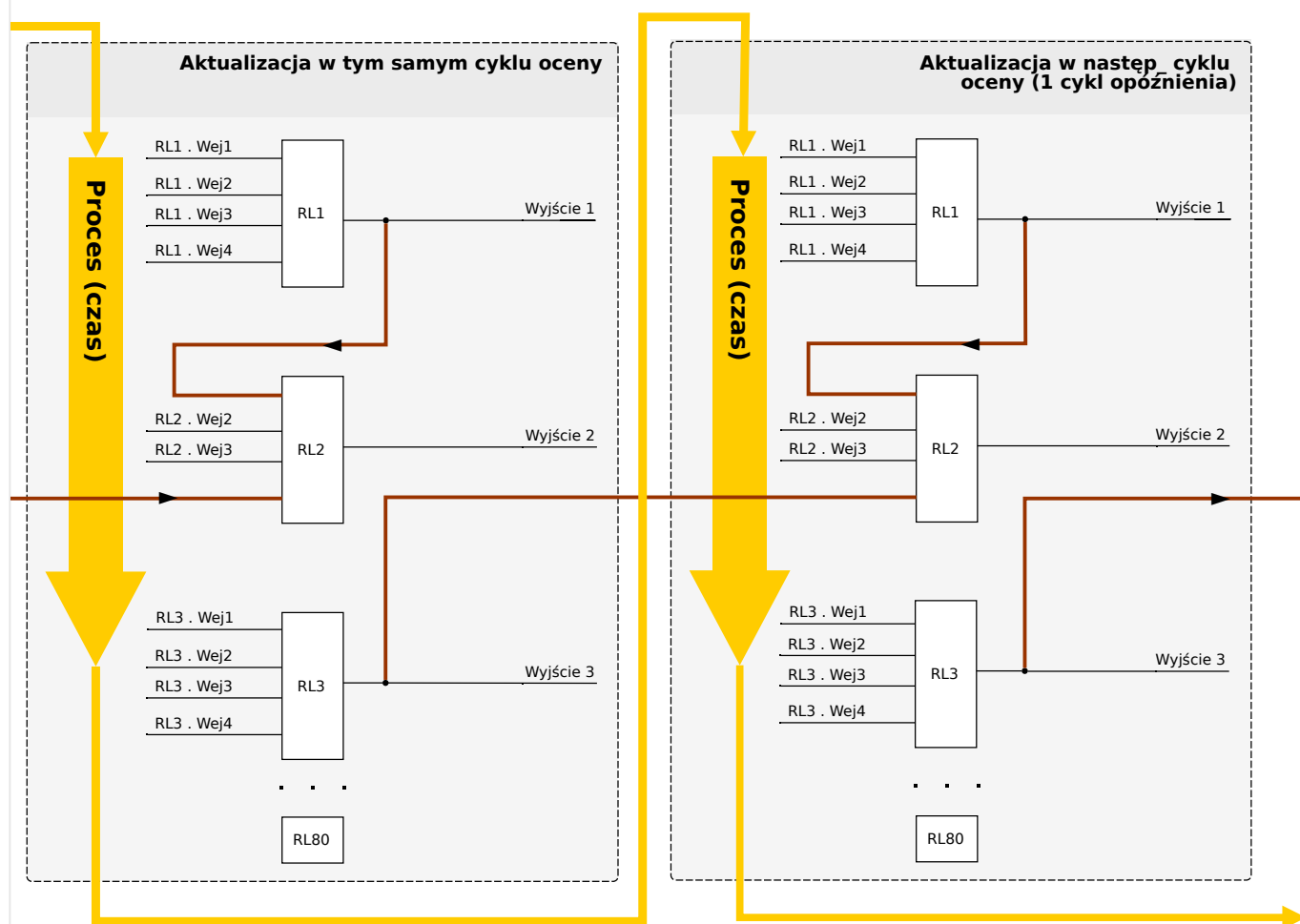
Rys. 134: Ukł. kaskadowy w porządku malejącym.
