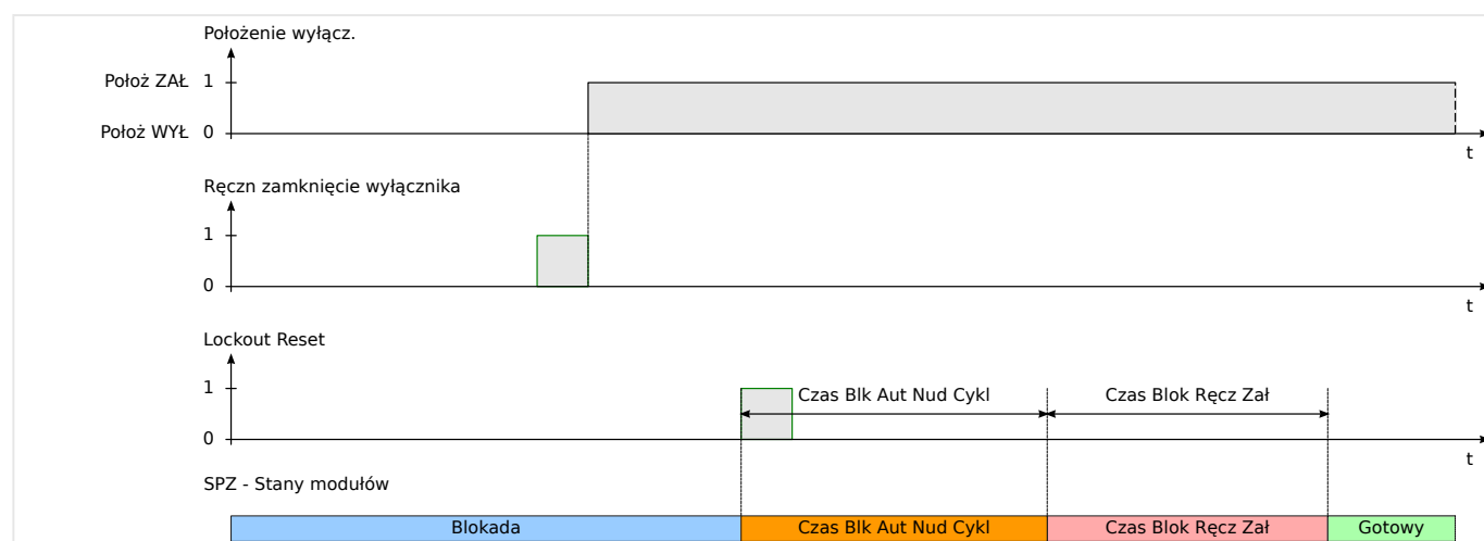
Rys. 108: Logika resetowania blokady automatyki SPZ w przypadku odebrania sygnału resetowania blokady po ręcznym zamknięciu wyłącznika.
