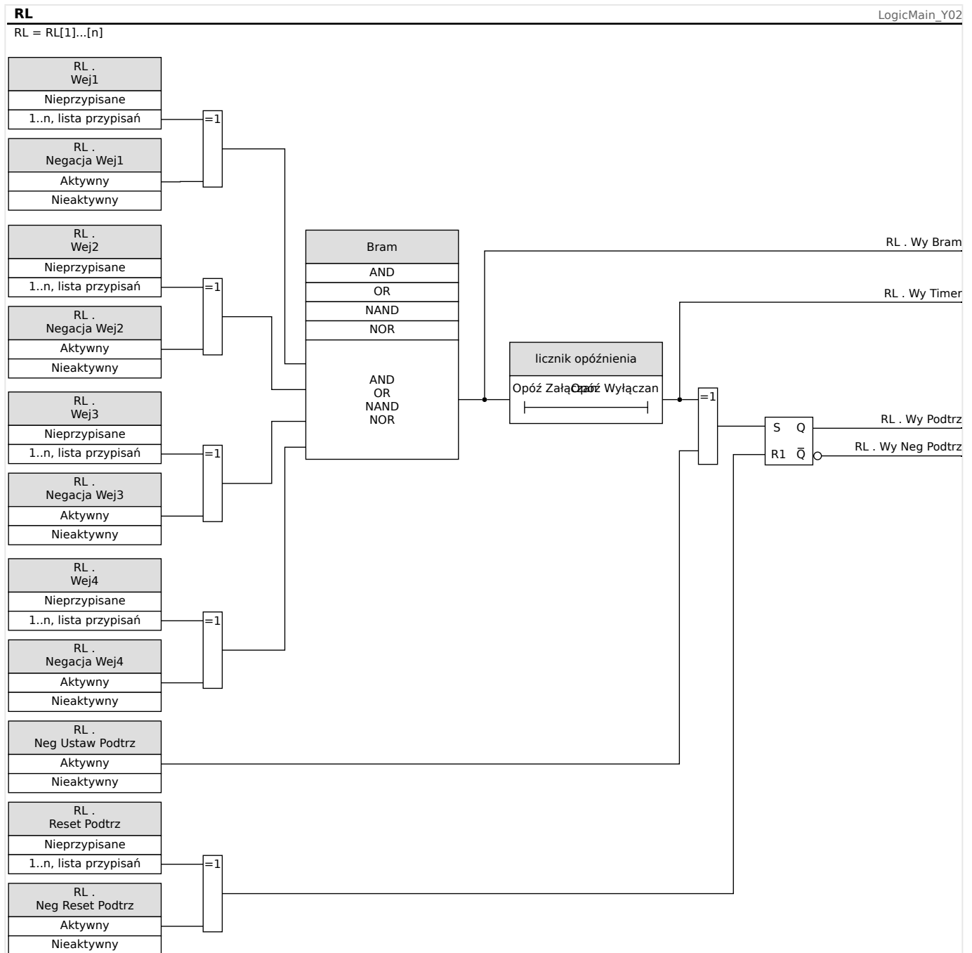
Rys. 131: Przegląd szczegółowy — ogólny schemat logiczny.
