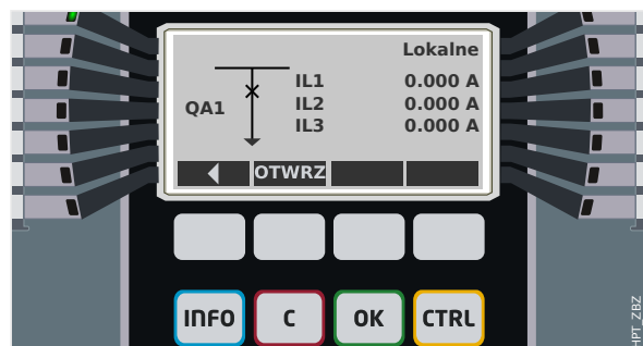
Rys. 119: Przykład strony sterowania z wyłącznikiem w pozycji zamkniętej.
