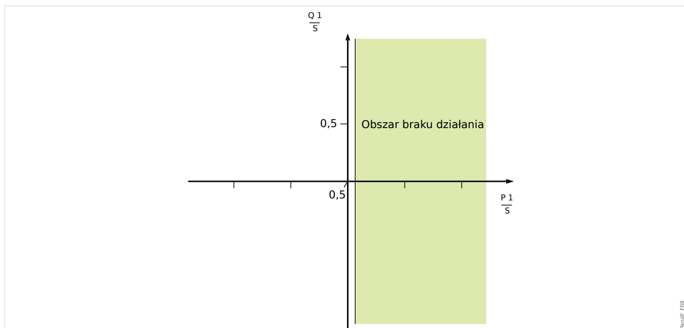
Rys. 100: Metoda 2 (kontrola czystej mocy czynnej). „Metoda UFLS” = „Nadzór Czystej Mocy Czyn”.
