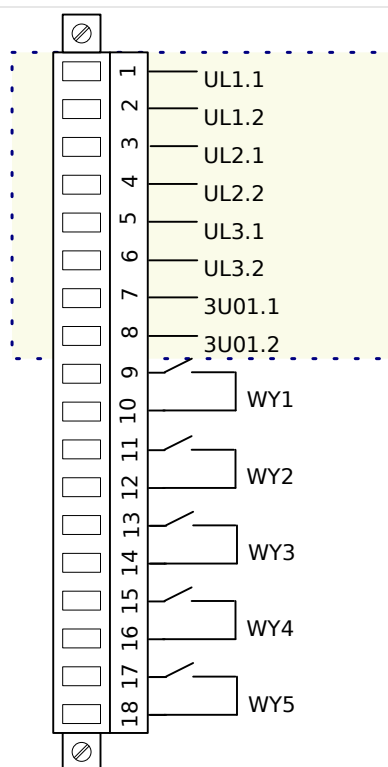
Rys. 29: Przypisanie elektromechaniczne
