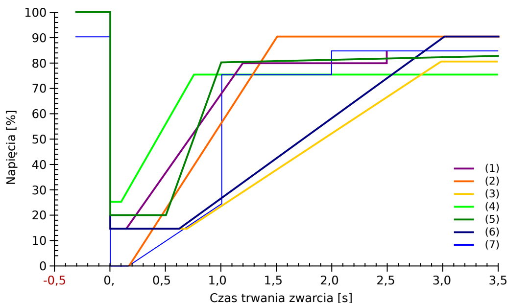
Rys. 77: Normy LVRT; źródło: eBWK Bd. 60 (2008) Nr 4. Autorzy: Dipl.-Ing. Thomas Smolka, Dr.-Ing. Karl-Heinz Weck, Zertifizierungstelle der FGH e.V., Mannheim, sowie Dipl.-Ing. (FH) Matthias Bartsch, Enercon GmbH, Aurich.
