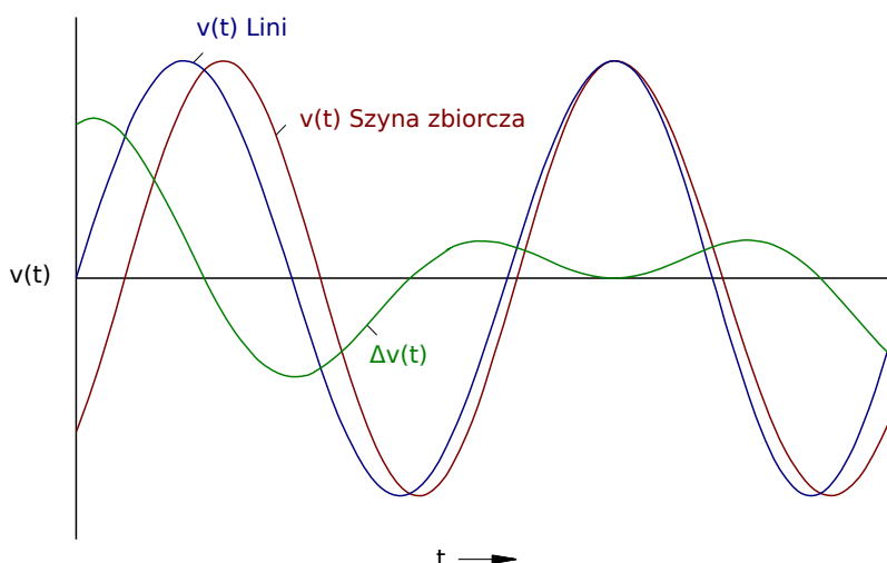
Rys. 110: Krzywa napięciowa ze zwiększoną rozdzielczością.
