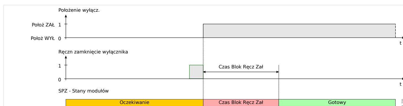
Rys. 105: Stany SPZ podczas ręcznego zamykania wyłącznika.
