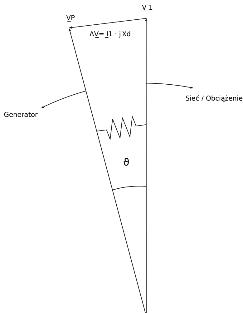
Rys. 85: Wektory napięcia przy pracy równoległej z siecią.
