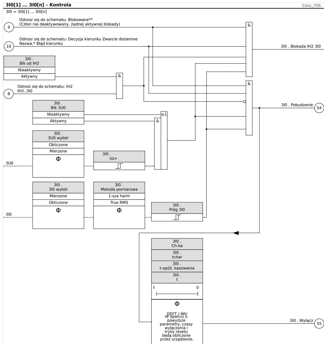
Rys. 71: Zabezpieczenie nadprądowe ziemnozwarciowe, część 1 (funkcja kontroli, decyzja o wyzwoleniu).
