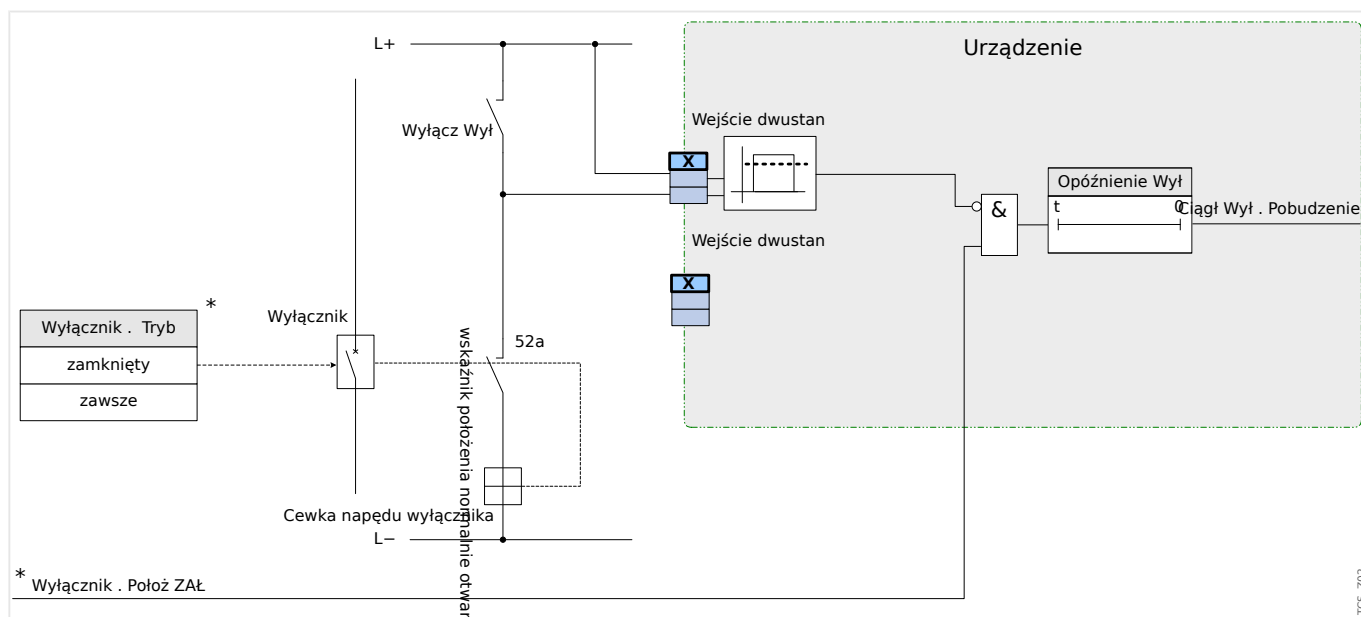
Rys. 116: Przykład okablowania: Układ kontroli ciągłości obwodów wyłącznika z tylko jednym stykiem pomocniczym wyłącznika „Położ ZAŁ” (52a).
