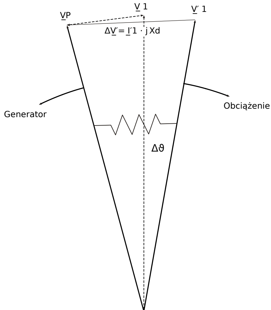
Rys. 87: Wektory napięcia przy awarii sieci.
