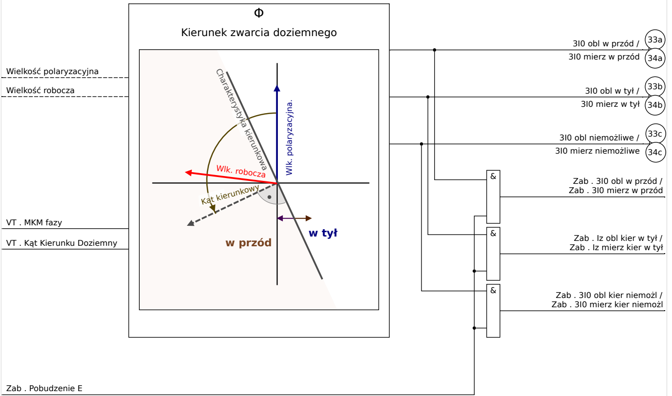
Rys. 65: Zasada określania kierunku obowiązująca dla wszystkich metod z wyjątkiem „ \cos(\phi) ”, „ \sin(\phi) ”.
