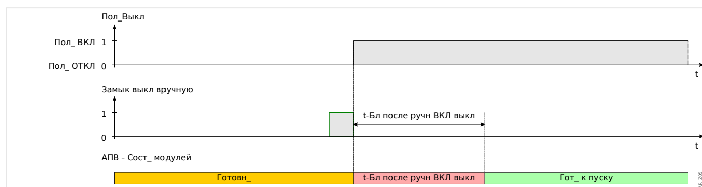
Рис. 105: Состояния автоматического повторного включения во время замыкания выключателя вручную.
