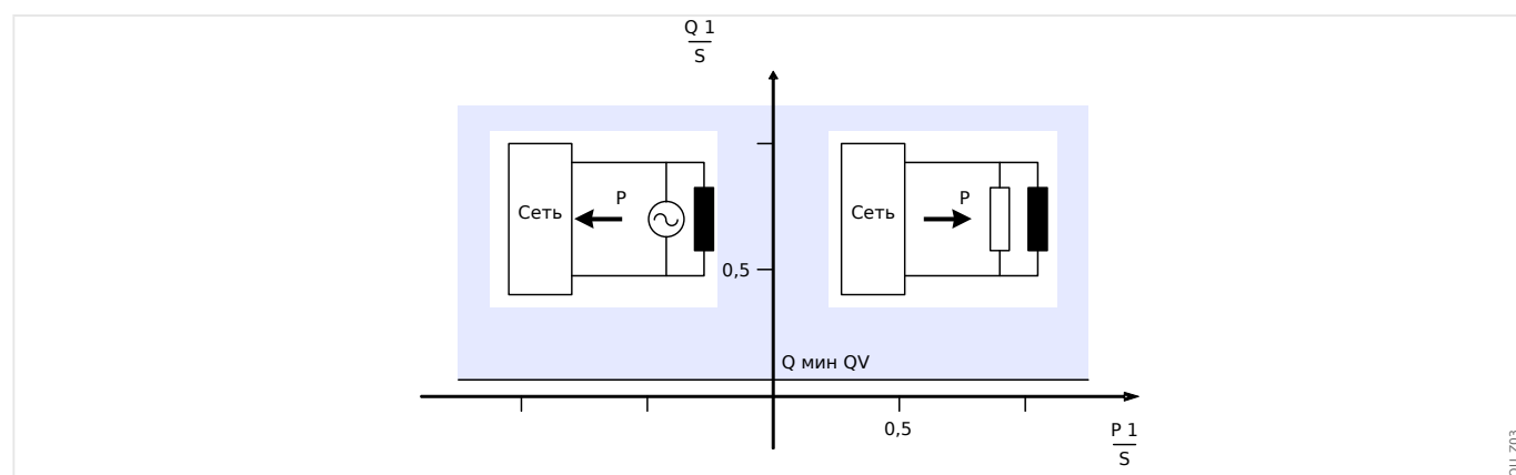
Рис. 92: Метод 2: контроль чистой реактивной мощности.
