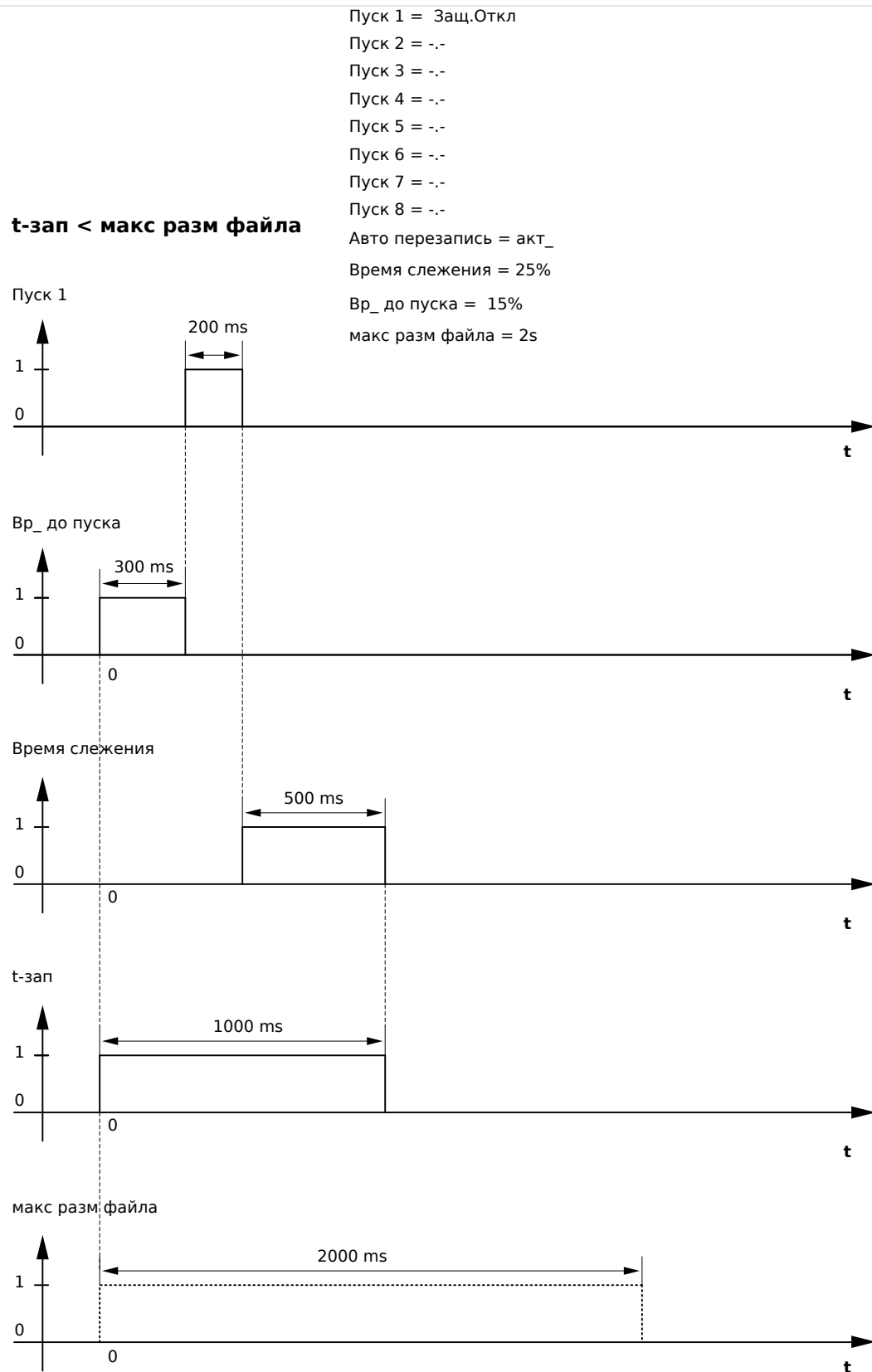
Рис. 128: Пример временной диаграммы регистратора аварийных нарушений II
