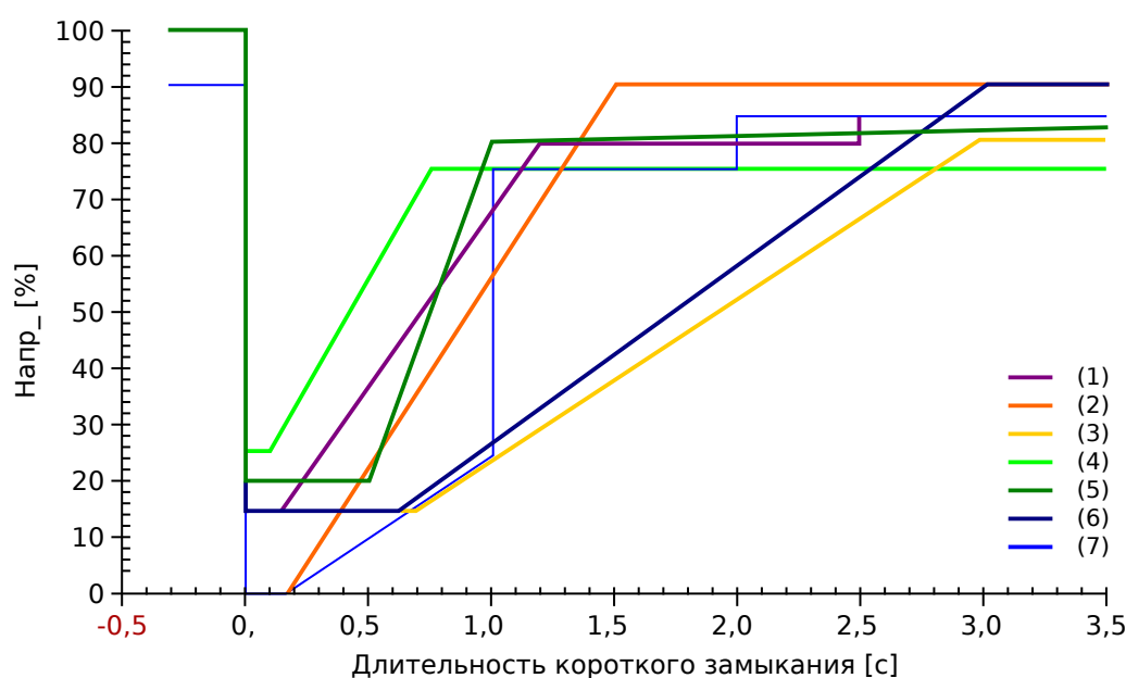
Рис. 77: Стандарты РПН; источник: eBWK Bd. 60 (2008 г.), № 4. Авторы: дипломированный инженер Томас Смолка, д. т. н. Карл-Хайнц Век, центр сертификации FGH e.V., Мангейм, а также дипломированный инженер (FH) Матиас Барч, Enercon GmbH, Аурих.
