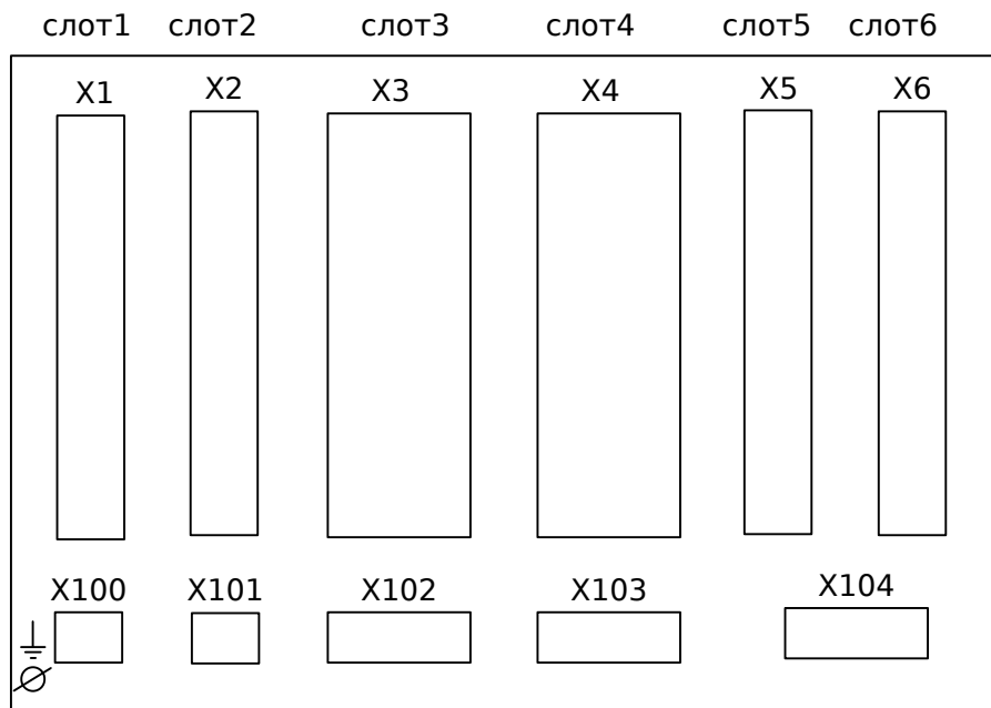
Рис. 7: Корпус В2 — принципиальная схема
