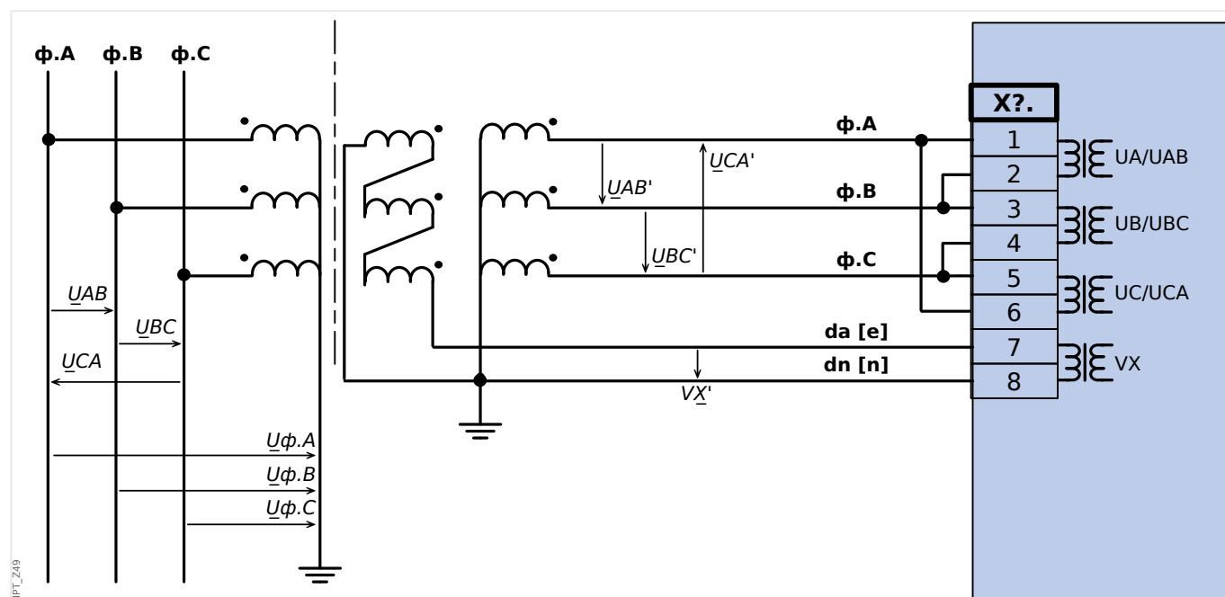
Рис. 33: Измерение трехфазного напряжения - схема измерительных входов: "соединение треугольником" Измерение напряжения нулевой последовательности \underline{V}_G через вспомогательные обмотки (e-n) («открытый треугольник»)
