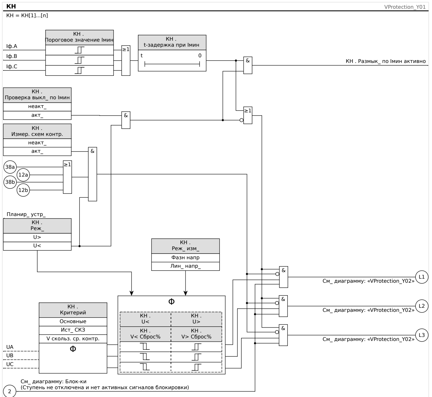
Рис. 74: Функциональные возможности модуля защиты по напряжению, часть 1.
