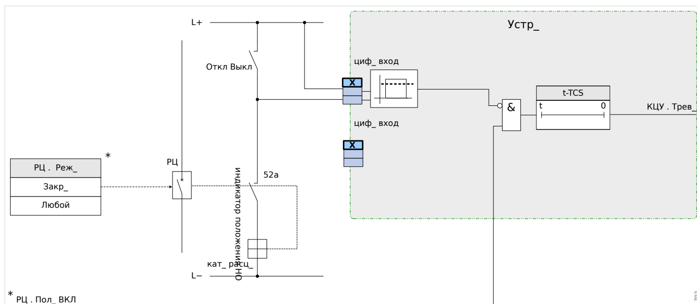
Рис. 59: Пример соединения: контроль цепи отключения только с одним вспомогательным контактом выключателя «Всп Вкл» (52a).
