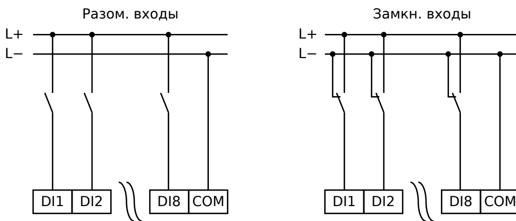
Рис. 80: Безопасное состояние цифровых входов
