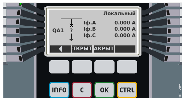
Рис. 62: Пример страницы управления, выключатель в аварийном (недопустимое состояние) положении.
