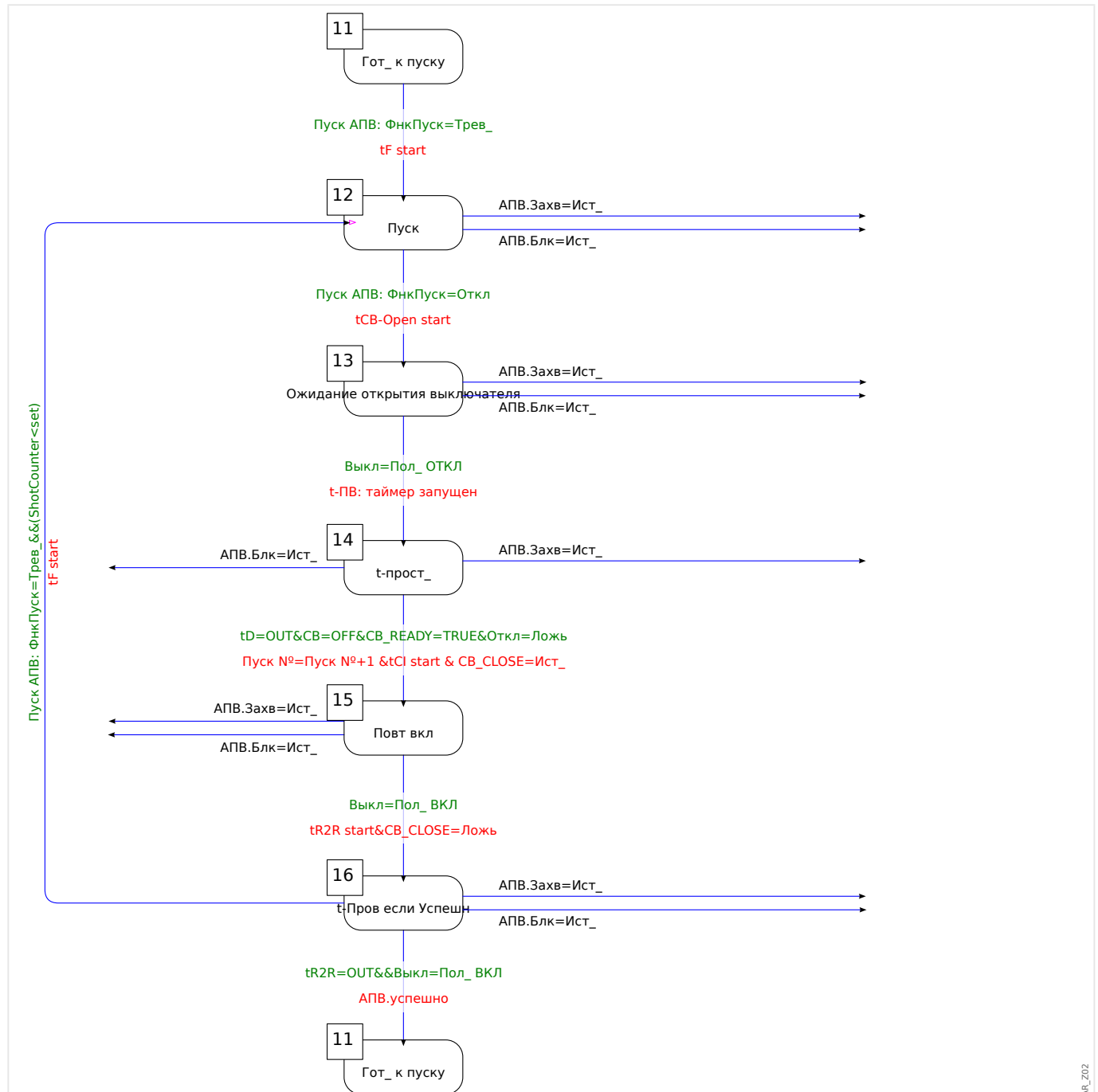
Рис. 49: Цикл выполнения АПВ (состояние 4).
