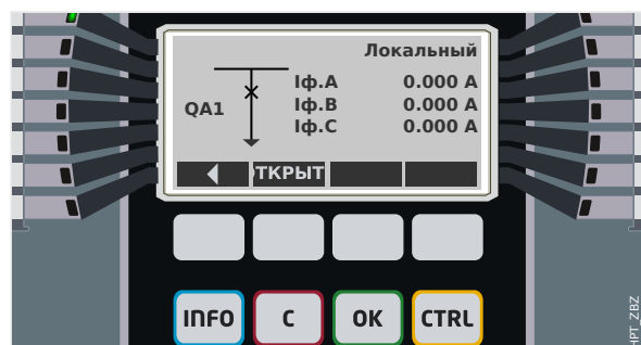
Рис. 61: Пример страницы управления, выключатель в замкнутом положении.
