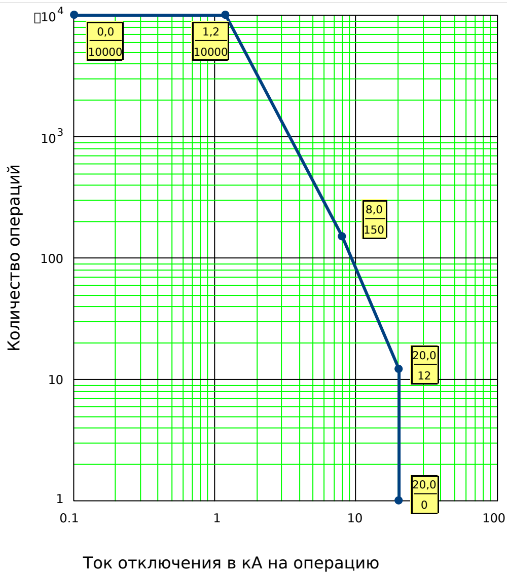
Рис. 66: Эксплуатационная кривая выключателя для типичного выключателя 25кВ
