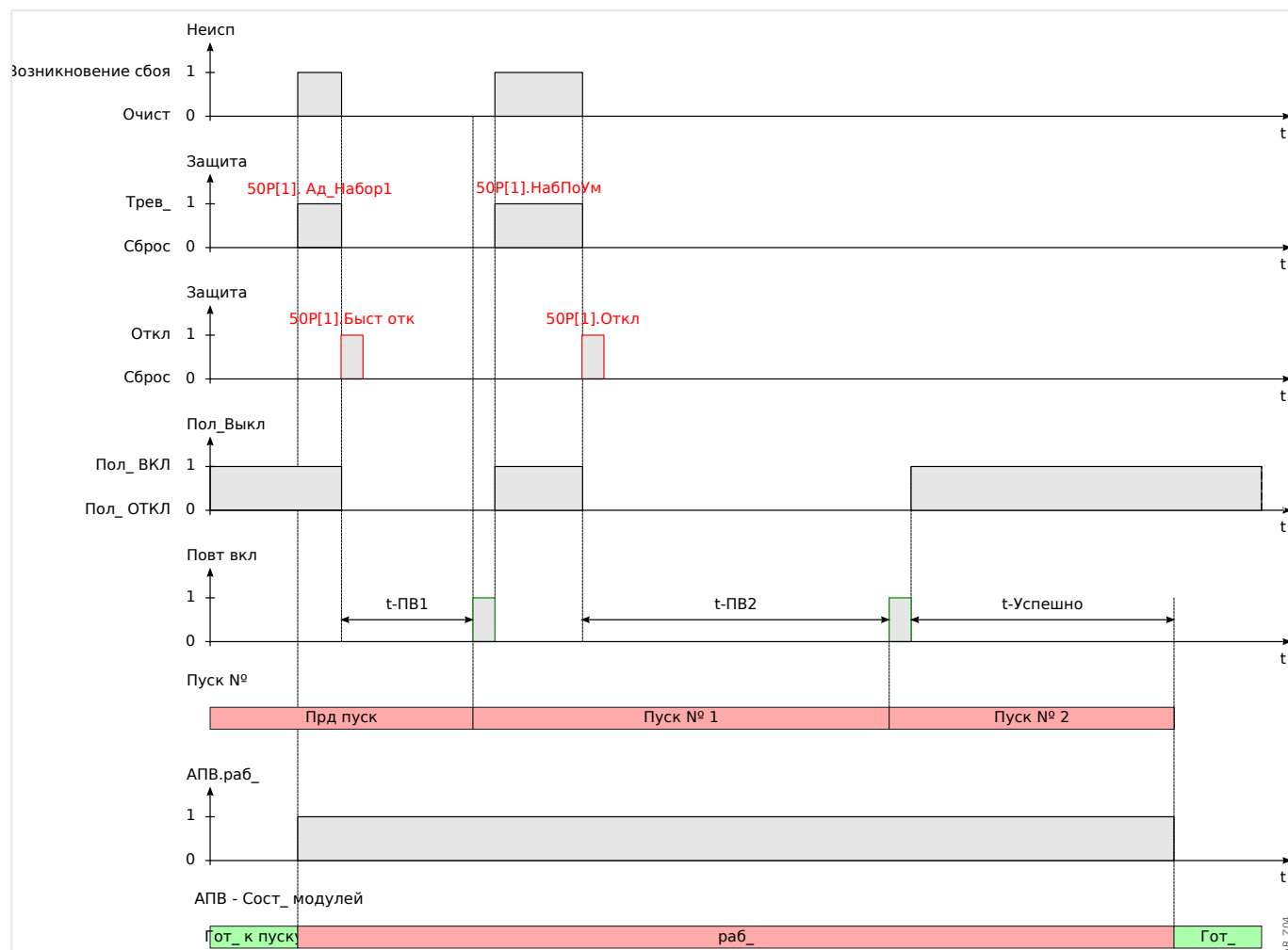
Рис. 51: Диаграмма синхронизации автоматического повторного включения для схемы с 2 удачными попытками автоматического повторного включения и ускорением перед импульсом.
