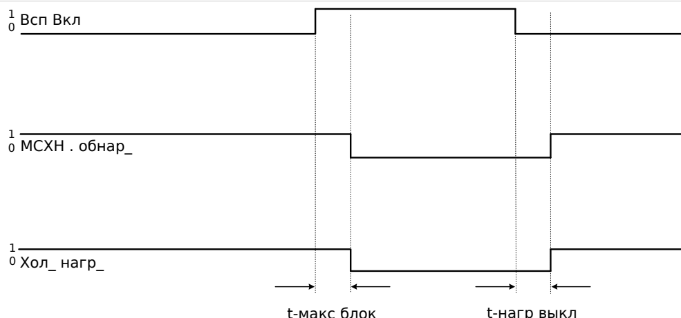
Рис. 56: Пример: Положение выключателя.
