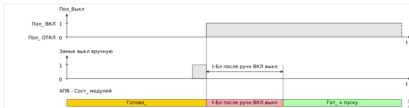
Рис. 52: Состояния автоматического повторного включения во время замыкания выключателя вручную.
