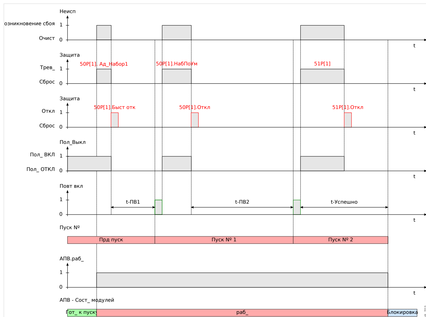
Рис. 50: Диаграмма синхронизации автоматического повторного включения для схемы с 2 неудачными попытками автоматического повторного включения и ускорением перед импульсом.
