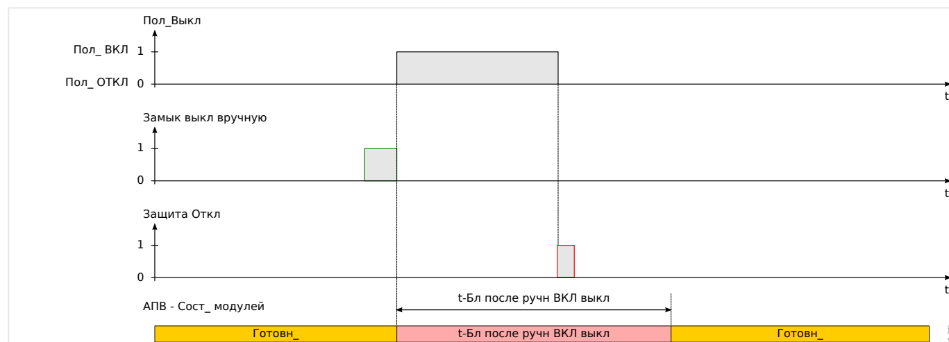
Рис. 53: Отключение защиты во время работы таймера блокировки замыкания вручную.
