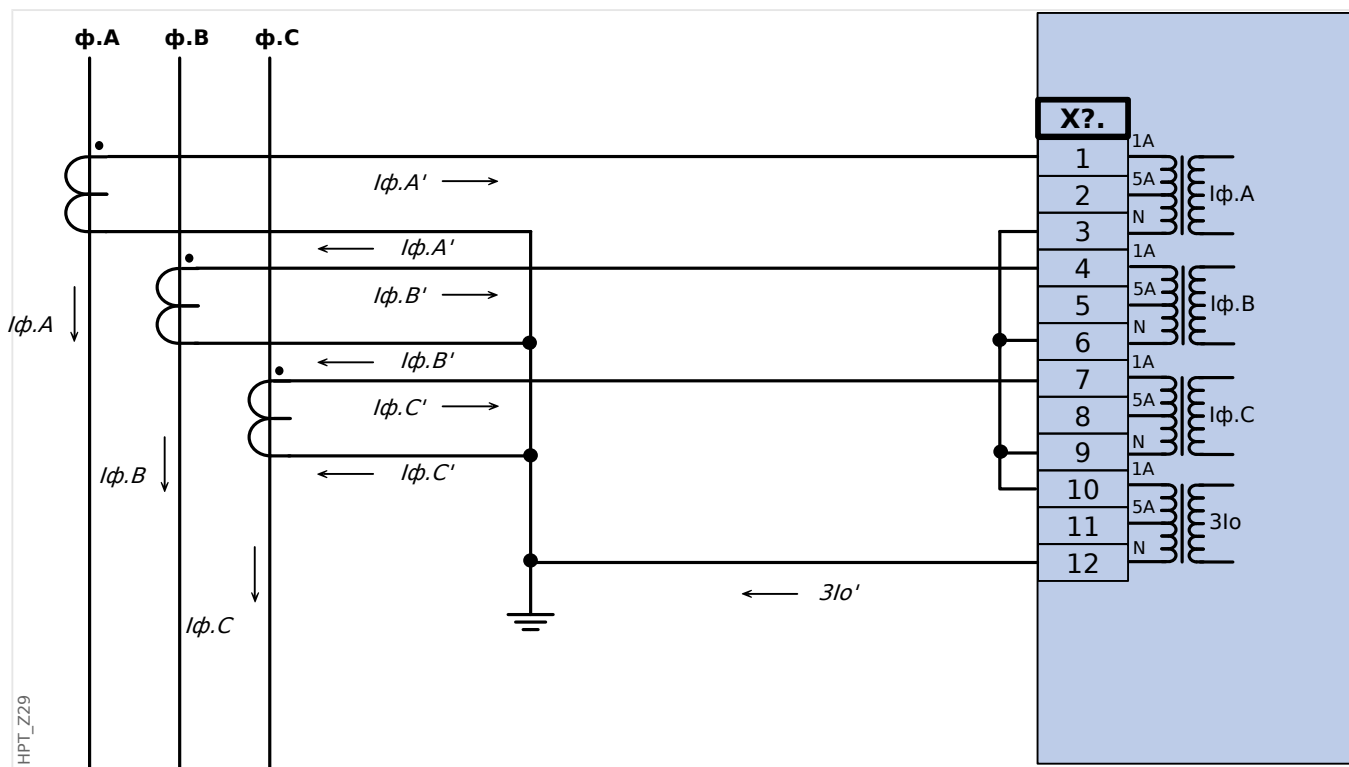
Рис. 22: Измерение фазных токов по схеме «полной» звезды; I_n вторичн. = 1 А. Ток на землю, измеряемый через соединение по схеме Холмгрин 3I_o .ном.втор. = 1 А.
