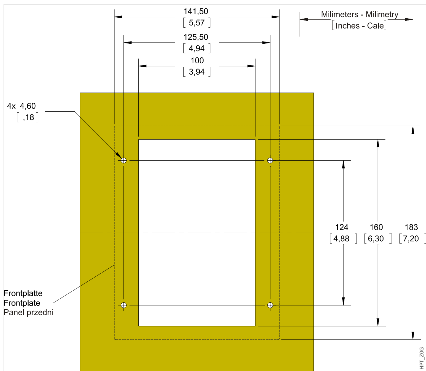
Рис. 6: Вырез дверцы в корпусе B1 (версия с 8 кнопками). (Все размеры указаны в миллиметрах, за исключением размеров в квадратных скобках — [дюймы].)
