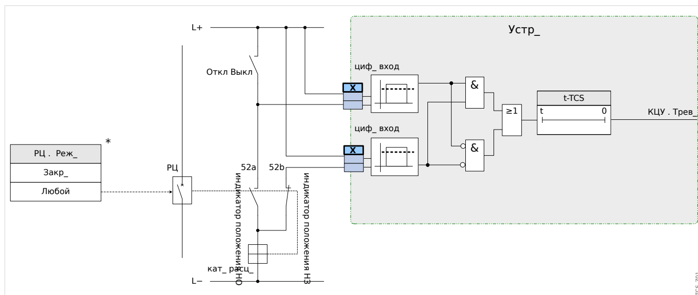
Рис. 58: Пример соединения: контроль цепи отключения с двумя вспомогательными контактами выключателя «Всп Вкл» (52a) и «Всп Выкл» (52b).
