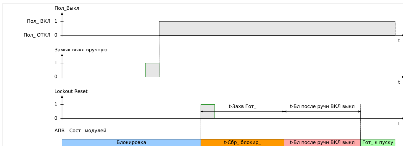
Рис. 55: Логика сброса блокировки АПВ при получении команды сброса блокировки после замыкания выключателя вручную.
