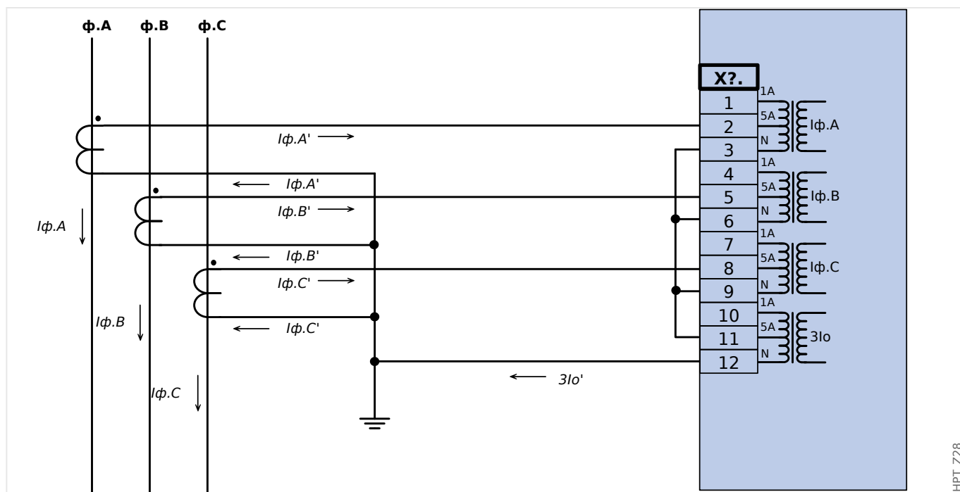
Рис. 21: Измерение фазных токов по схеме «полной» звезды; I_n вторичн. = 5 А. Ток на землю, измеряемый через соединение по схеме Холмгрин 3I_o .ном.втор. = 5 А.
