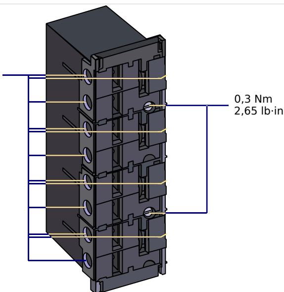
Рис. 79: Штепсельные соединения со встроенными закорачивающими перемычками (стандартные токовые входы)
