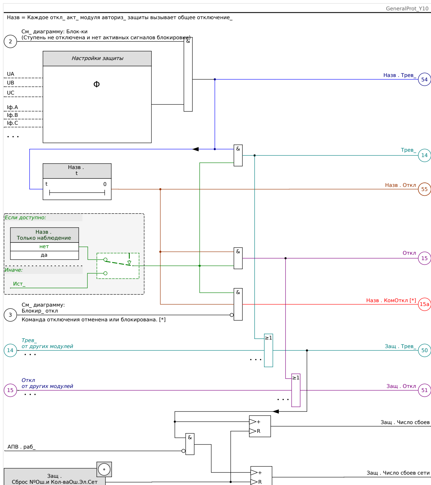
Рис. 43: Примерная схема функций любого элемента защиты HighPROTEC.
