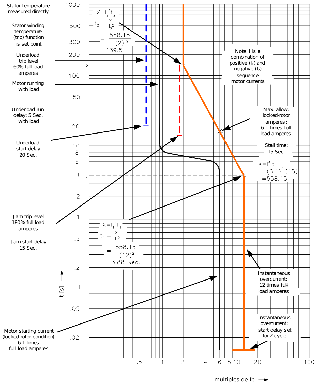
Fig. 69: Courbe de protection du moteur (exemple 3 - avec thermomètres à résistance).
