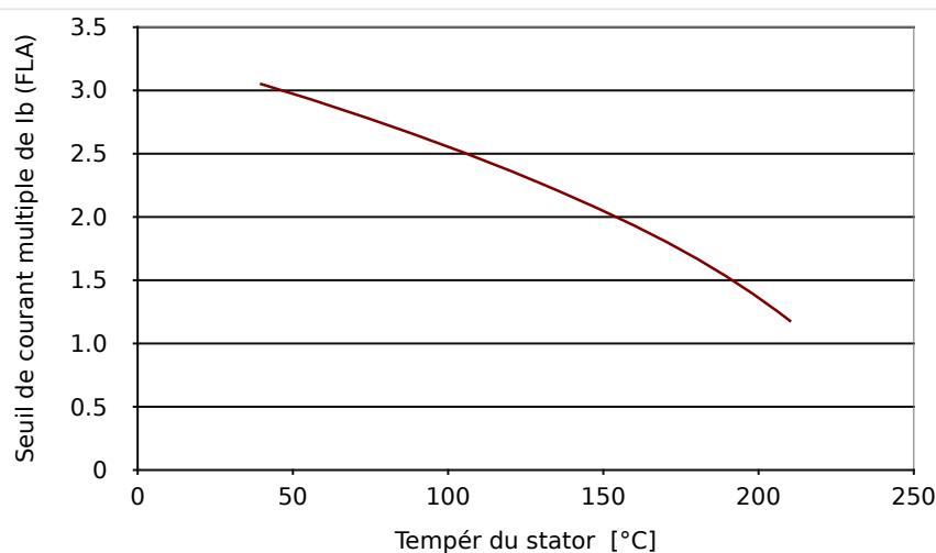
Fig. 64: Seuil de courant efficace / Tempér maxi du stator.
