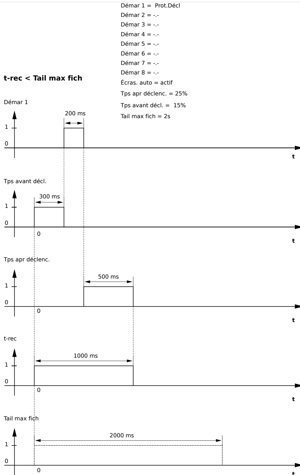
Fig. 100: Exemple de diagramme des temps de l'enregistreur de perturbations II
