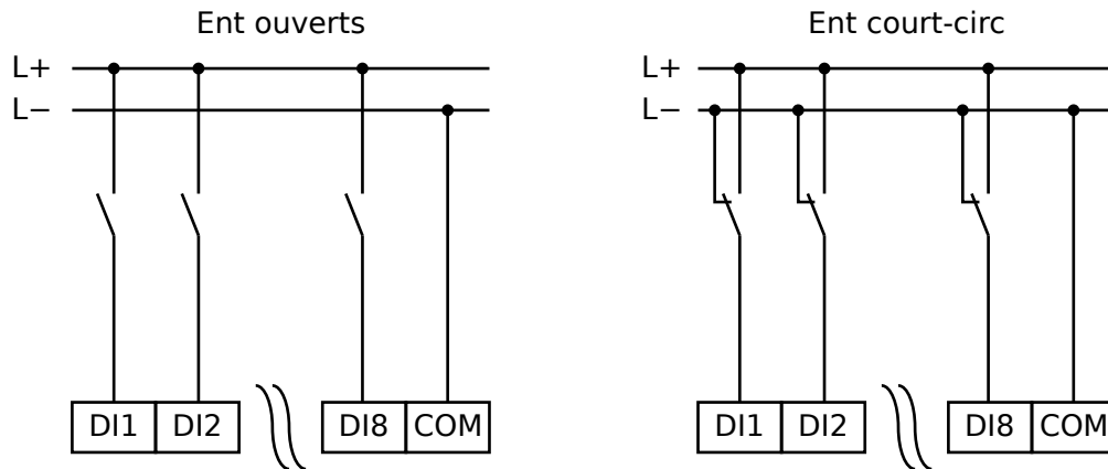
Fig. 111: État sécuritaire des entrées numériques
