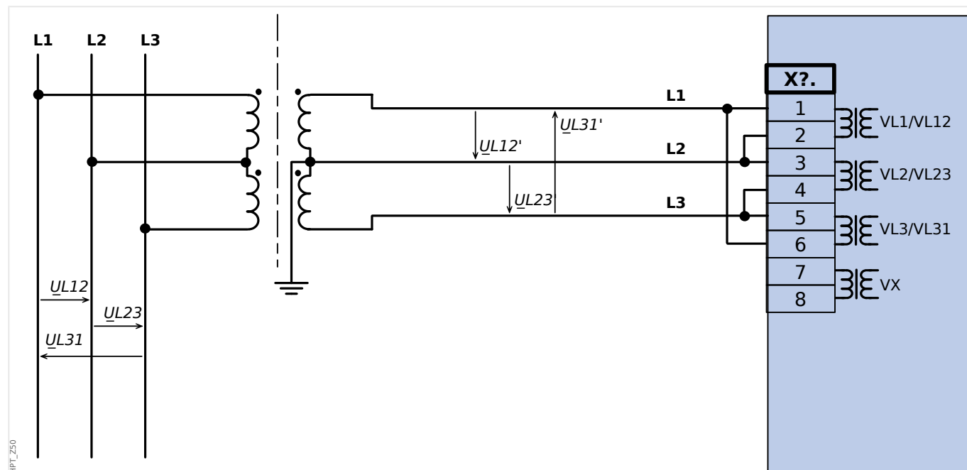
Fig. 32: Mesure de tension biphasée - câblage des entrées de mesure: "Trian ouv"
