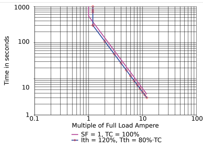
Fig. 65: Limite du modèle Img thermique et courbes de déclenchement sans dét RTD.
