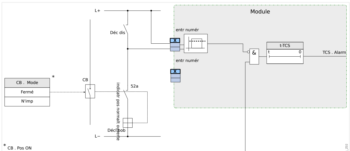
Fig. 88: Exemple de connexion : Surveillance du circuit de déclenchement avec un contact auxiliaire de disjoncteur »Aux ON« (52a).
