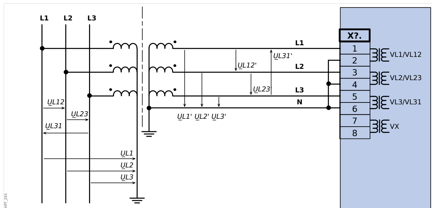
Fig. 28: VT Wye : Mesure de tension triphasée - câblage des entrées de mesure: "connex étoile"
