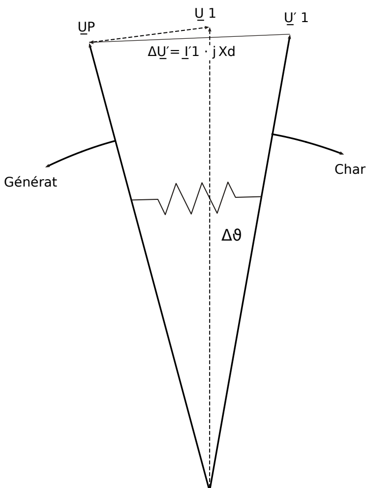
Fig. 81: Vecteurs de tension en cas de coupure de réseau.
