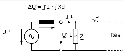
Fig. 80: Circuit équivalent en cas de coupure de réseau.
