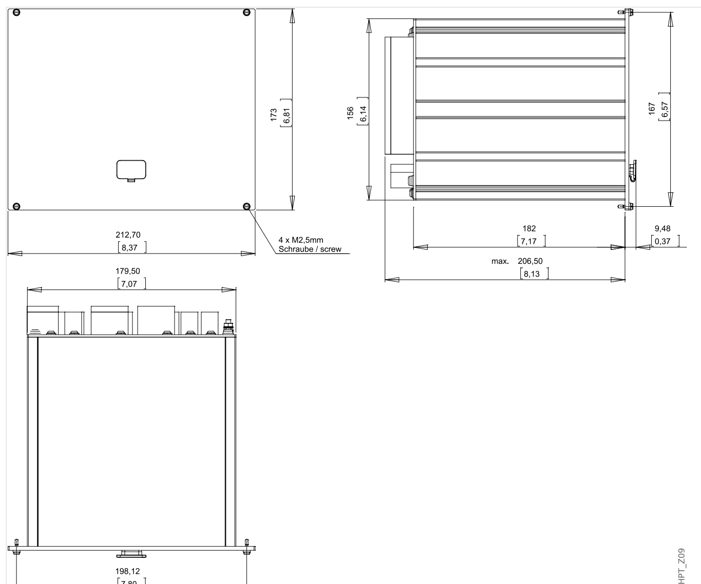
Fig. 4: Vue de trois côtés du boîtier B2 (modules 19 pouces) (Toutes les dimensions sont indiquées en millimètres (mm), à l'exception des dimensions indiquées entre crochets [pouces]).
