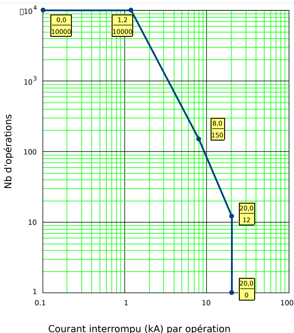
Fig. 96: Courbe de maintenance du disj pour un disj 25 ~kV typique
