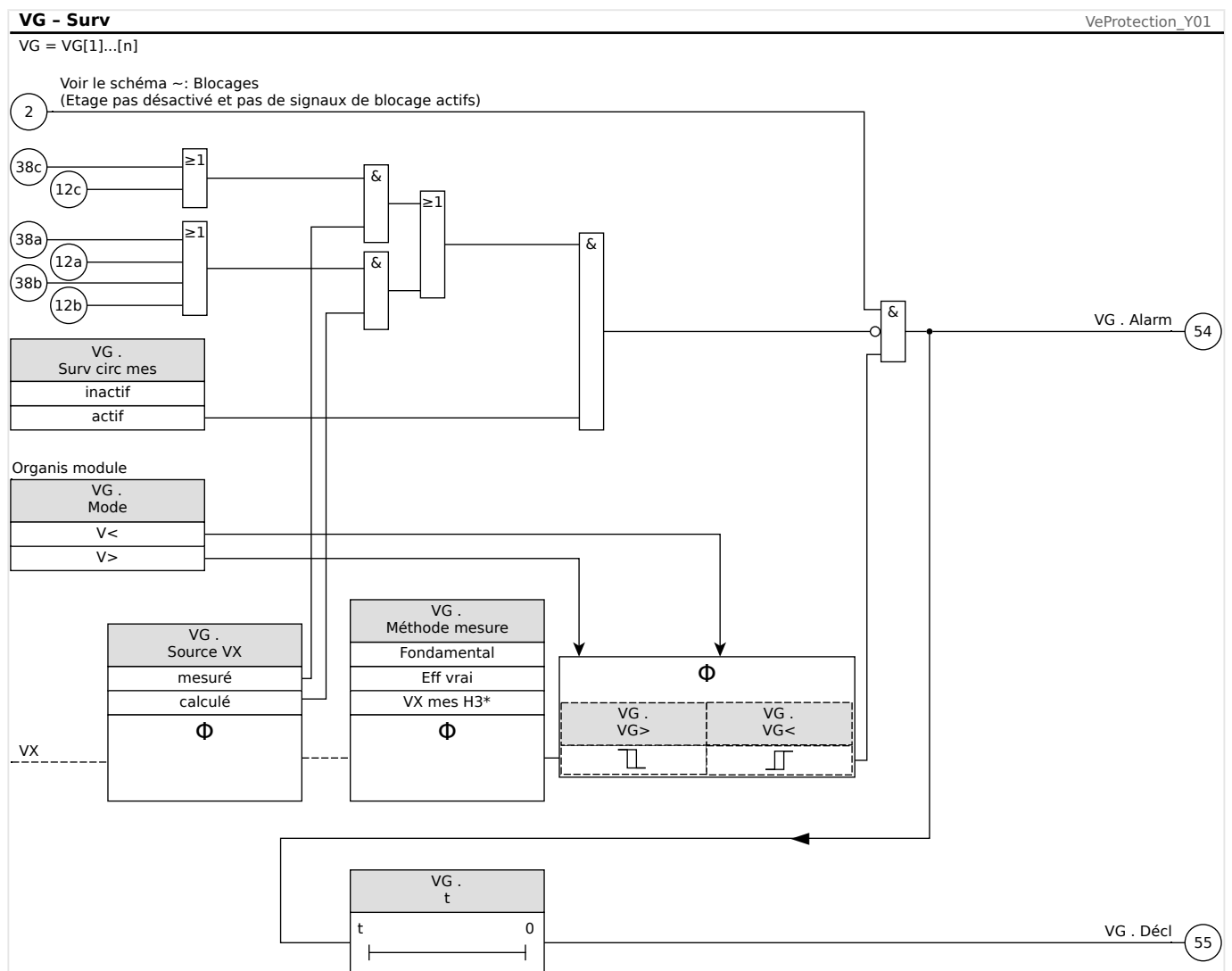
Fig. 76: VG, VX - Surveillance de la tension, partie 1 (fonction de supervision, décision de déclenchement).
