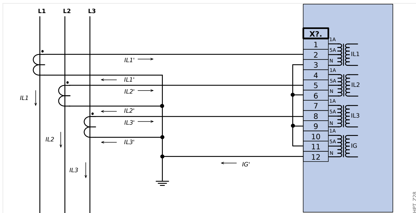
Fig. 21: Mesure de courant triphasé; I_n \text{ sec} = 5 \text{ A} Mesure courant via connexion de Holmgreen; IG_{nom} \text{ sec} = 5 \text{ A}
