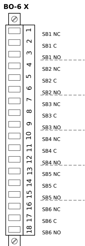
Fig. 13: Affectation électromécanique
