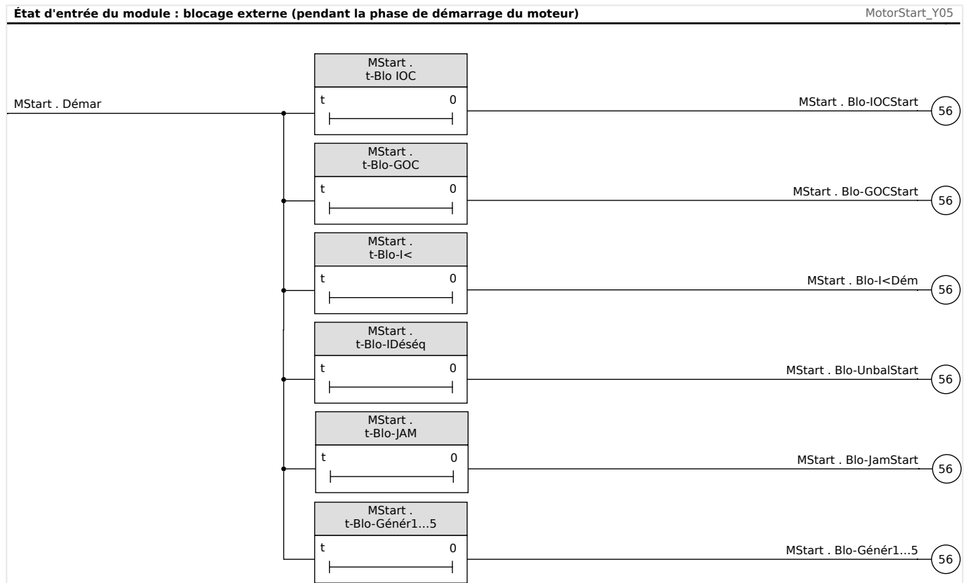
Fig. 60: Blocage temporaire des fonctions de protection du courant lors du démarrage du moteur.
