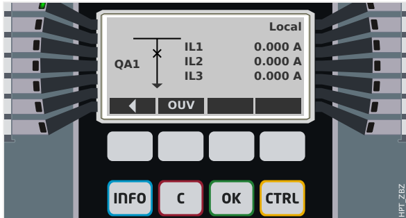
Fig. 91: Exemple de page de contrôle, avec le « disjoncteur » en position fermée.
