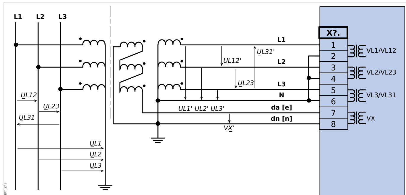
Fig. 29: VT Wye avec une connexion en triangle ouvert.
