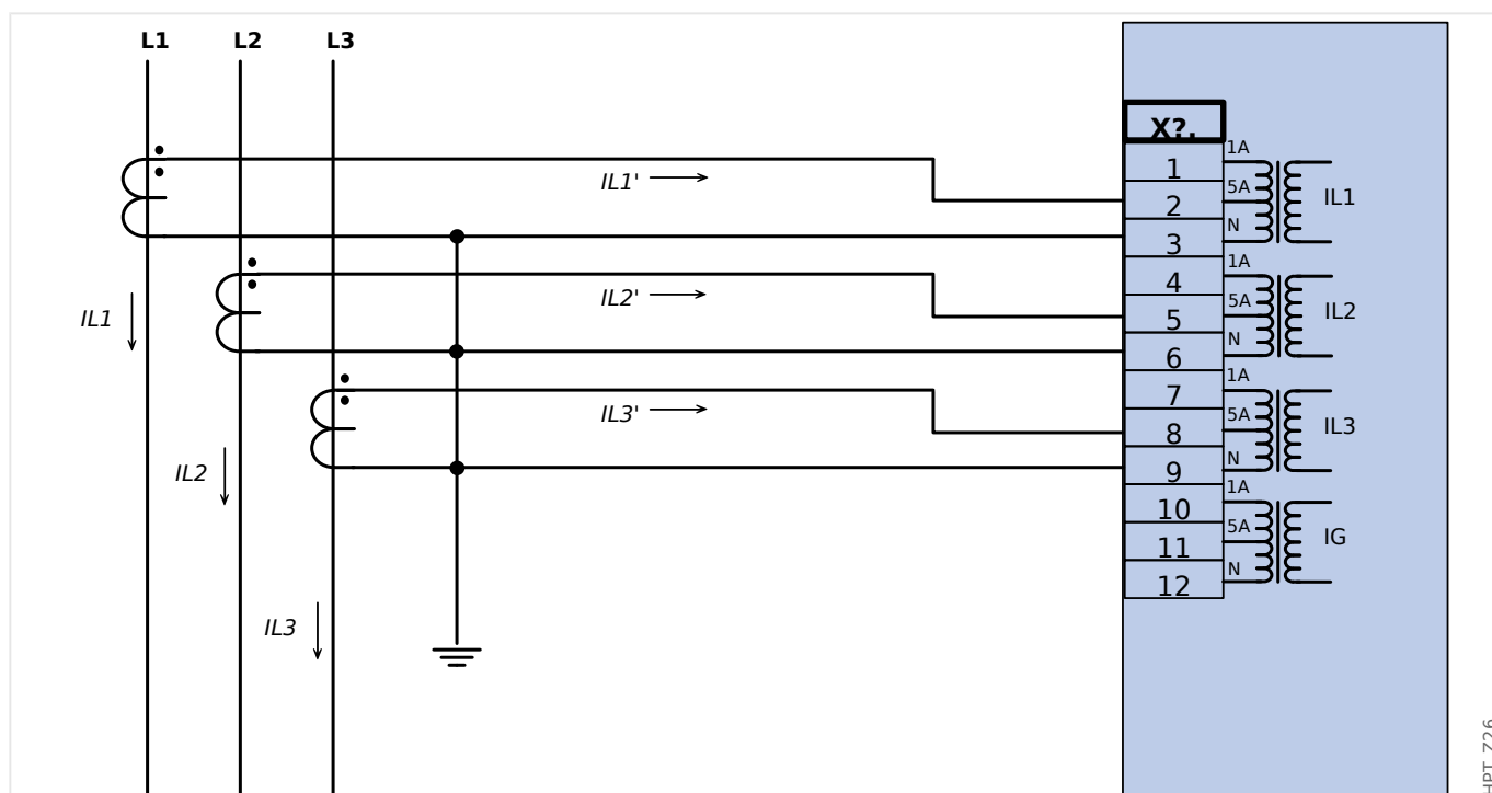
Fig. 19: Mesure de courant triphasé; I_n \text{ sec} = 5 \text{ A}
