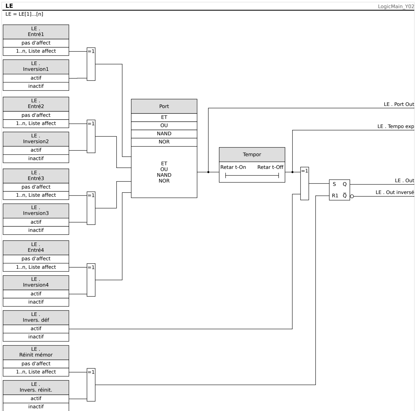
Fig. 103: Présentation détaillée - Diagramme logique global.
