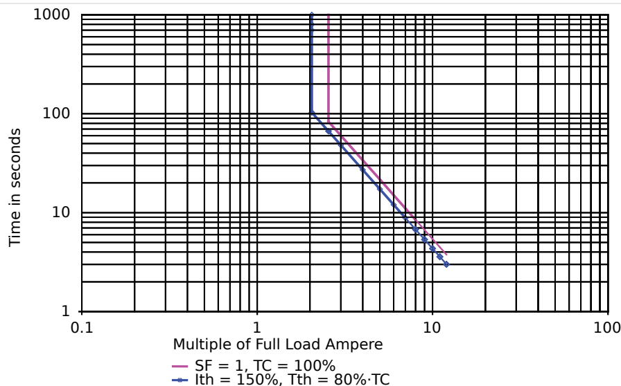
Fig. 66: Limite du modèle img thermique et courbes de déclenchement avec RTD = 100^{\circ}\text{C}
