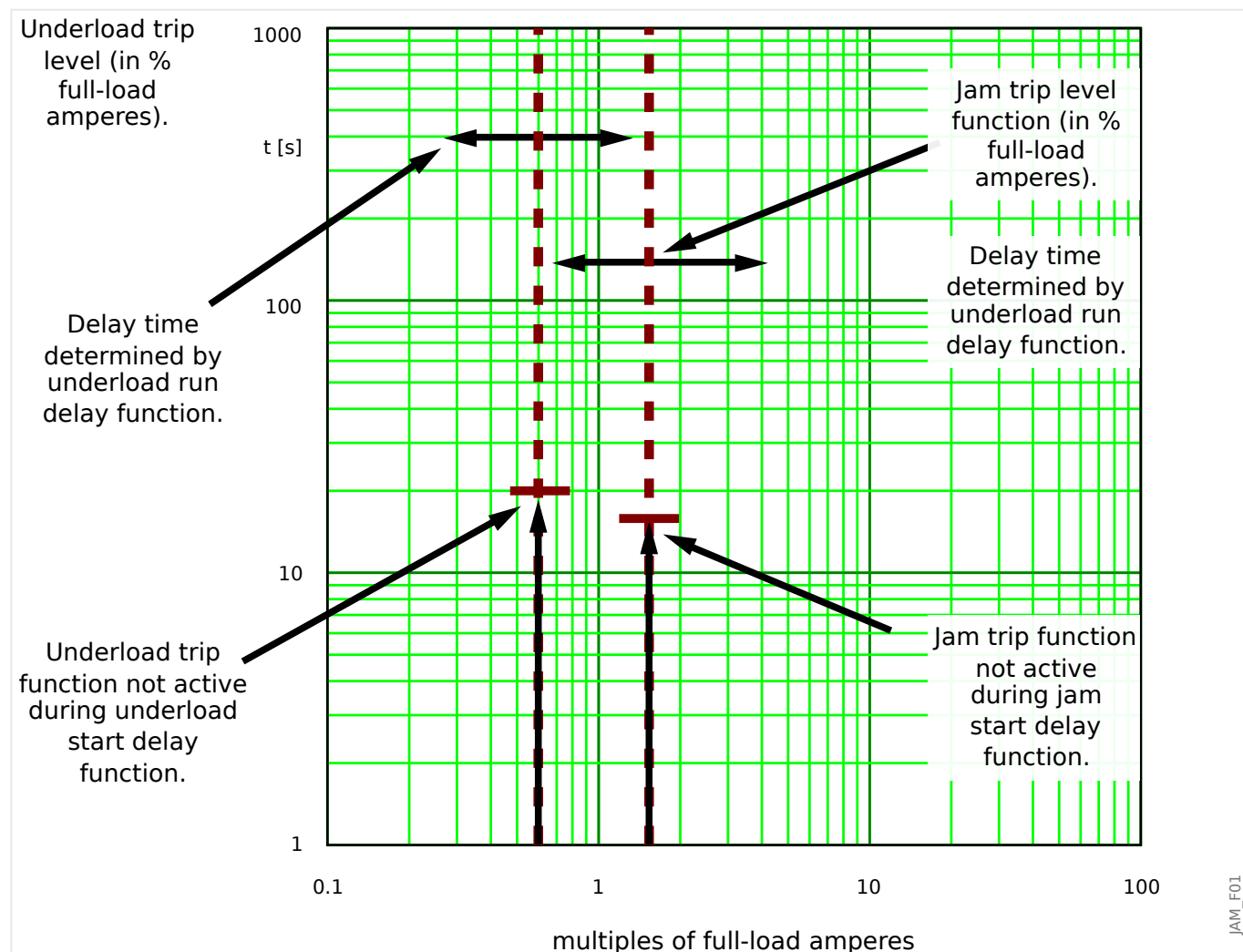
Fig. 70: Fonction de déclenchement de charge insuffisante et JAM.
