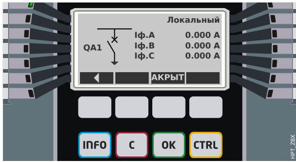
Рис. 93: Пример страницы управления, выключатель в разомкнутом положении.
