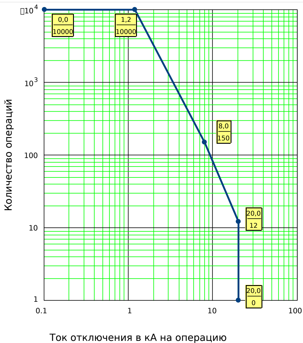
Рис. 96: Эксплуатационная кривая выключателя для типичного выключателя 25кВ
