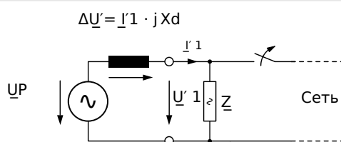
Рис. 80: Эквивалентная цепь при сбое электросети.
