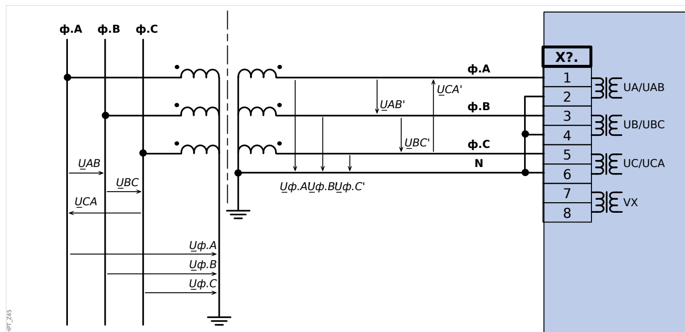
Рис. 28: VT Wye: Измерение трехфазного напряжения по схеме «звезда»
