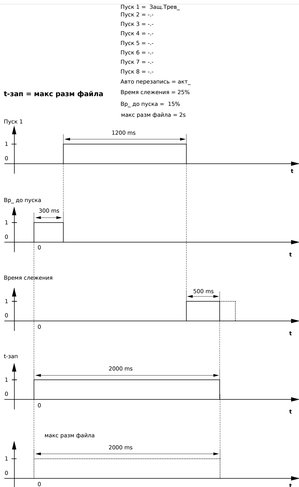
Рис. 99: Пример временной диаграммы регистратора аварийных нарушений I
