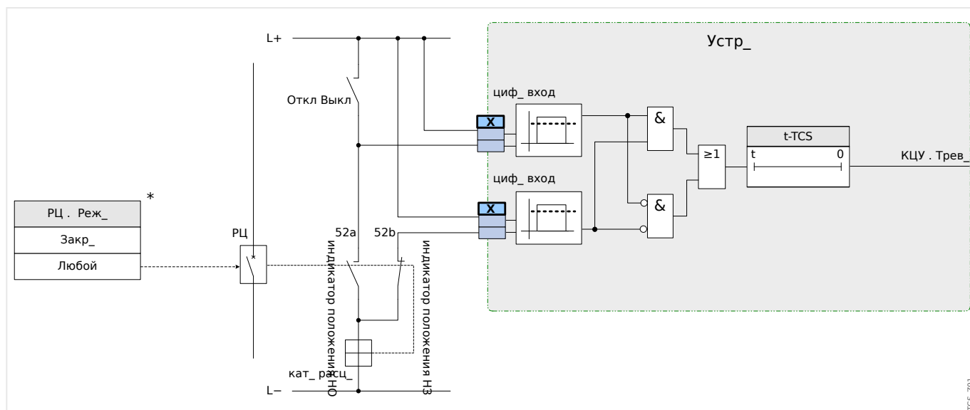
Рис. 87: Пример соединения: контроль цепи отключения с двумя вспомогательными контактами выключателя «Всп Вкл» (52a) и «Всп Выкл» (52b).
