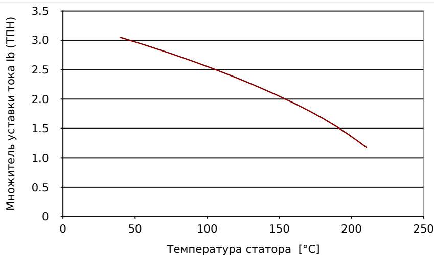
Рис. 64: Эффективная уставка тока по ср. с максимальной температурой статора.
