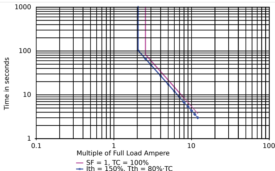
Рис. 66: Кривые ограничений и отключения тепловой модели при ТДС = 100 °С.
