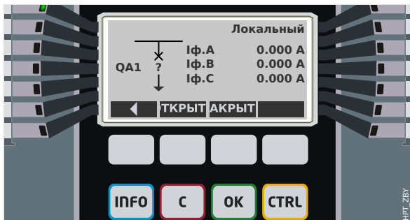
Рис. 92: Пример страницы управления, выключатель в аварийном (недопустимое состояние) положении.
