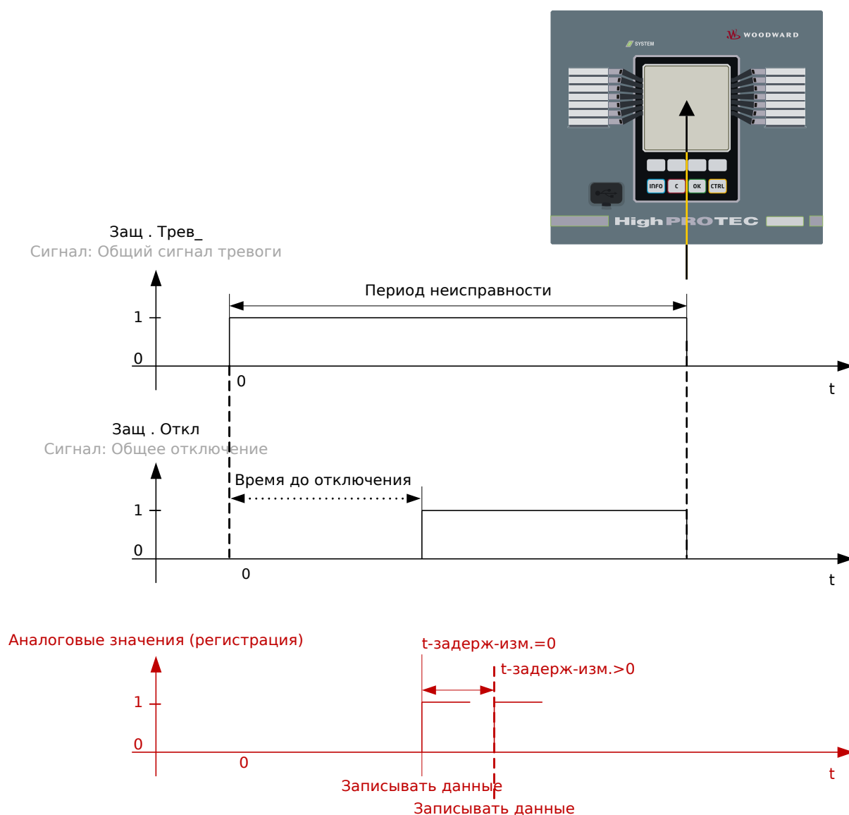
Рис. 101: Регистратор неисправностей: время и длительность.
