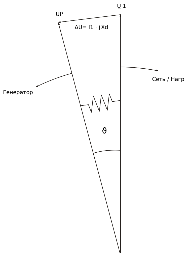
Рис. 79: Векторы напряжения в параллельной работе с электросетью.
