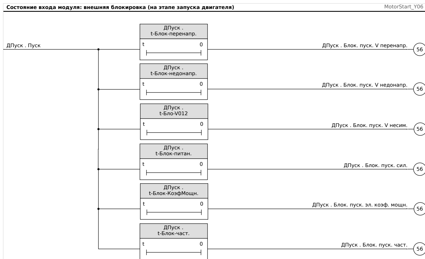
Рис. 61: Временная блокировка функций защиты по напряжению во время запуска двигателя.
