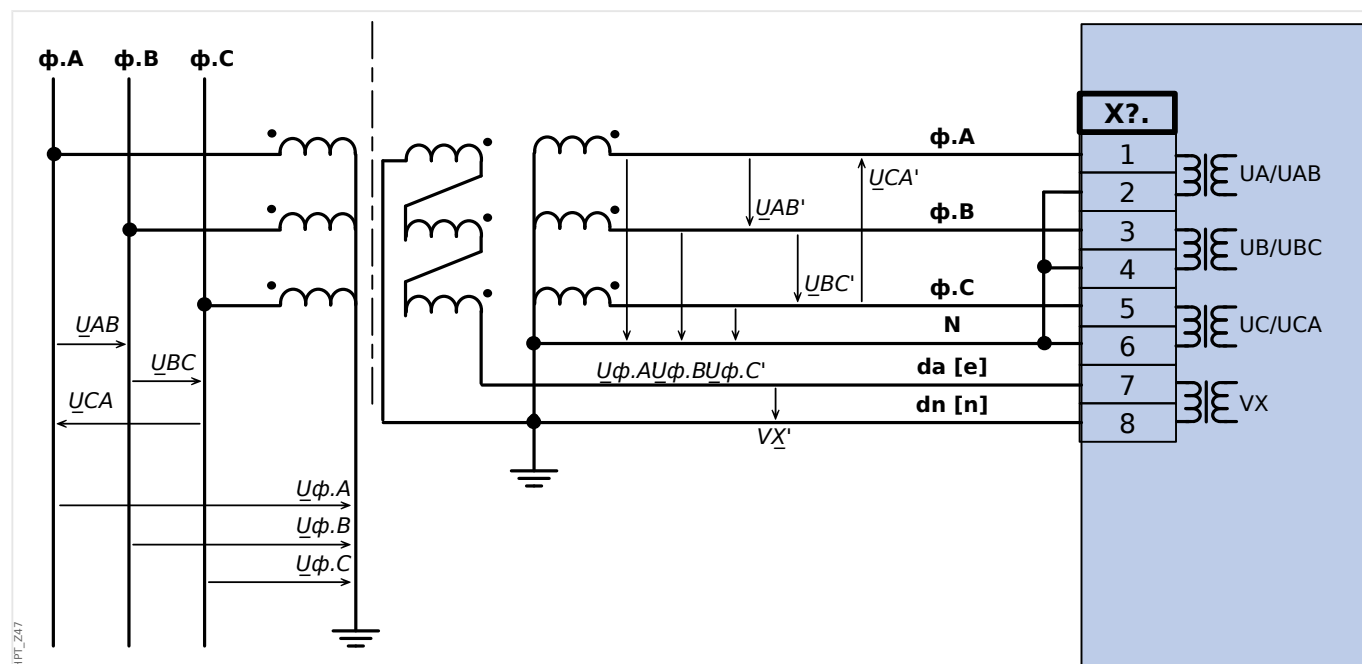
Рис. 29: VT Wye с соединением разомкнутого треугольника.
