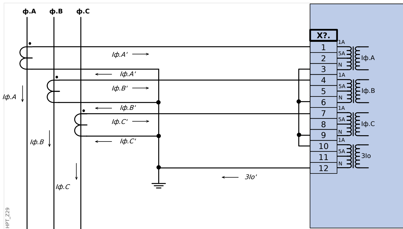
Рис. 22: Измерение фазных токов по схеме «полной» звезды; I_n вторичн. = 1 А. Ток на землю, измеряемый через соединение по схеме Холмгрин 3I_{0'} ном.втор. = 1 А.
