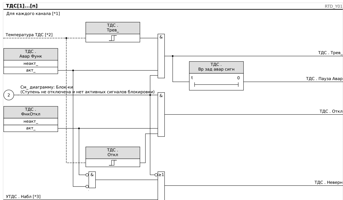
Рис. 86: Общий принцип работы (аварийный сигнал с задержкой, отключение без задержки).
