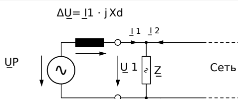
Рис. 78: Эквивалентная цепь синхронного генератора, параллельного электросети.
