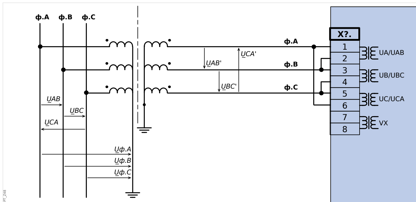
Рис. 30: Измерение трехфазного напряжения - схема измерительных входов: "соединение треугольником"
