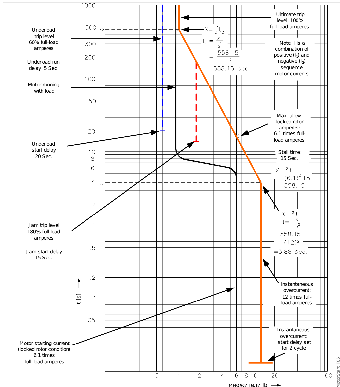
Рис. 68: Кривая защиты двигателя (пример 2 — без ТДС).
