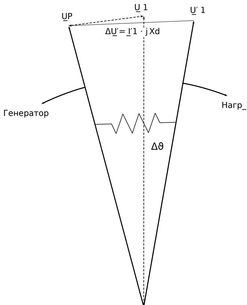
Рис. 81: Векторы напряжения при сбое электросети.
