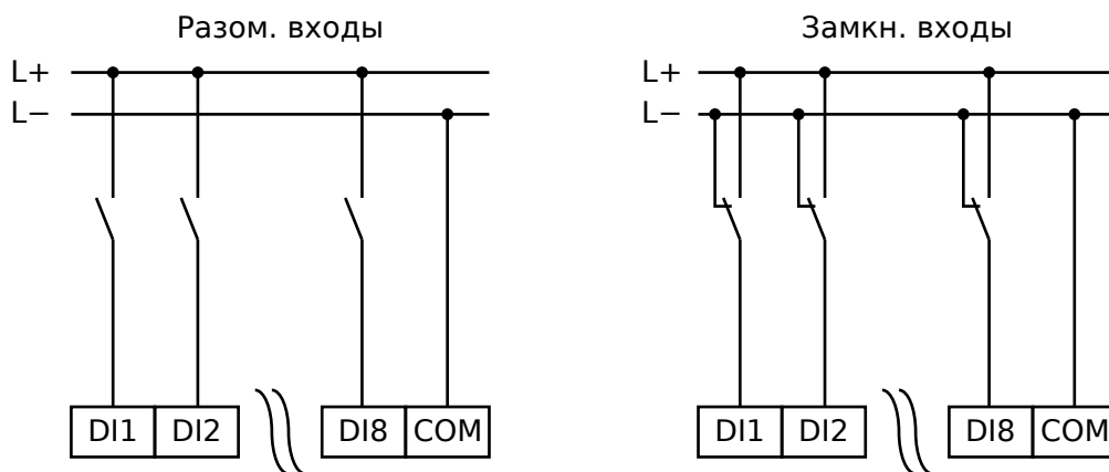
Рис. 111: Безопасное состояние цифровых входов
