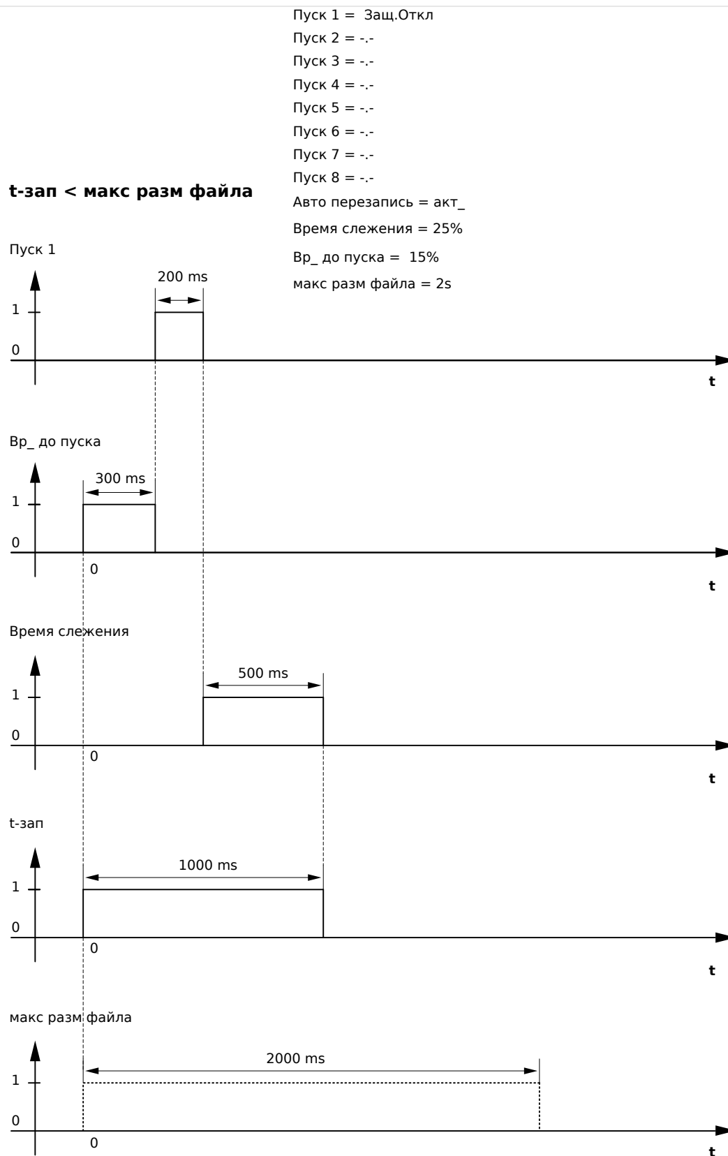
Рис. 100: Пример временной диаграммы регистратора аварийных нарушений II
