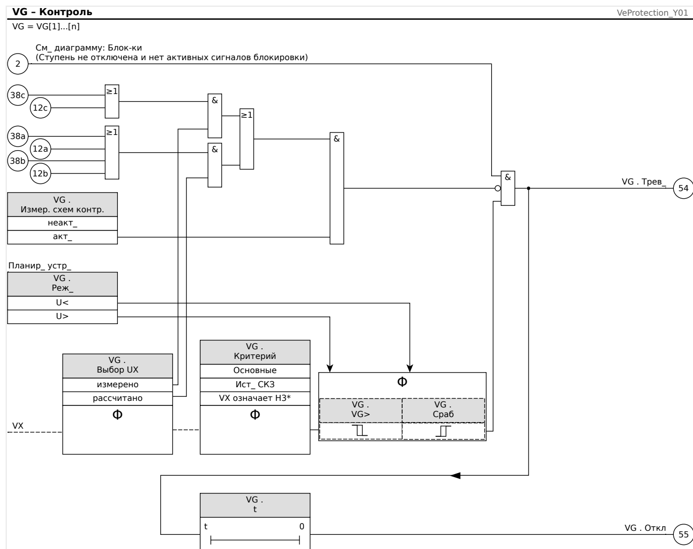
Рис. 44: Контроль напряжения VG, VX, часть 1 (функция контроля, отключение).
