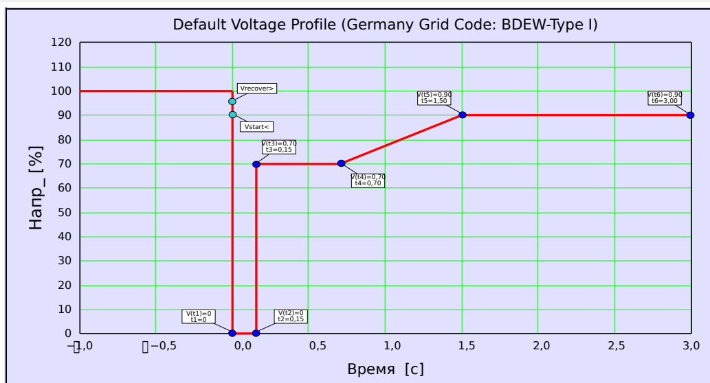
Рис. 59: Профиль LVRT по умолчанию (BDEW, тип I).
