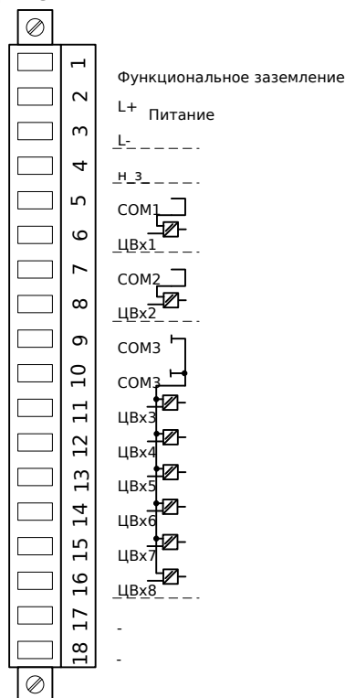
ЦВх-8Р X
