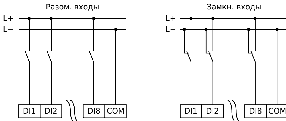
Рис. 81: Безопасное состояние цифровых входов
