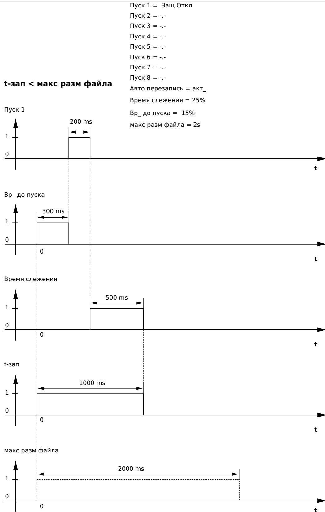
Рис. 71: Пример временной диаграммы регистратора аварийных нарушений II
