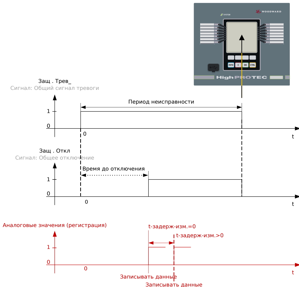
Рис. 72: Регистратор неисправностей: время и длительность.
