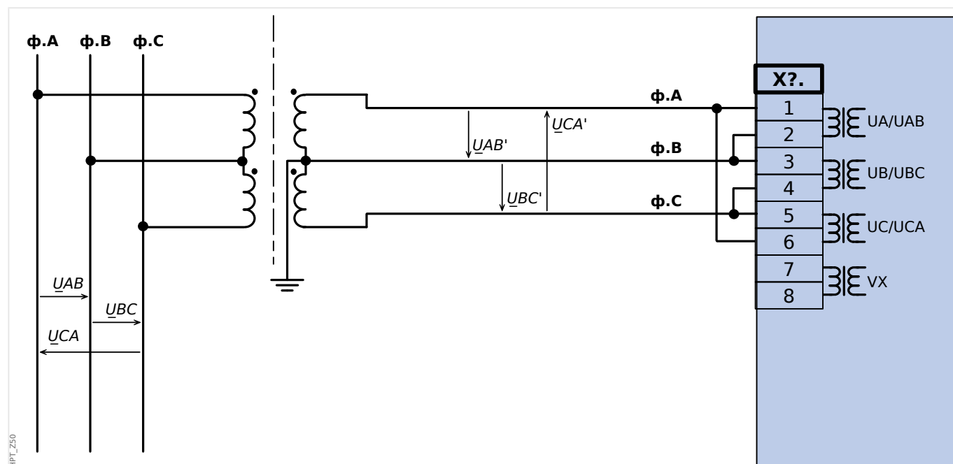
Рис. 21: Измерение двухфазного напряжения - электрическая схема измерительных входов: «соединение открытым треугольником»
