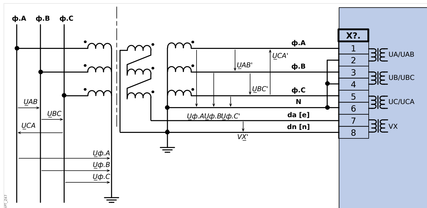
Рис. 18: VT Wye с соединением разомкнутого треугольника.
