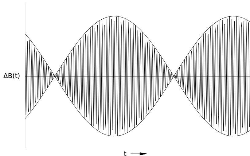
Рис. 52: Кривая напряжения.
