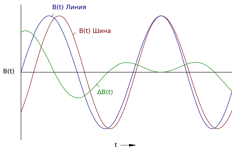
Рис. 53: Кривая напряжения с увеличенным разрешением.
