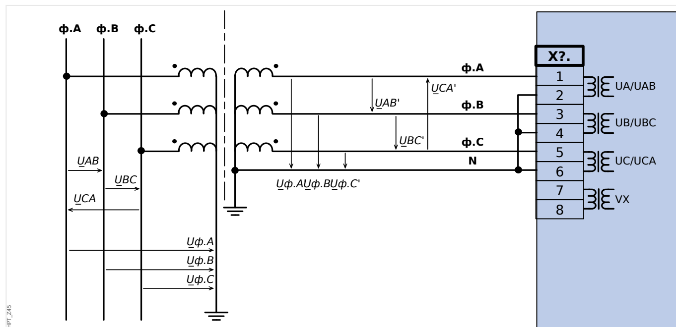
Рис. 17: VT Wye: Измерение трехфазного напряжения по схеме «звезда»
