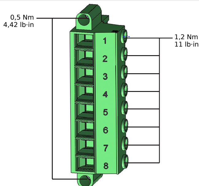
Рис. 80: Измерительные контакты платы измерения напряжения «TU» (→ «2.5.1 TU — измерительные входы напряжения»).
