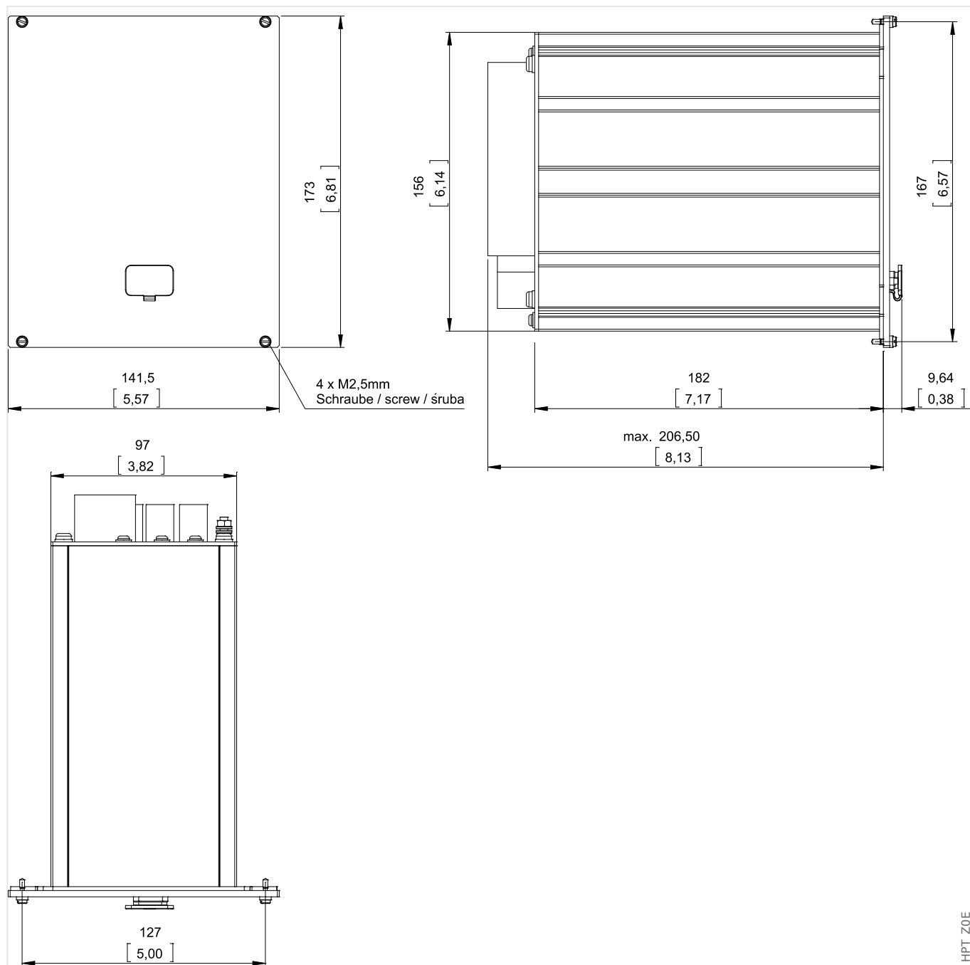
Рис. 4: Корпус В1: внешний вид (19-дюймовые устройства). (Все размеры указаны в миллиметрах, за исключением размеров в квадратных скобках — [дюймы].)
