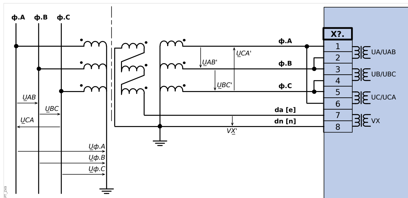
Рис. 20: Измерение трехфазного напряжения - схема измерительных входов: "соединение треугольником" Измерение напряжения нулевой последовательности VG через вспомогательные обмотки (e-n) («открытый треугольник»)
