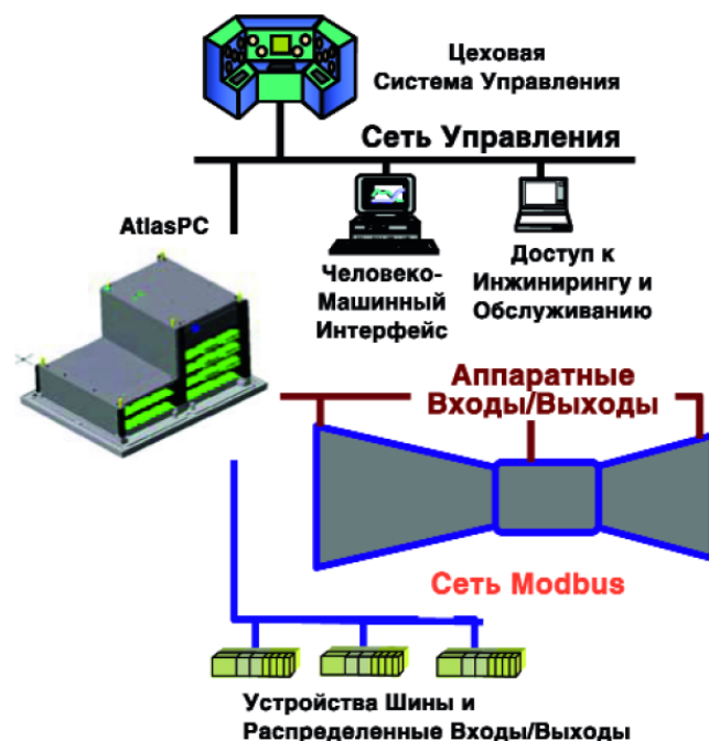
Типовая Конфигурация AtlasSC – Стратегия Сетевого Управления
