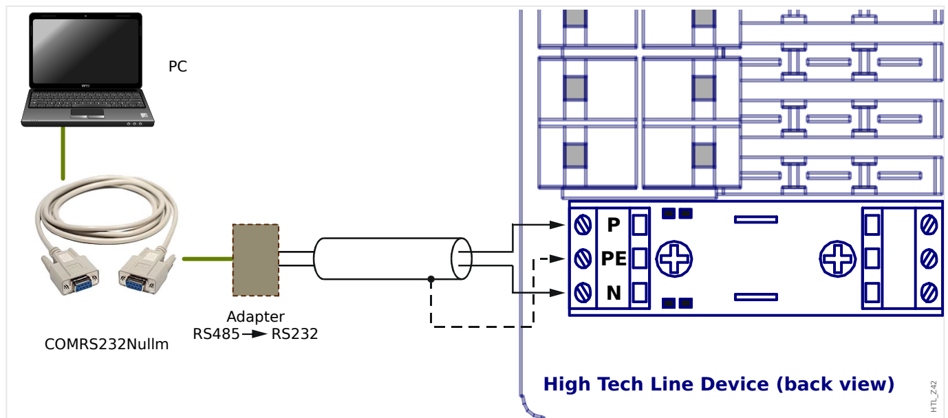
Fig. 3: Conexão de dispositivo de proteção da Linha de alta tecnologia com um PC.
